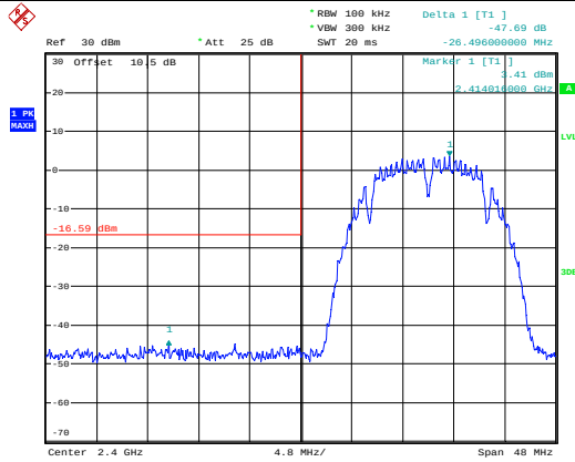
802.11b_Chain 0_Lowest Band edge
