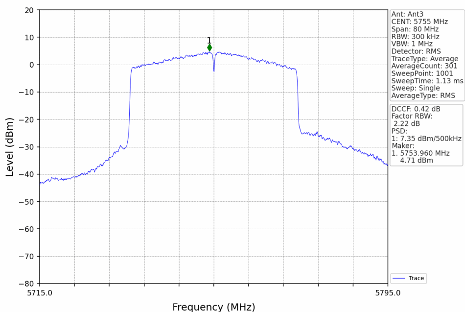
802.11ax(HEW40)_LCH_5755MHz_RU484_Left_Ant3_NTNV
