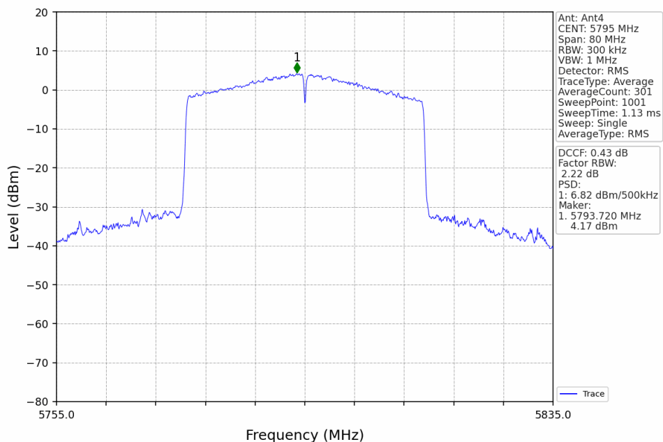
802.11ax(HEW40)_HCH_5795MHz_RU484_Left_Ant4_NTNV
