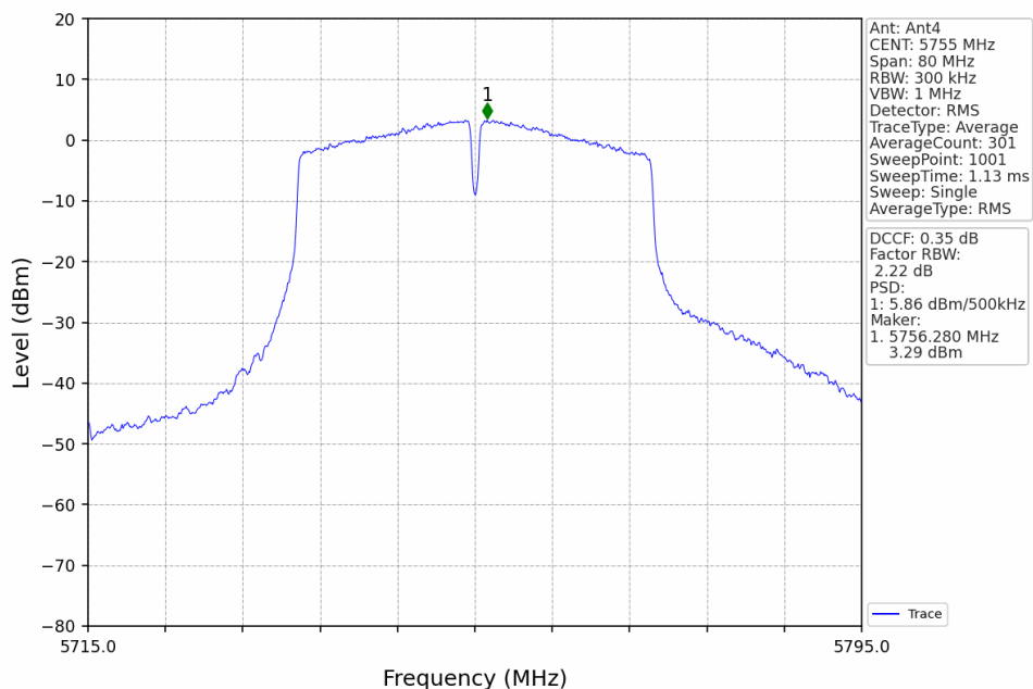
802.11n(HT40)_LCH_5755MHz_Ant4_NTNV
