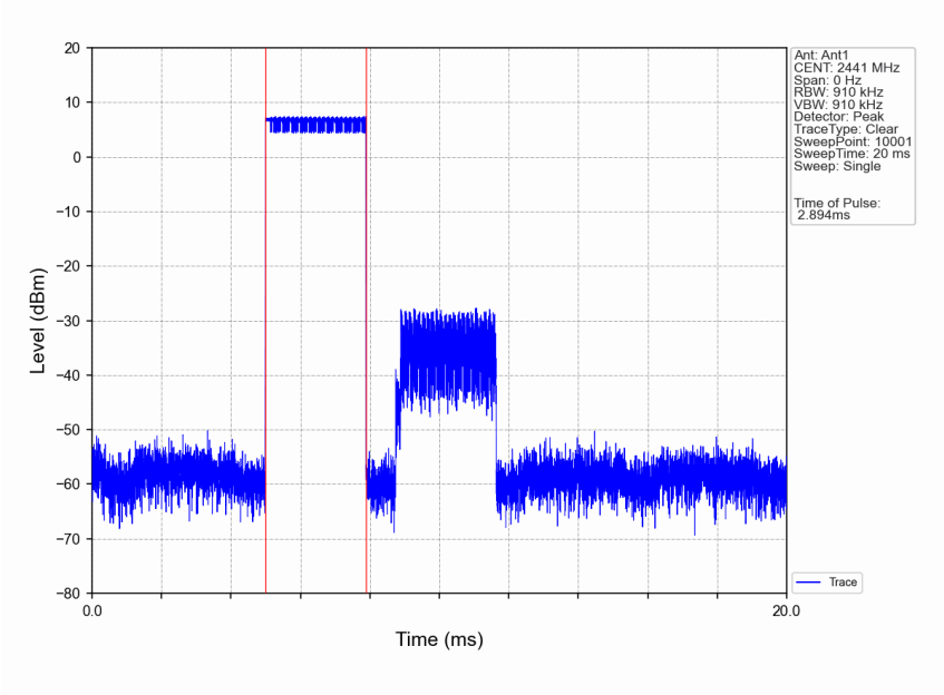
Pi/4DQPSK_2DH5_HOPP_Ant1_NTNV
