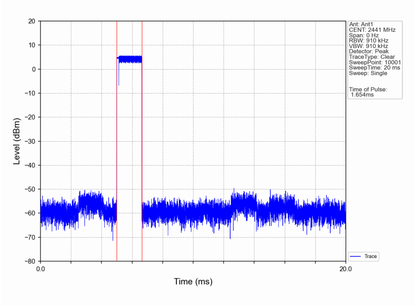
8DPSK_3DH3_HOPP_Ant1_NTNV
