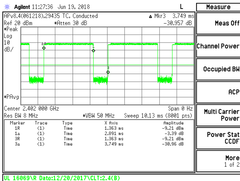
8PSK
