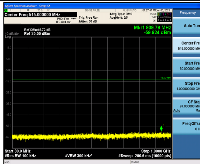
Band2-3MHz-16QAM-18900-1-0-Low-30-1000--59.92-PASS
