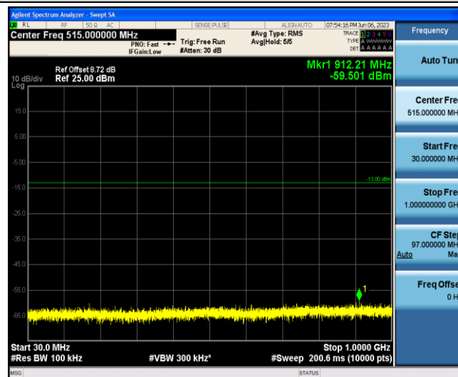
Band2-5MHz-QPSK-18900-1-0-Low-30-1000--59.5-PASS
