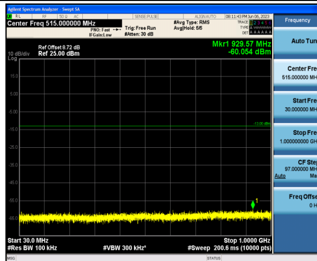
Band2-10MHz-QPSK-18900-1-0-Low-30-1000--60.05-PASS
