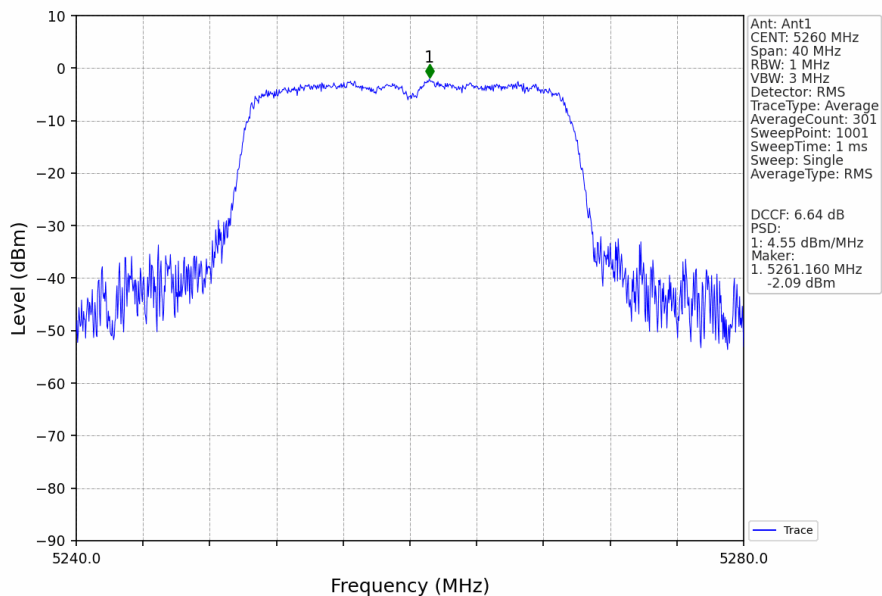
802.11ax(HEW20)_LCH_5260MHz_RU242_Left_Ant1_NTNV
