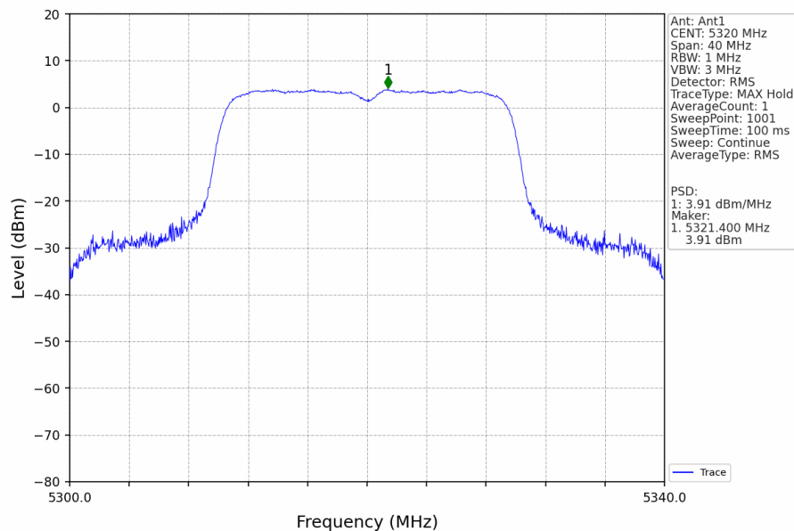
802.11ax(HEW20)_HCH_5320MHz_RU242_Left_Ant1_NTNV
