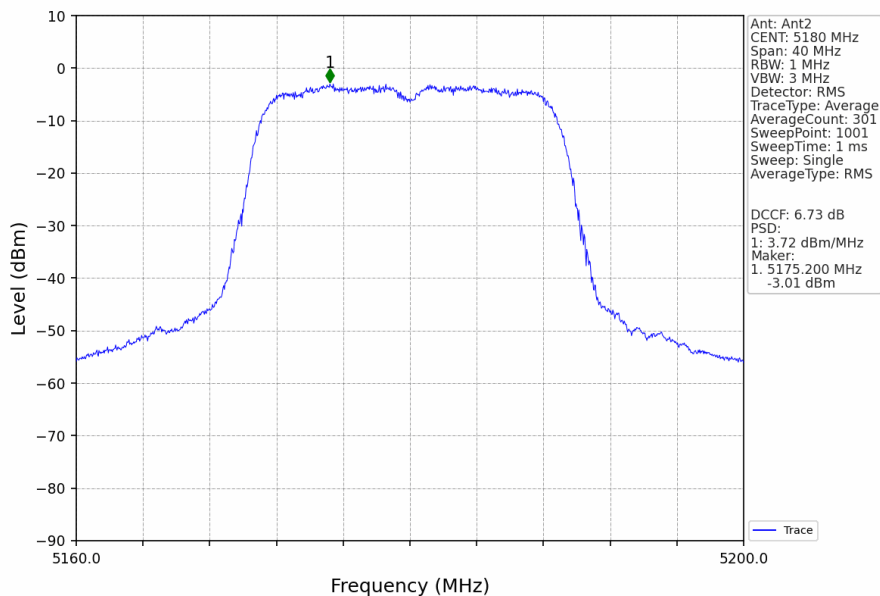
802.11ax(HEW20)_LCH_5180MHz_RU242_Left_Ant2_NTNV
