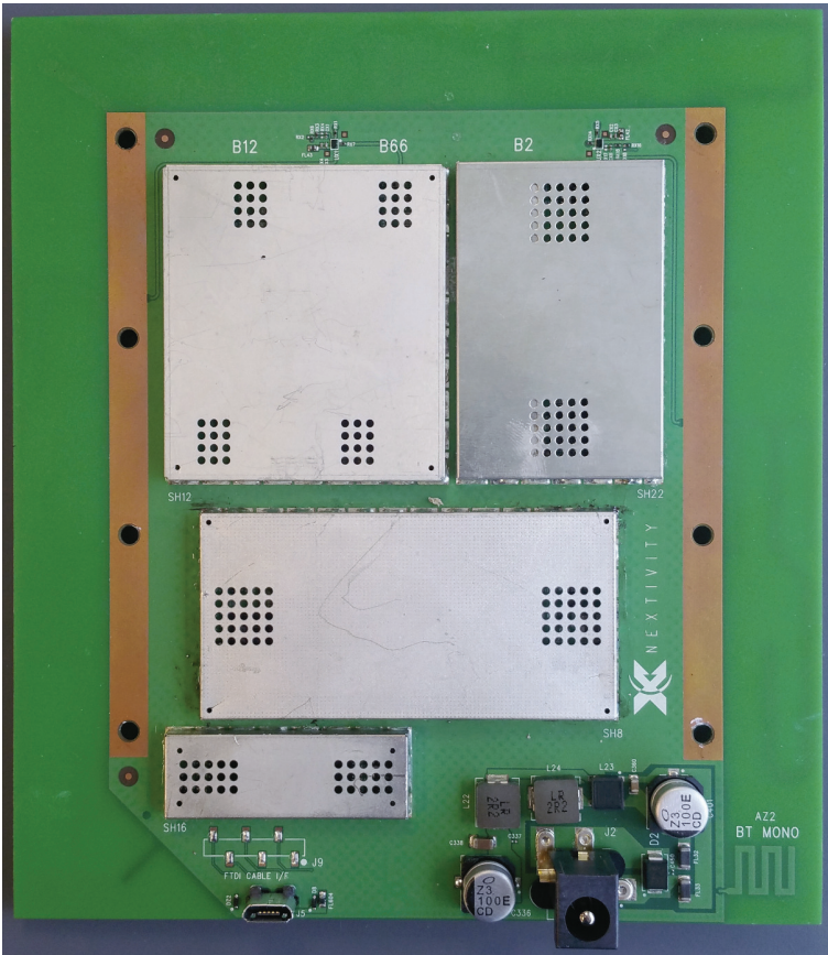
PCB Side_2 - CU
