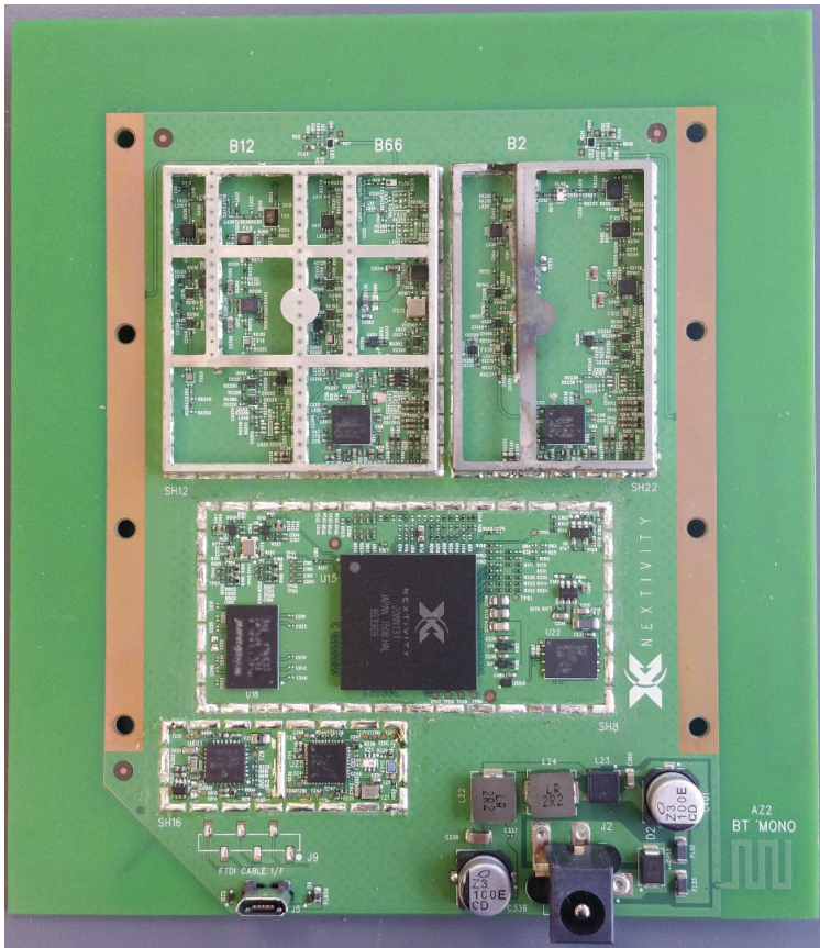
PCB Side_2_no shield - CU
