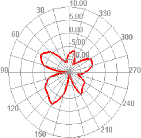
2420.000MHz
