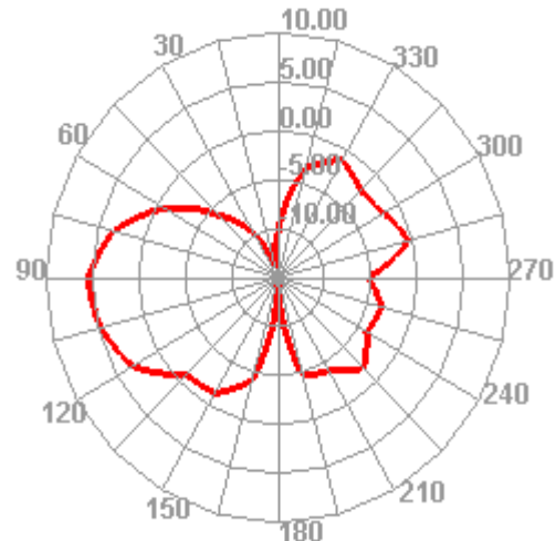
2490.000MHz E2
