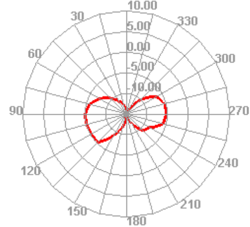
2500.000MHz E1
