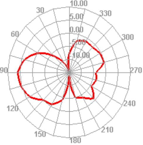
2460.000MHz H
