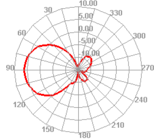
2500.000MHz E2
