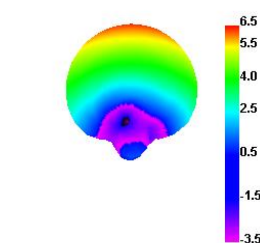
2470.000MHz
