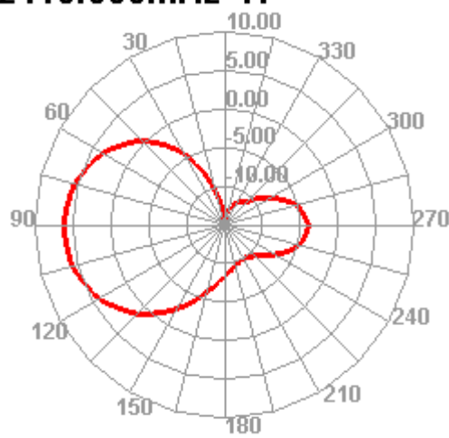
2410.000MHz H
