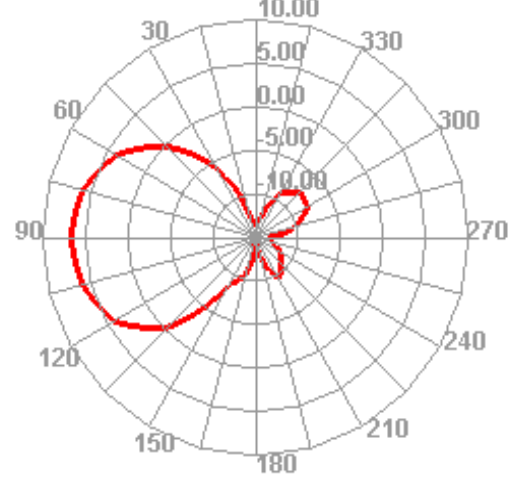
2470.000MHz H
