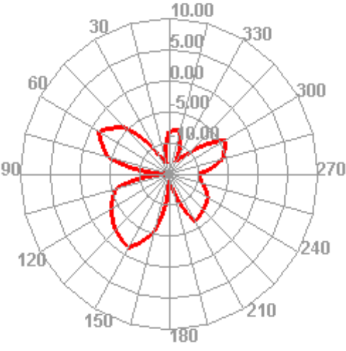
2470.000MHz
