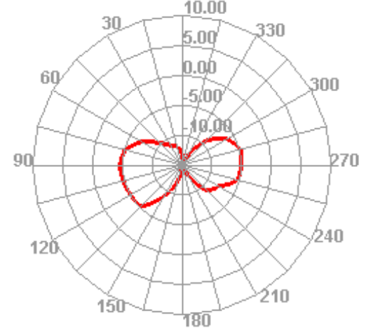
2480.000MHz E1
