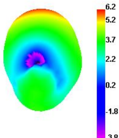
2400.000MHz E1
