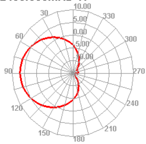
2450.000MHz H
