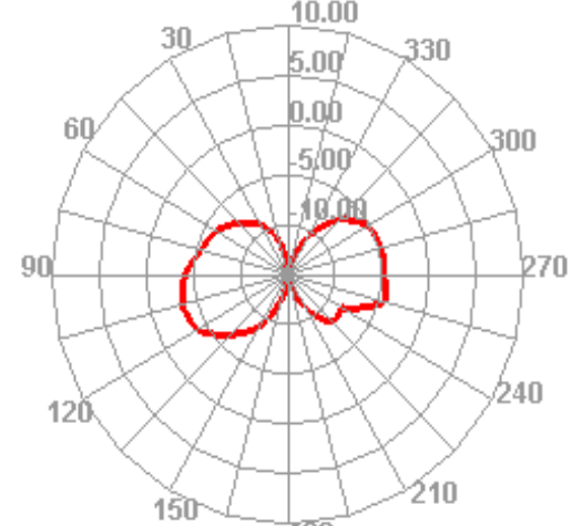
2420.000MHz
