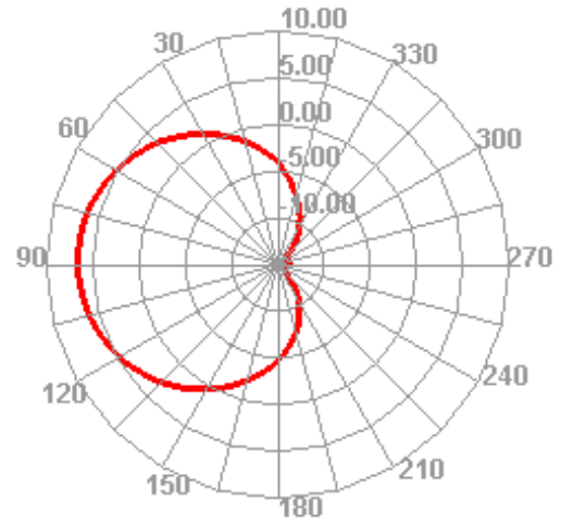
2460.000MHz E2
