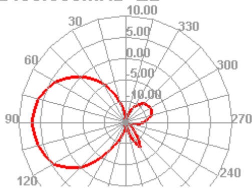
2410.000MHz H
