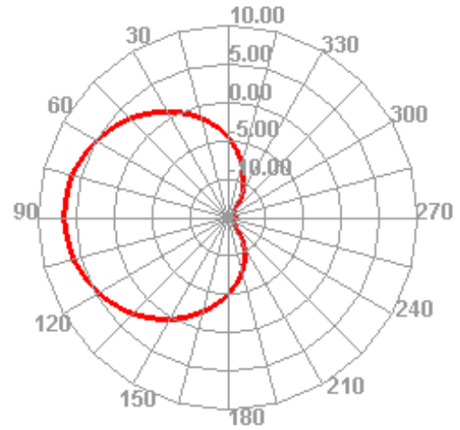
2470.000MHz H
