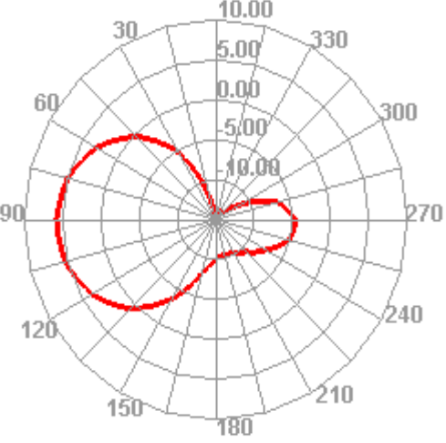
2460.000MHz E2
