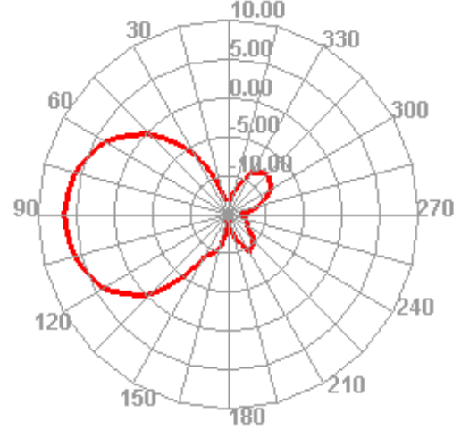
2480.000MHz H
