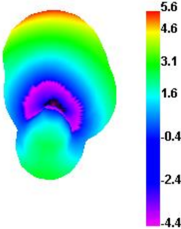
2470.000MHz
