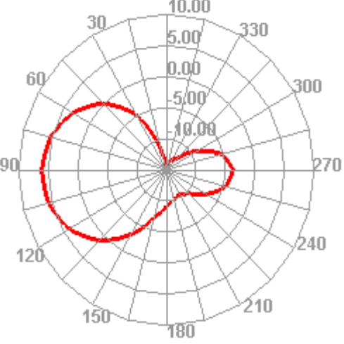
2430.000MHz H
