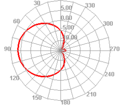
2490.000MHz H
