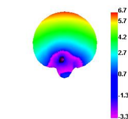
2460.000MHz E1
