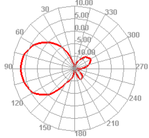
2450.000MHz H
