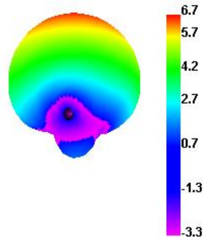
2440.000MHz
