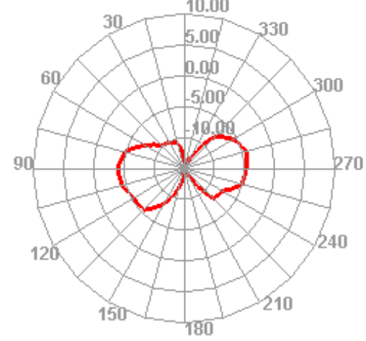
2470.000MHz
