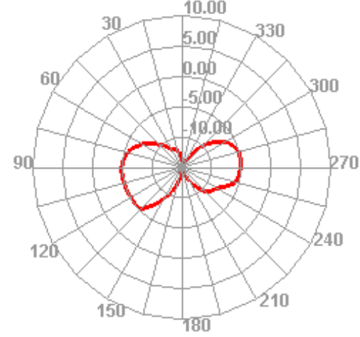
2490.000MHz E1
