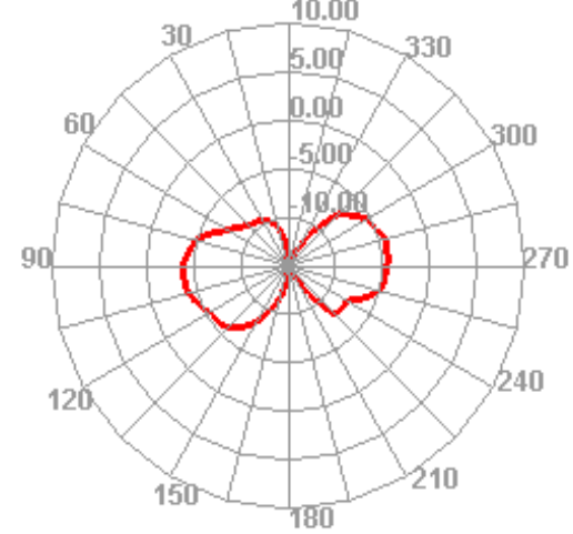
2460.000MHz
