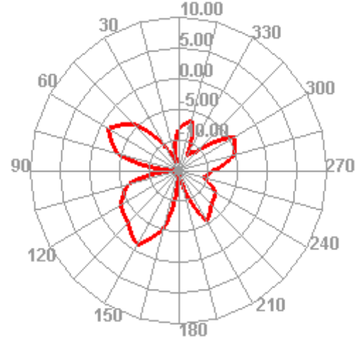
2440.000MHz
