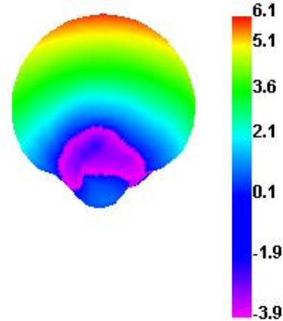
2500.000MHz
