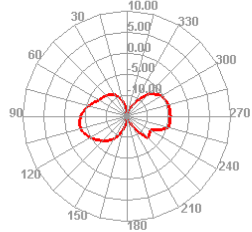
2440.000MHz
