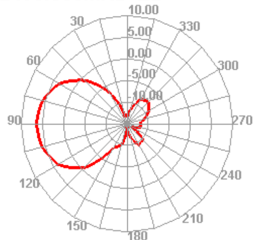
2490.000MHz E2
