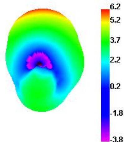
2410.000MHz
