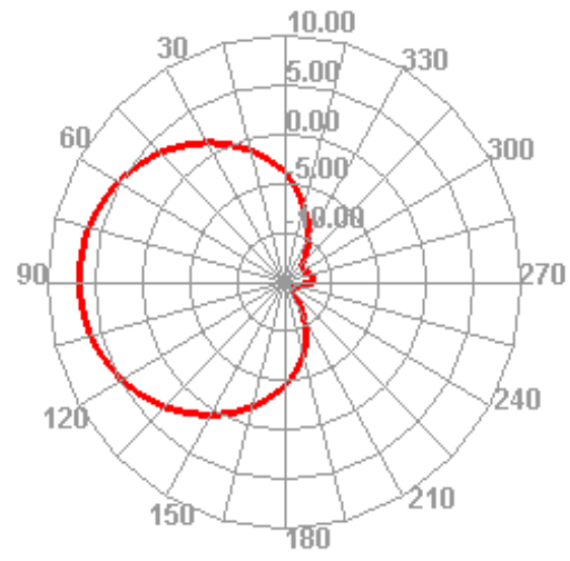
2440.000MHz H
