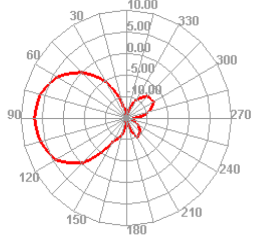
2460.000MHz H
