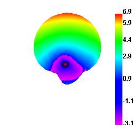
2420.000MHz E1
