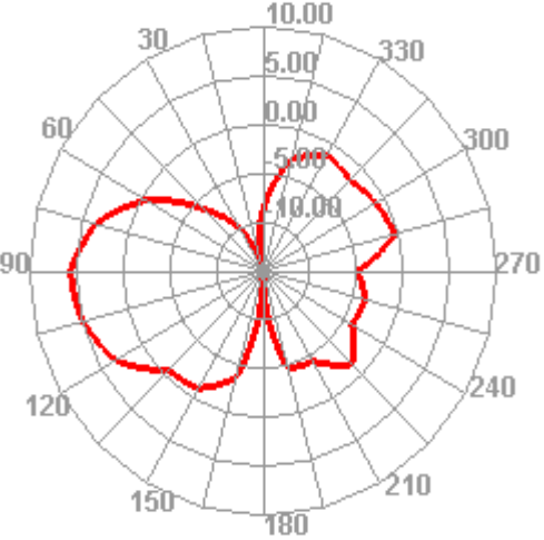
2480.000MHz H
