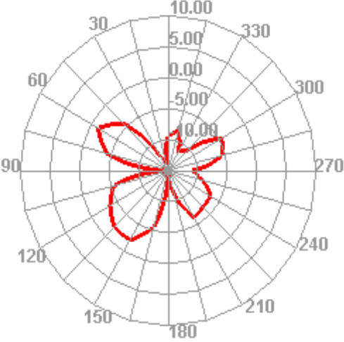
2480.000MHz E1
