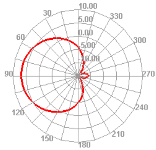
2420.000MHz E2
