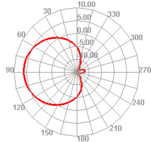
2500.000MHz H
