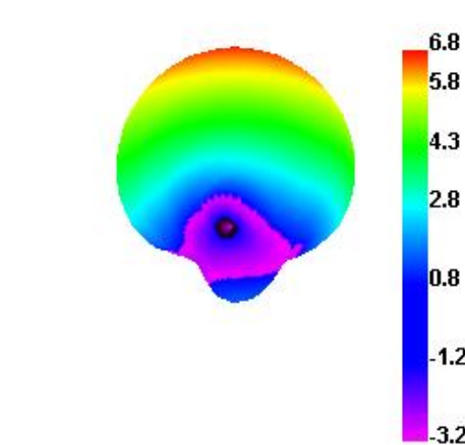
2430.000MHz
