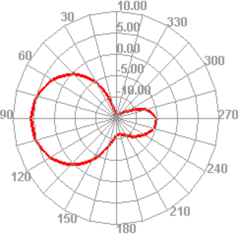
2480.000MHz E2
