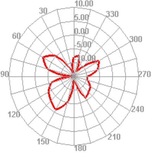
2460.000MHz
