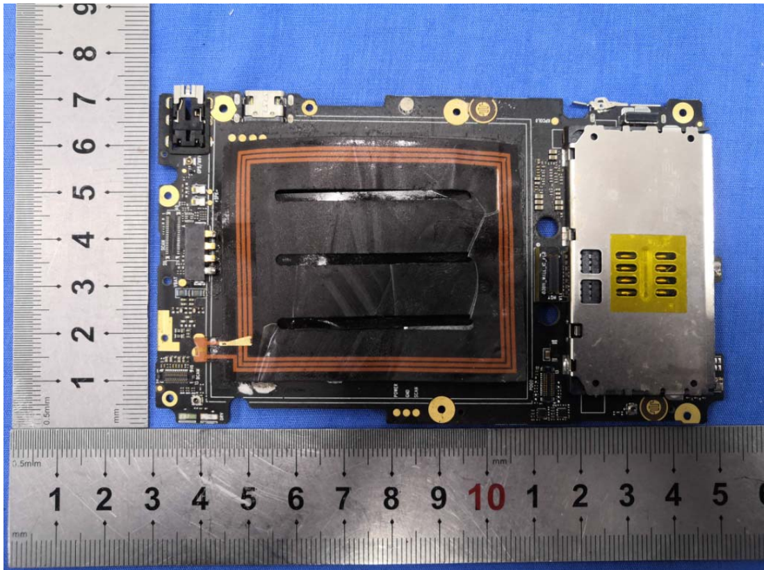
NFC Antenna
