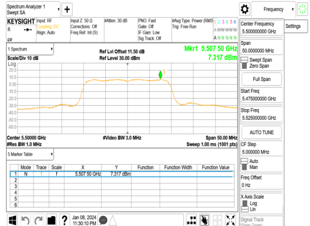
802.11ax_20MHz_Chain0_5500MHz_RU106_53
