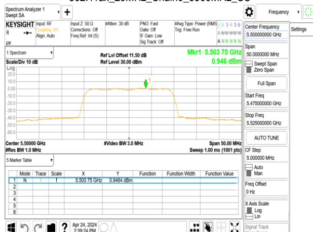
802.11ax_20MHz_Chain0_5500MHz_SU
