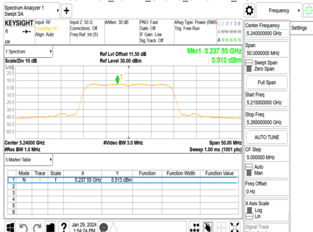
802.11ax_20MHz_Chain0_5240MHz_RU
