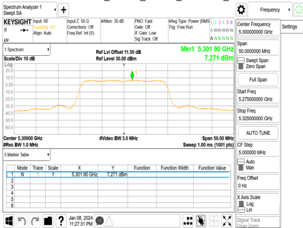
802.11ax_20MHz_Chain0_5300MHz_SU
