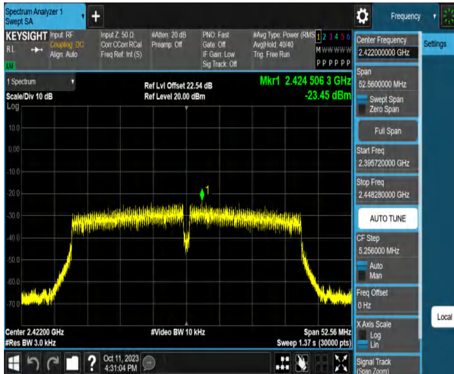
11N40MIMO_Ant2_2422
