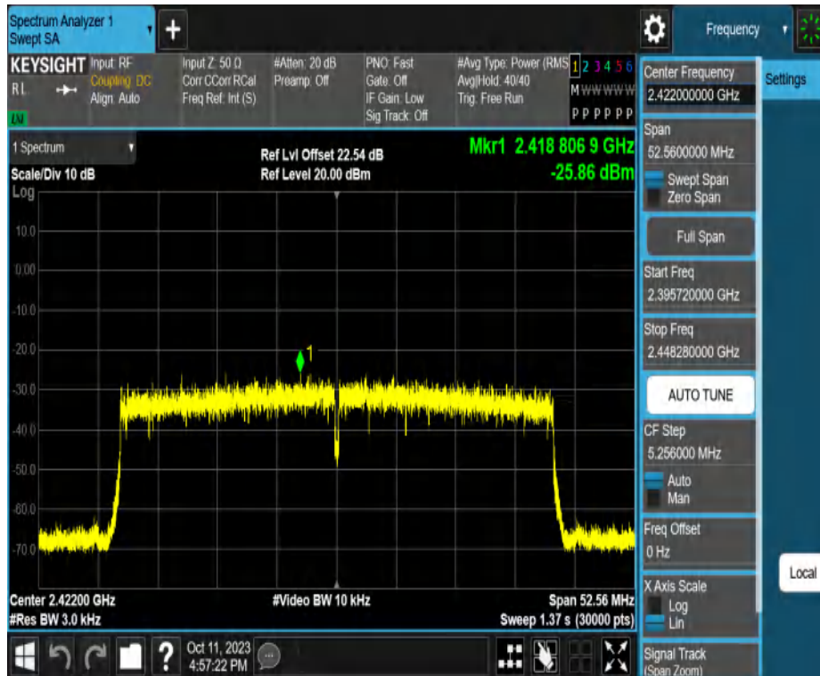
11AX40MIMO_Ant2_2422
