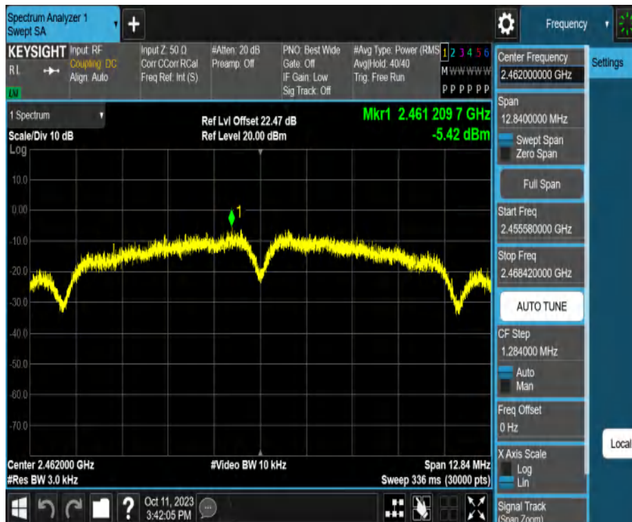
11B-CDD_Ant2_2462
