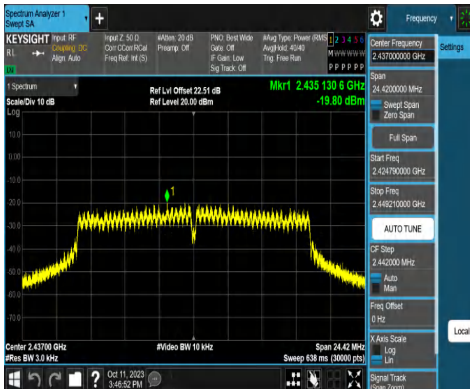
11G-CDD_Ant2_2437
