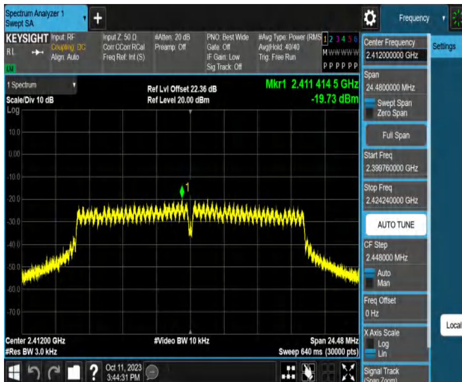
11G-CDD_Ant2_2412
