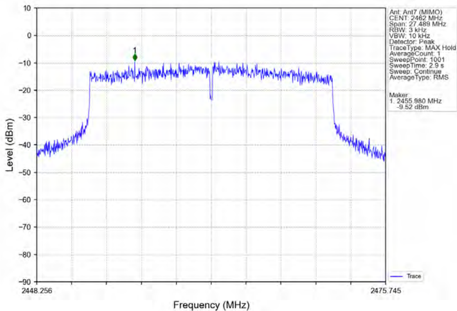
802.11ax(HEW20)_HCH_2462MHz_RU242_Left_Ant7 (MIMO)_NTNV
