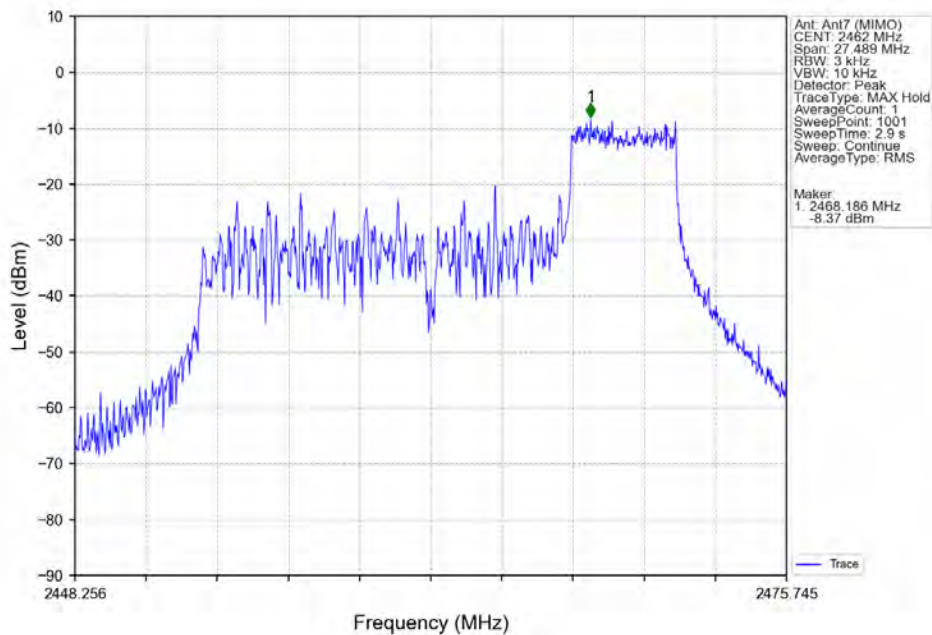
802.11ax(HEW20)_HCH_2462MHz_RU52_Right_Ant7 (MIMO)_NTNV
