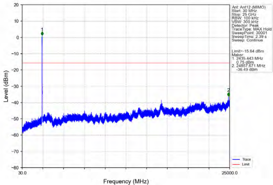
802.11n(HT40)_LCH_2422MHz_Ant12 (MIMO)_NTNV
