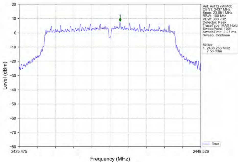
802.11g_MCH_2437MHz_Ant12 (MIMO)_NTNV
