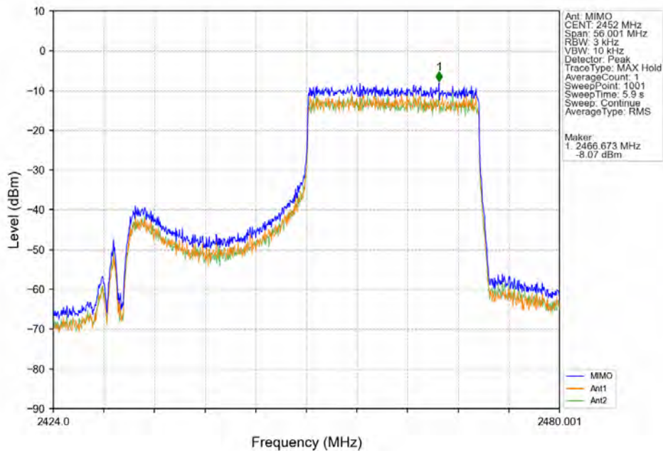
802.11ax(HEW40)_HCH_2452MHz_RU484_Left_Ant7 (MIMO)_NTNV
