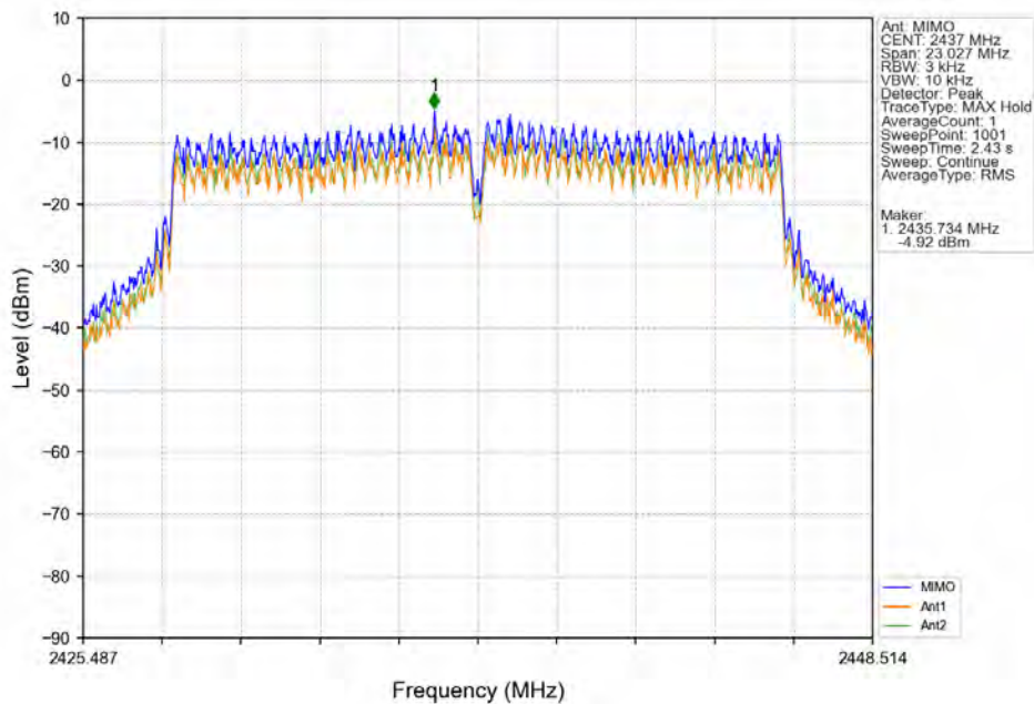
802.11ac(VHT20)_MCH_2437MHz_MIMO_NTNV
