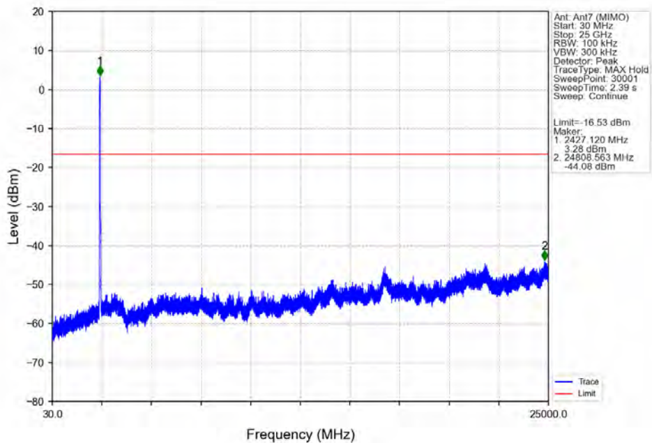
802.11ax(HEW40)_LCH_2422MHz_RU484_Left_Ant7 (MIMO)_NTNV
