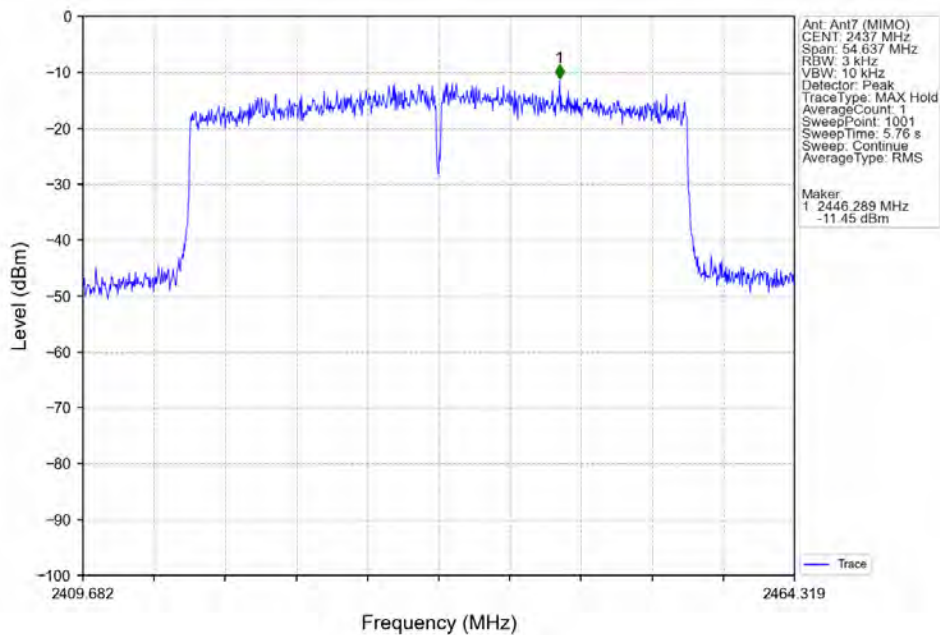
802.11ax(HEW40)_MCH_2437MHz_RU484_Left_Ant7 (MIMO)_NTNV
