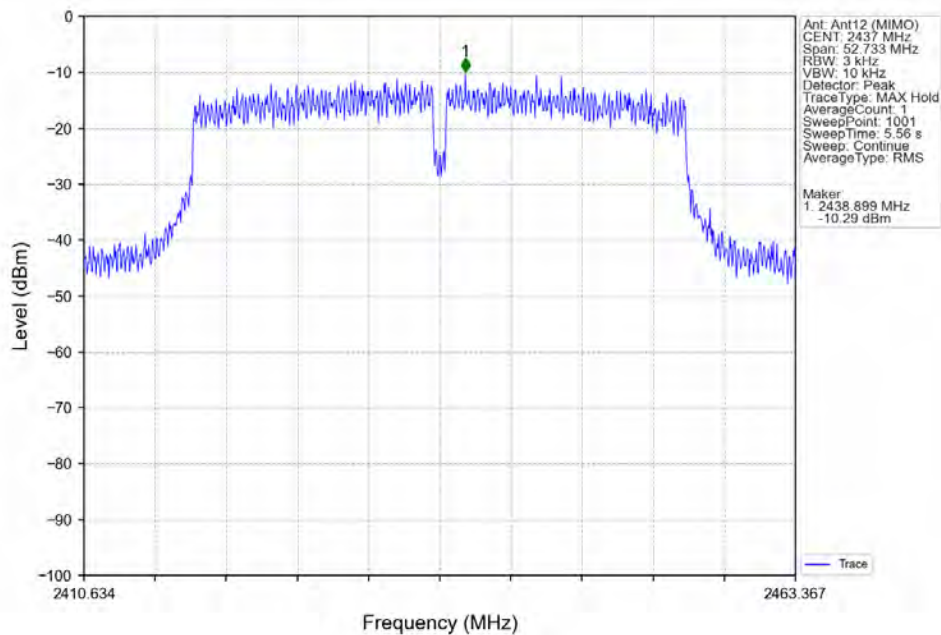
802.11ac(VHT40)_MCH_2437MHz_Ant12 (MIMO)_NTNV
