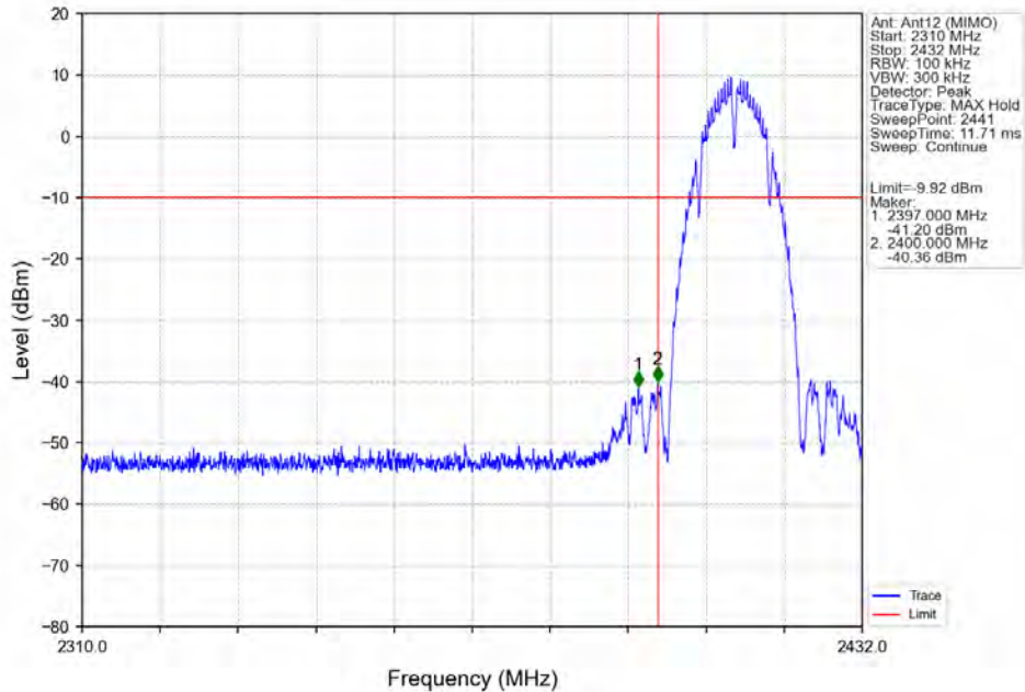
802.11b_LCH_2412MHz_Ant12 (MIMO)_NTNV
