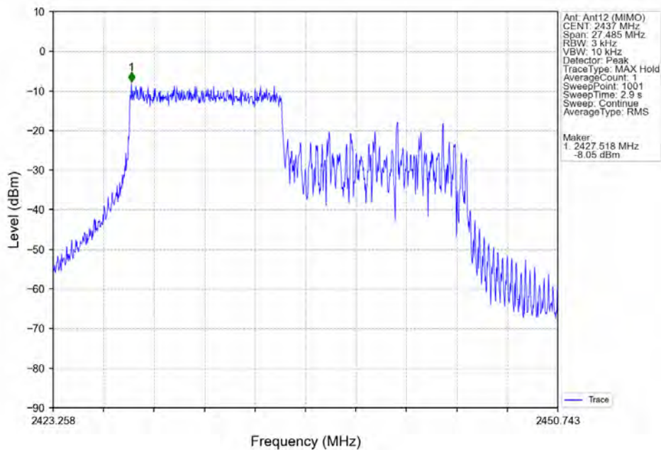
802.11ax(HEW20)_MCH_2437MHz_RU106_Left_Ant12 (MIMO)_NTNV
