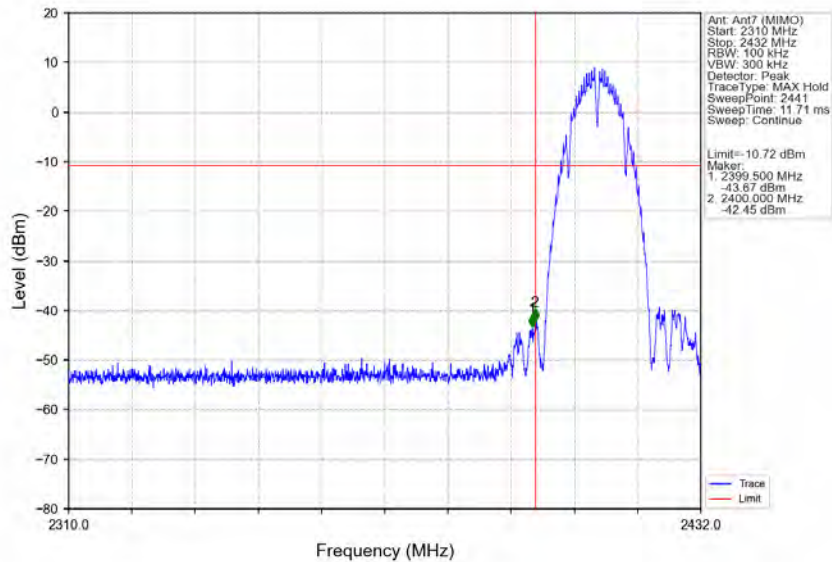
802.11b_LCH_2412MHz_Ant7 (MIMO)_NTNV
