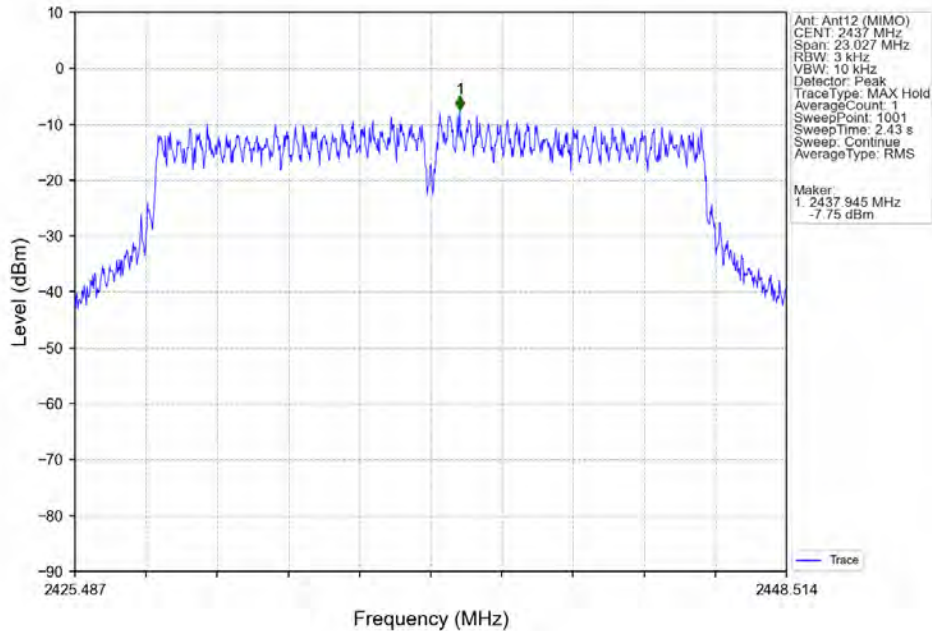
802.11ac(VHT20)_MCH_2437MHz_MIMO_NTNV
