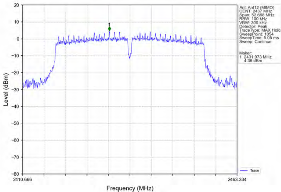
802.11n(HT40)_MCH_2437MHz_Ant12 (MIMO)_NTNV
