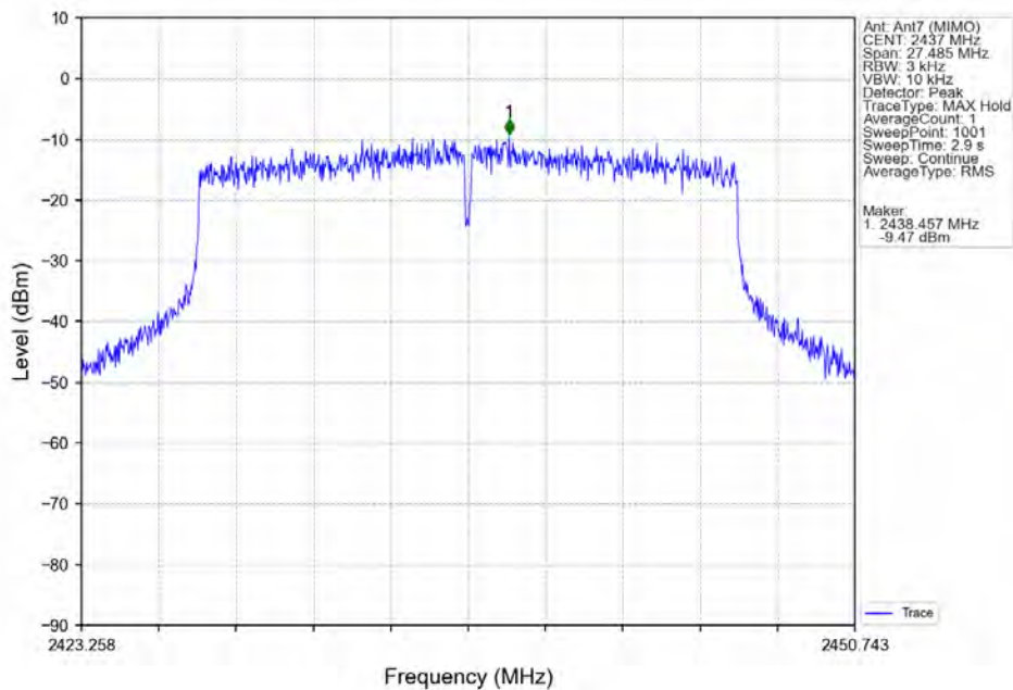
802.11ax(HEW20)_MCH_2437MHz_RU242_Left_Ant7 (MIMO)_NTNV
