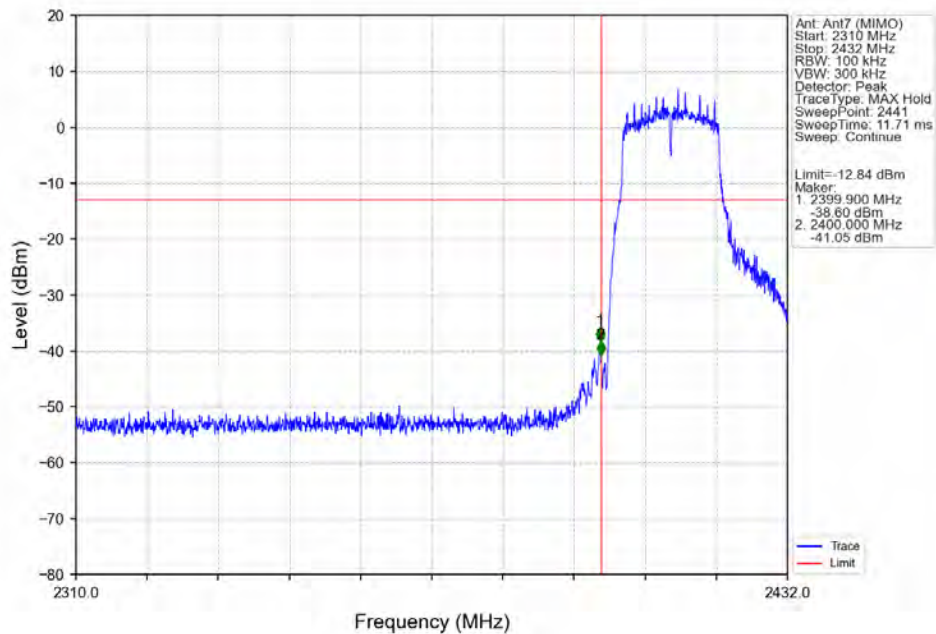
802.11g_LCH_2412MHz_Ant7 (MIMO)_NTNV
