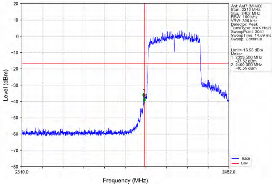
802.11ax(HEW40)_LCH_2422MHz_RU484_Left_Ant7 (MIMO)_NTNV
