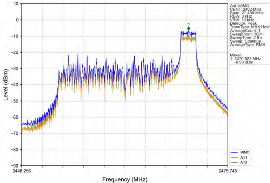
802.11ax(HEW20)_HCH_2462MHz_RU52_Right_Ant7 (MIMO)_NTNV
