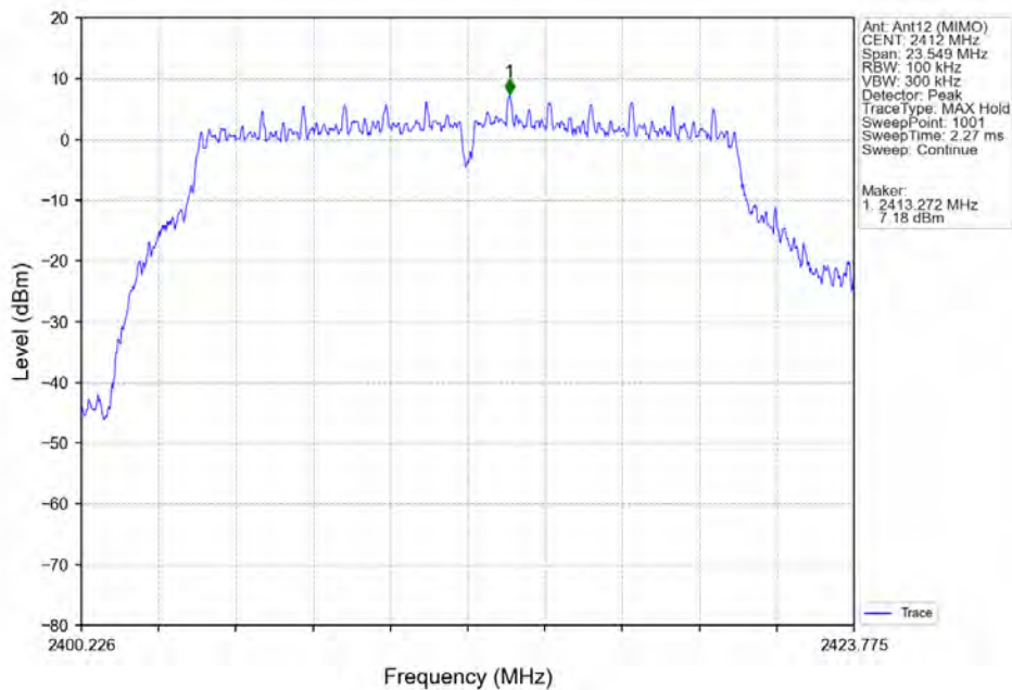
802.11g_LCH_2412MHz_Ant12 (MIMO)_NTNV
