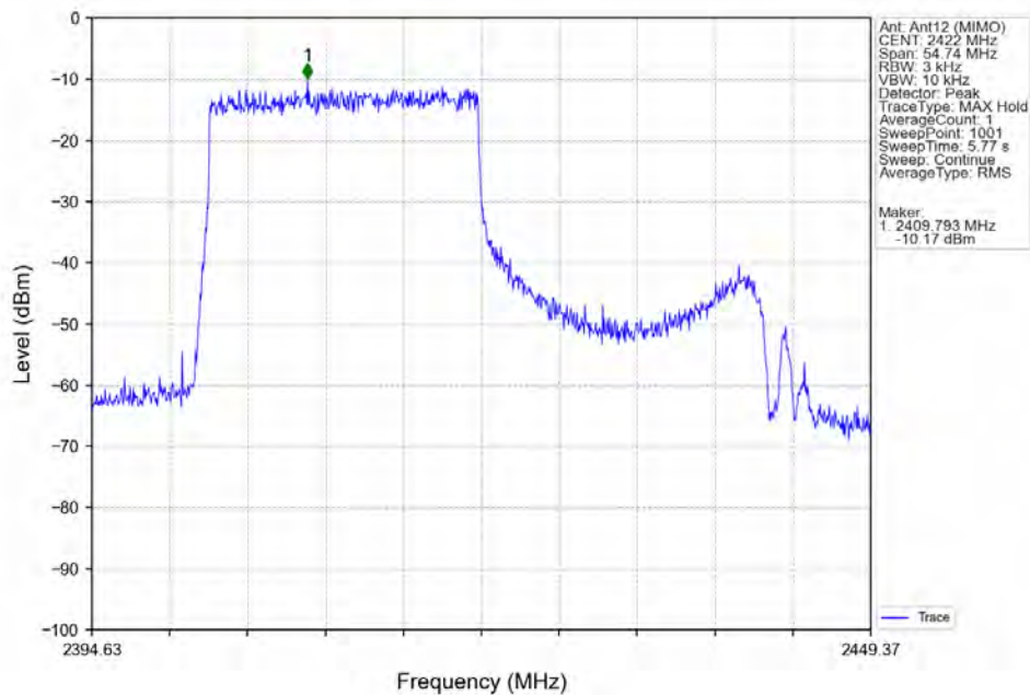
802.11ax(HEW40)_LCH_2422MHz_RU242_Left_Ant12 (MIMO)_NTNV
