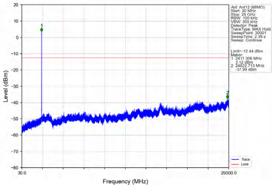
802.11g_LCH_2412MHz_Ant12 (MIMO)_NTNV
