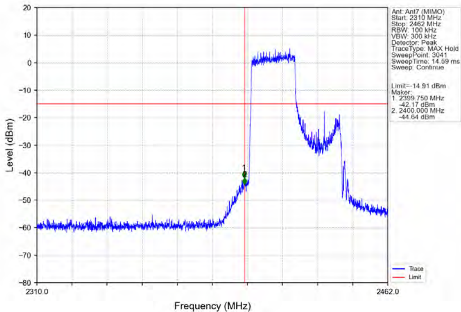
802.11ax(HEW40)_LCH_2422MHz_RU242_Left_Ant7 (MIMO)_NTNV
