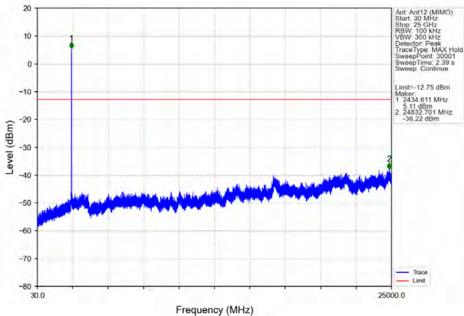
802.11n(HT20)_MCH_2437MHz_Ant12 (MIMO)_NTNV
