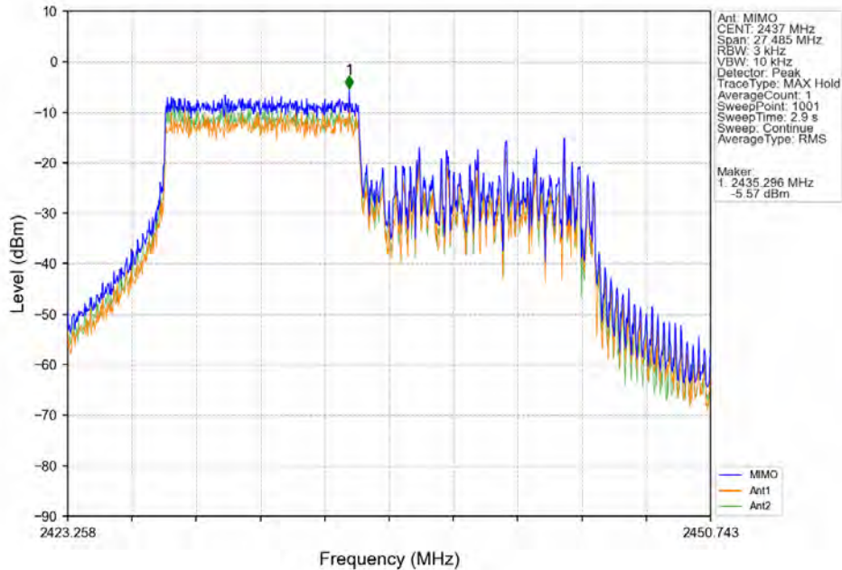
802.11ax(HEW20)_MCH_2437MHz_RU242_Left_Ant7 (MIMO)_NTNV
