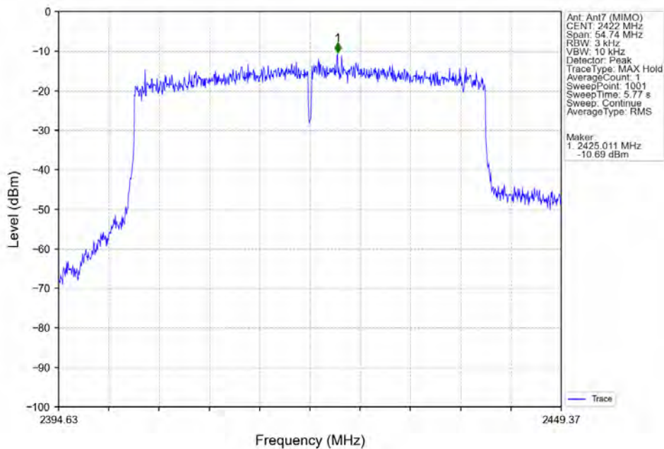
802.11ax(HEW40)_LCH_2422MHz_RU484_Left_Ant7 (MIMO)_NTNV
