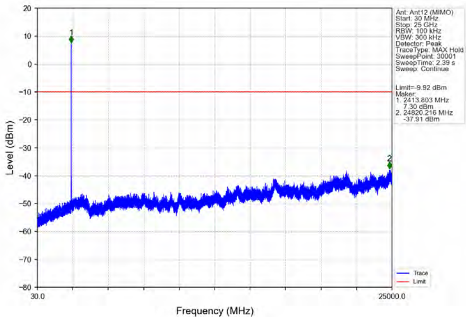
802.11b_LCH_2412MHz_Ant12 (MIMO)_NTNV
