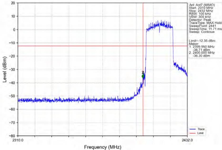
802.11ax(HEW20)_LCH_2412MHz_RU242_Left_Ant7 (MIMO)_NTNV
