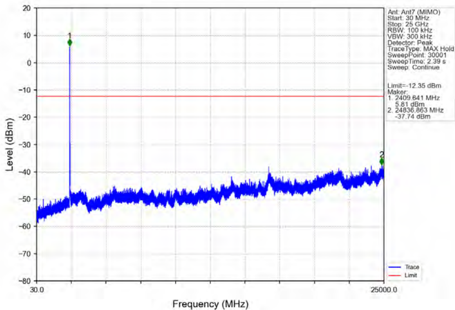
802.11ax(HEW20)_LCH_2412MHz_RU242_Left_Ant7 (MIMO)_NTNV
