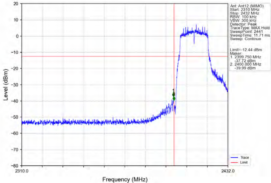
802.11g_LCH_2412MHz_Ant12 (MIMO)_NTNV
