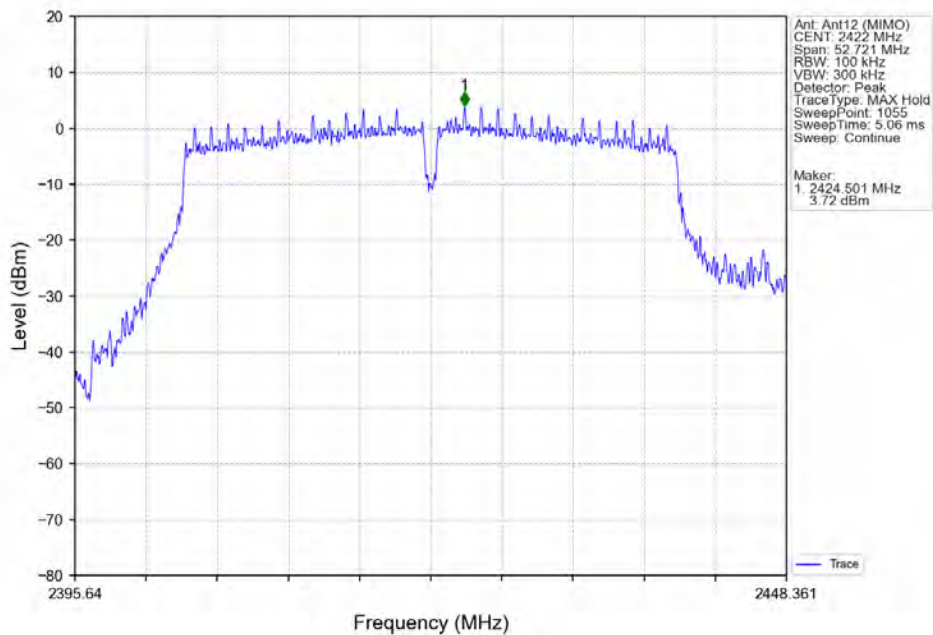
802.11n(HT40)_LCH_2422MHz_Ant12 (MIMO)_NTNV
