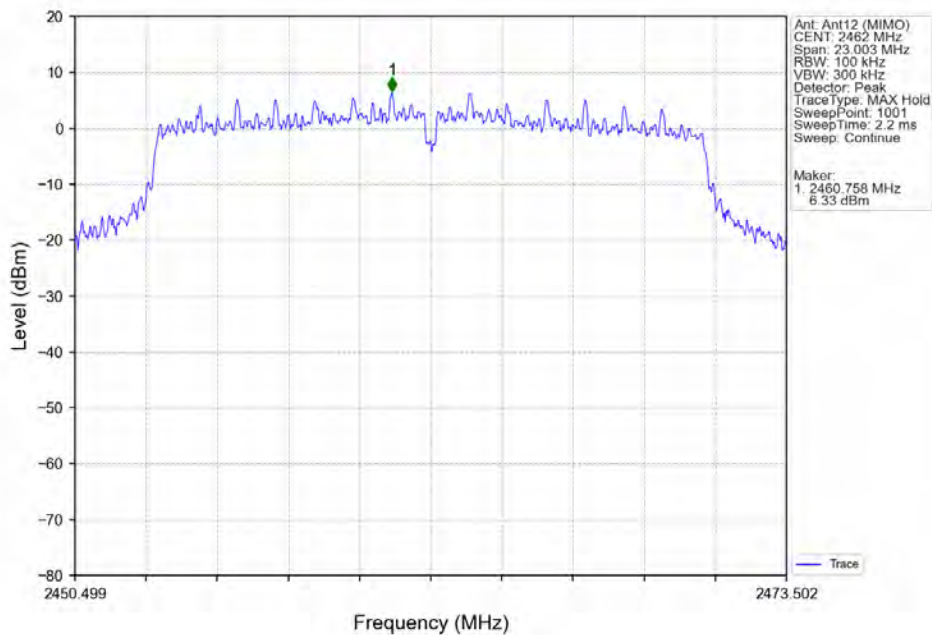
802.11ac(VHT20)_HCH_2462MHz_Ant12 (MIMO)_NTNV
