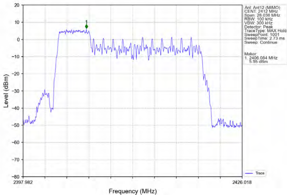
802.11ax(HEW20)_LCH_2412MHz_RU52_Left_Ant12 (MIMO)_NTNV
