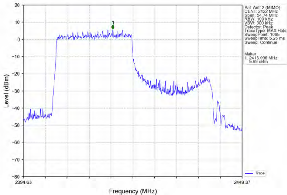
802.11ax(HEW40)_LCH_2422MHz_RU242_Left_Ant12 (MIMO)_NTNV
