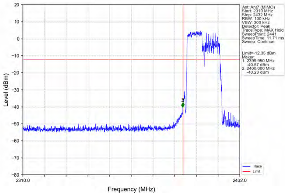
802.11ax(HEW20)_LCH_2412MHz_RU106_Left_Ant7 (MIMO)_NTNV
