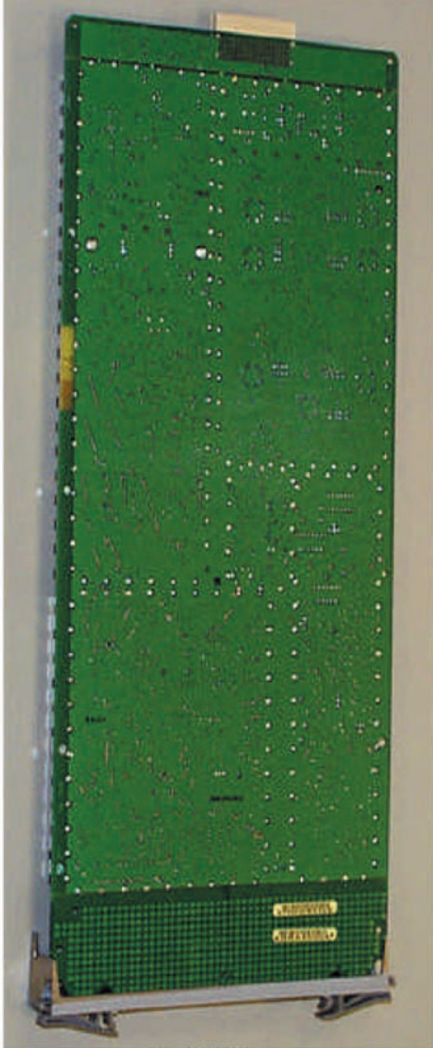
IHET6AP1 SC4812ET 1.9 GHz LFR Back
