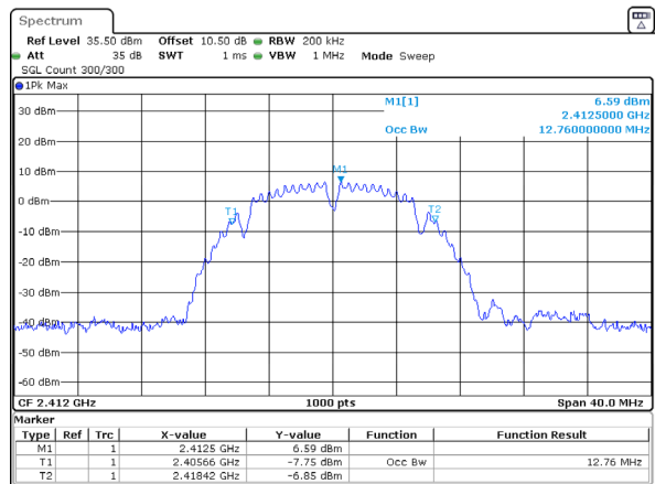
802.11b_2412MHz_Chain 0
