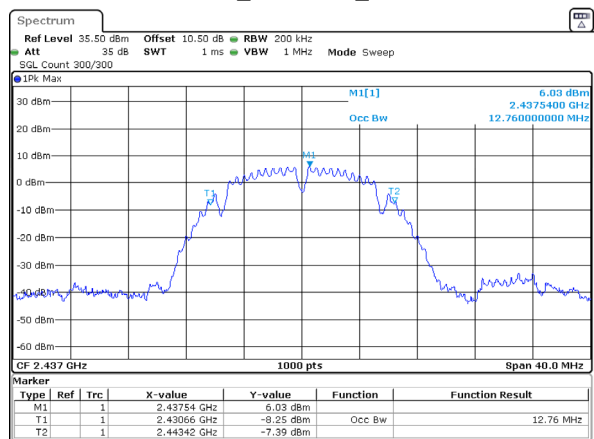
802.11b_2437MHz_Chain 1
