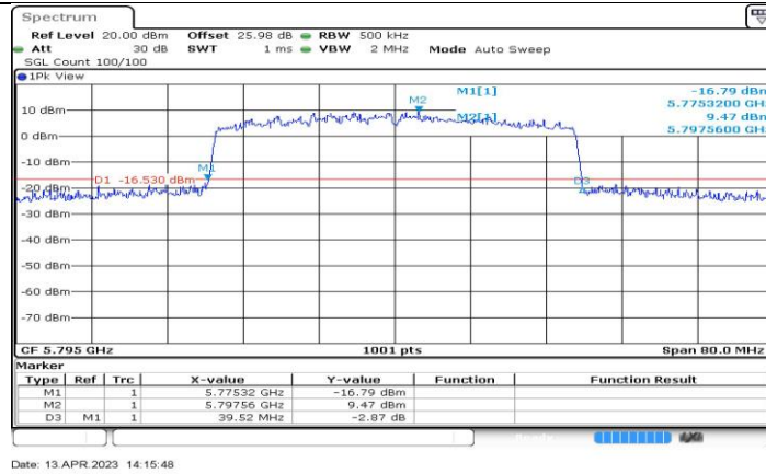
11BE40-CDD_Ant1_5795
