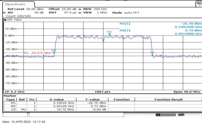
11BE20-CDD_Ant2_5200
