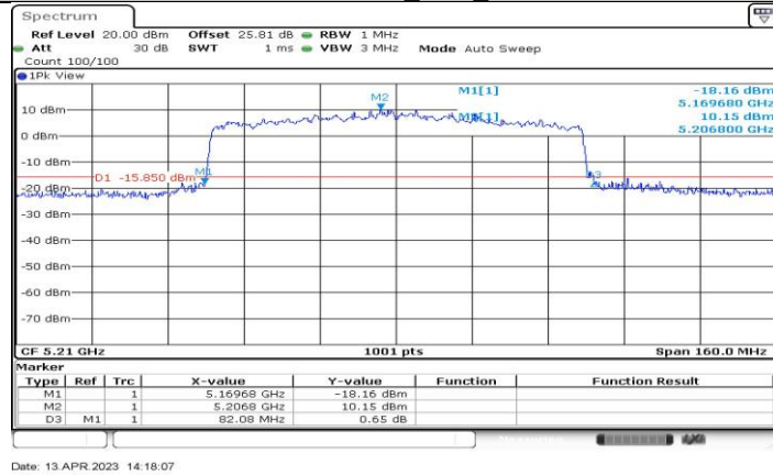
11BE80-CDD_Ant2_5210
