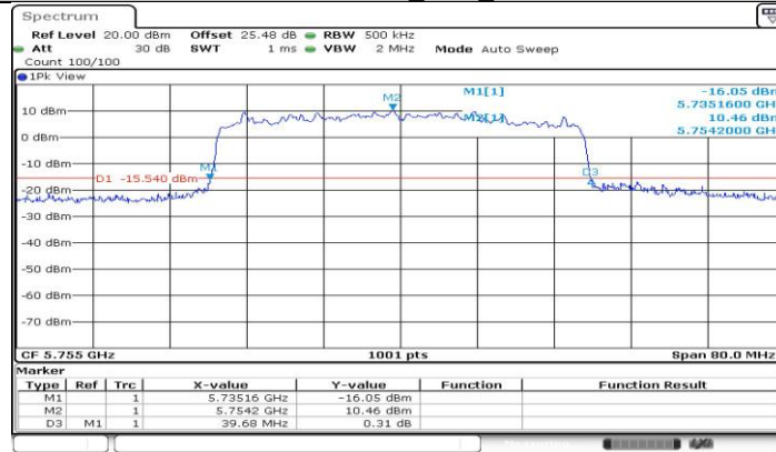
11BE40-CDD_Ant3_5755
