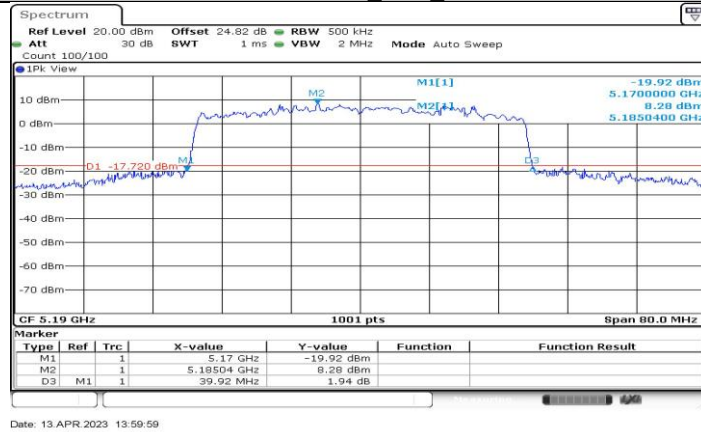
11BE40-CDD_Ant3_5190
