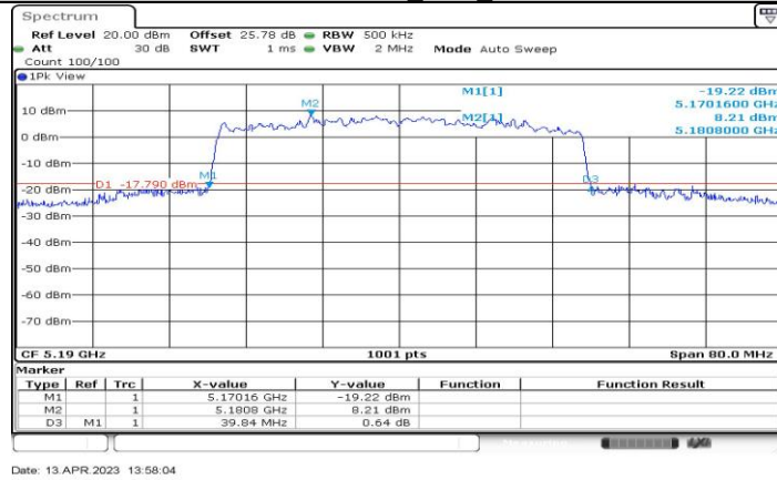
11BE40-CDD_Ant2_5190
