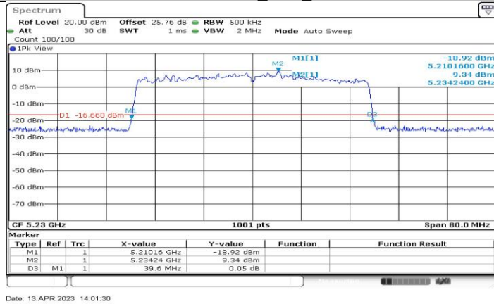
11BE40-CDD_Ant2_5230
