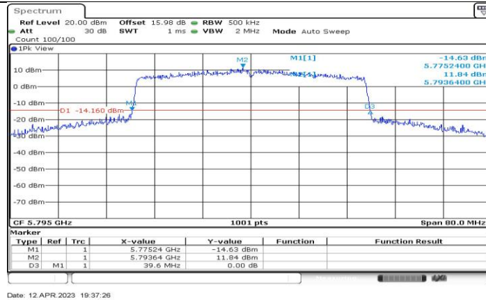
11AX40-CDD_Ant1_5795
