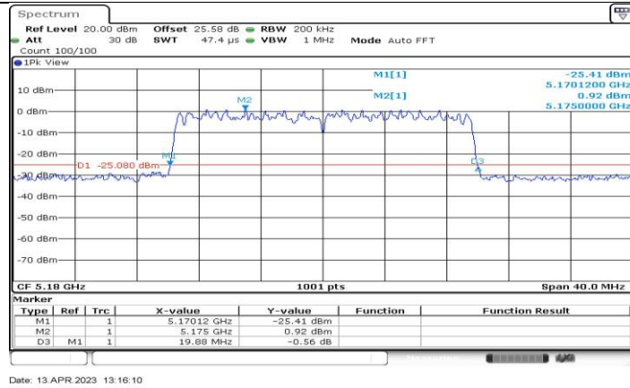
11BE20-CDD_Ant1_5180
