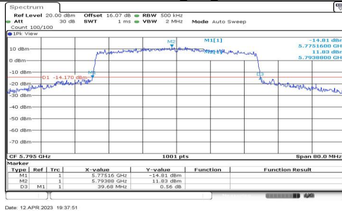
11AX40-CDD_Ant2_5795
