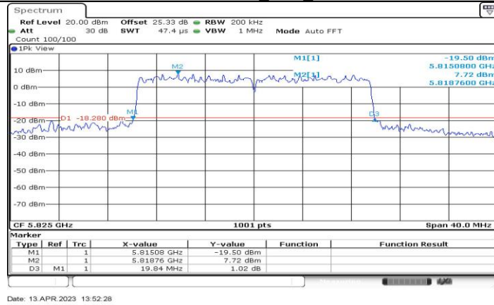
11BE20-CDD_Ant3_5825
