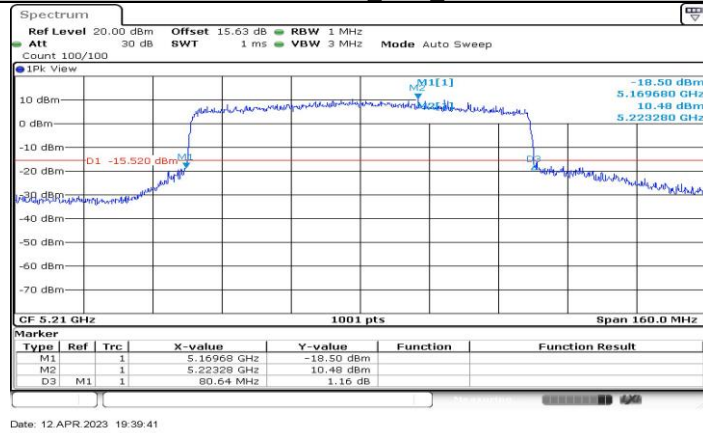
11AX80-CDD_Ant1_5210
