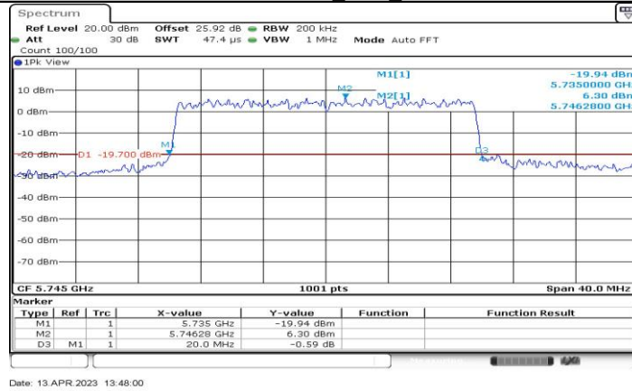
11BE20-CDD_Ant2_5745
