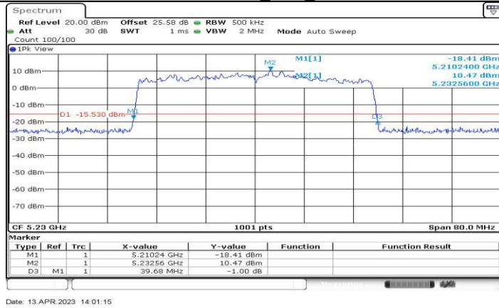
11BE40-CDD_Ant1_5230
