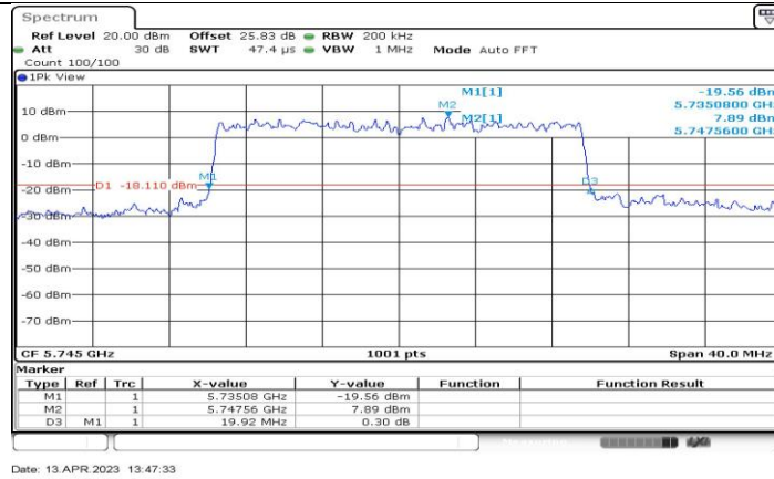
11BE20-CDD_Ant1_5745
