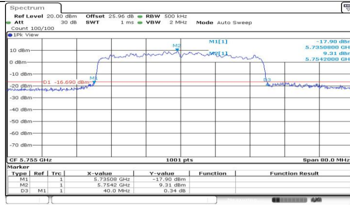
11BE40-CDD_Ant2_5755
