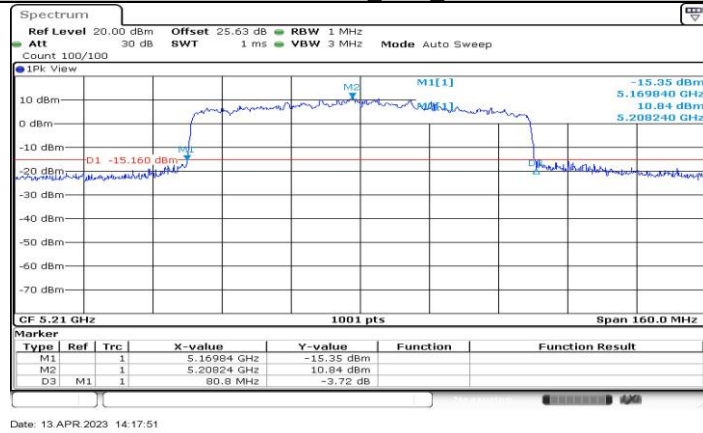
11BE80-CDD_Ant1_5210
