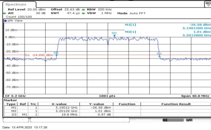
11BE20-CDD_Ant1_5200
