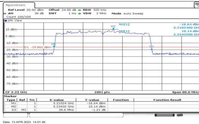
11BE40-CDD_Ant3_5230
