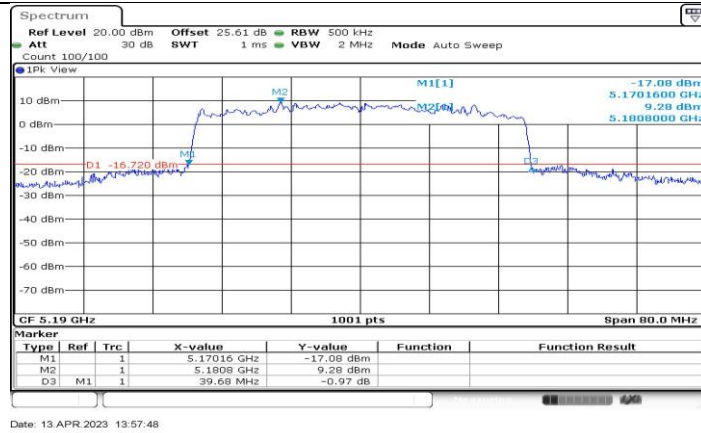
11BE40-CDD_Ant1_5190
