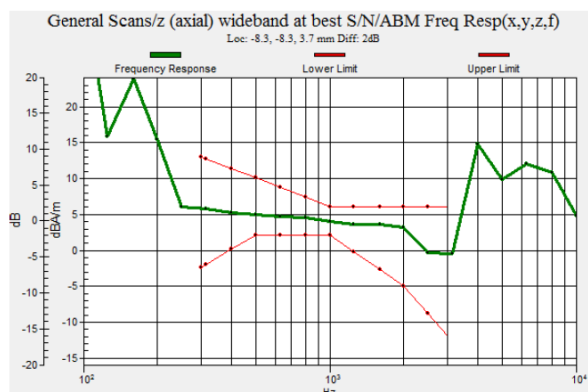
Fig 7.1 GSM850 Ch189
