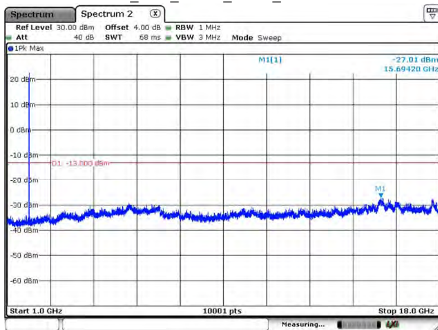
PCS_1900_CH512_GPRS_Above 1G
