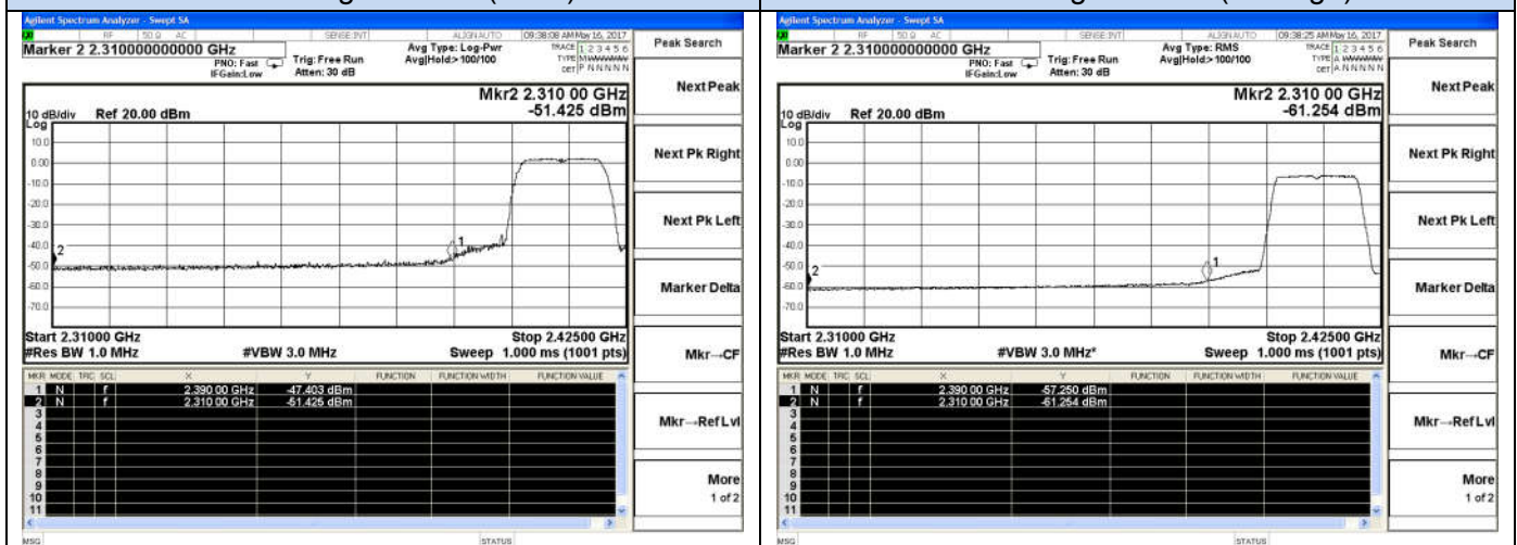
802.11g-Low channel(Average)
