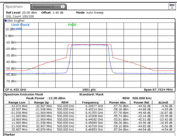
802.11ax (20MHz) 6435MHz Chain B NSS-1
