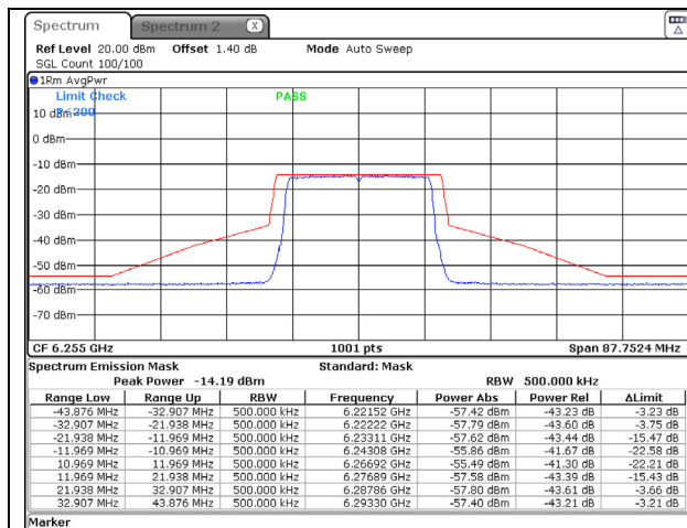
802.11ax (20MHz) 6255MHz Chain C NSS-1
