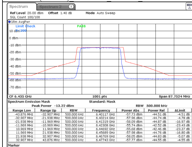
802.11ax (20MHz) 6435MHz Chain C NSS-1
