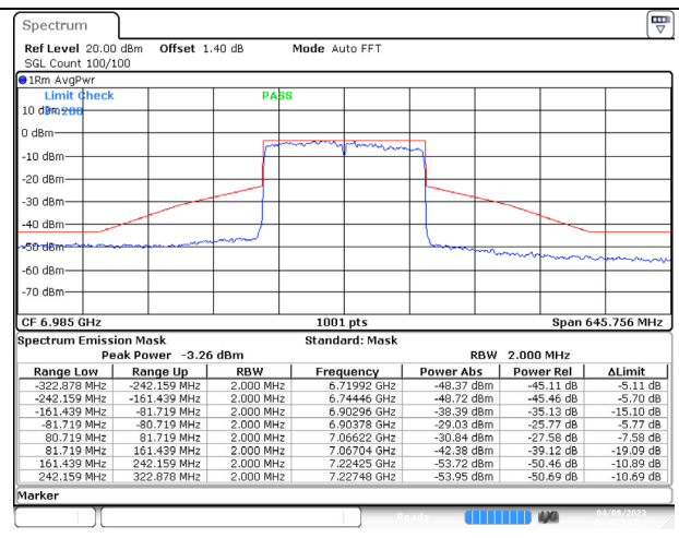
802.11ax (160MHz) 6985MHz Chain B NSS-4
