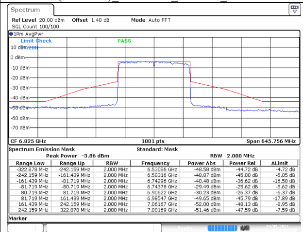
802.11ax (160MHz) 6825MHz Chain D NSS-4
