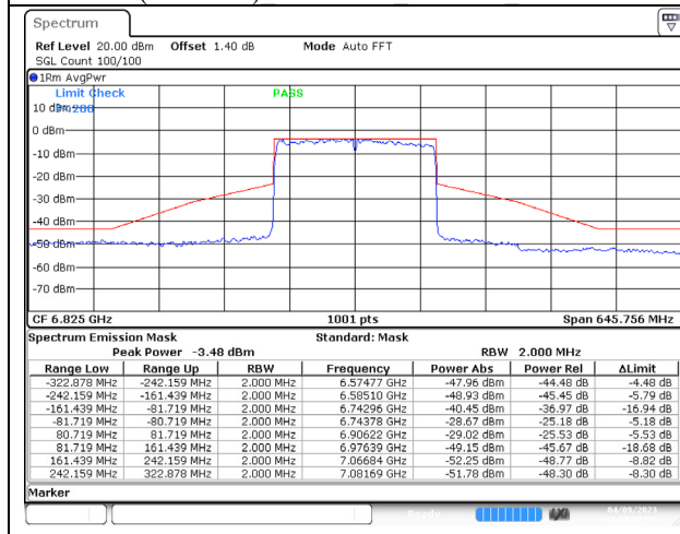
802.11ax (160MHz) 6825MHz Chain A NSS-4
