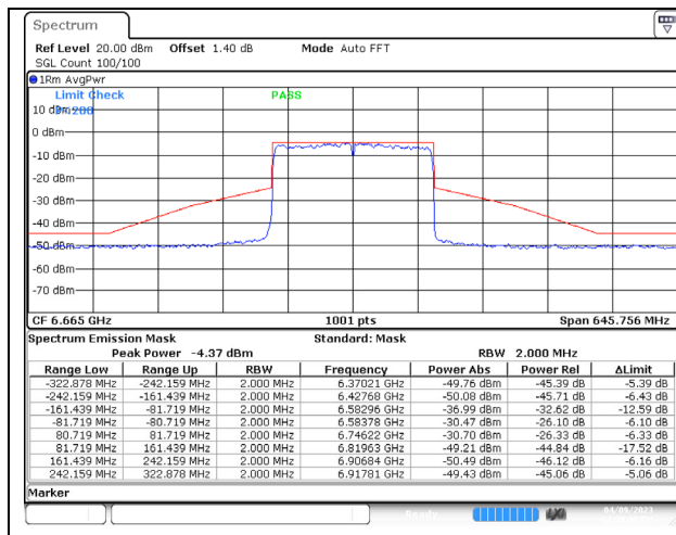
802.11ax (160MHz) 6665MHz Chain C NSS-4
