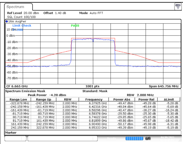
802.11ax (160MHz) 6665MHz Chain D NSS-4
