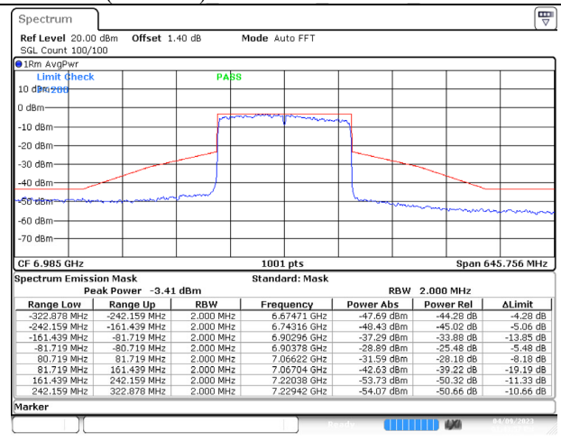
802.11ax (160MHz) 6985MHz Chain D NSS-4
