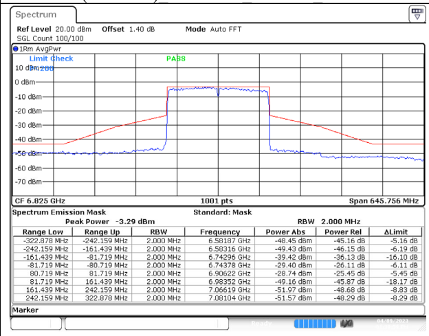
802.11ax (160MHz) 6825MHz Chain B NSS-4
