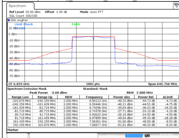
802.11ax (160MHz) 6825MHz Chain C NSS-4
