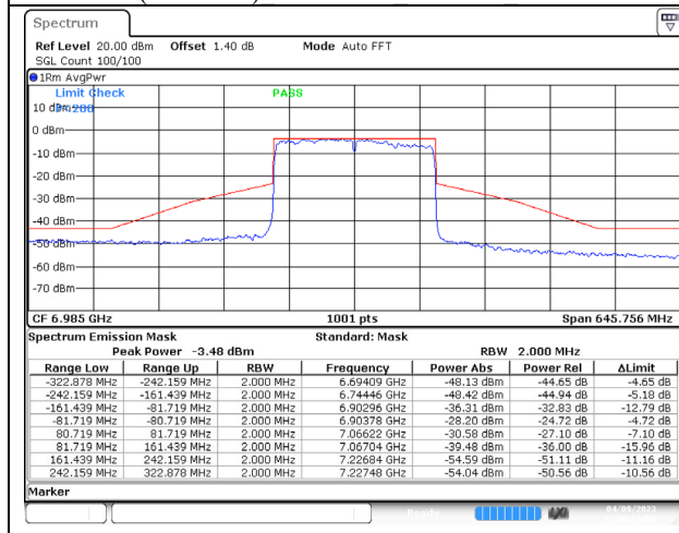
802.11ax (160MHz) 6985MHz Chain C NSS-4
