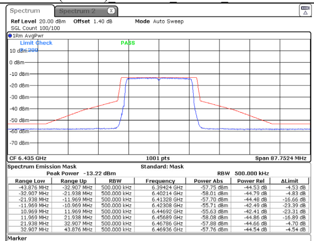
802.11ax (20MHz) 6435MHz Chain D NSS-1
