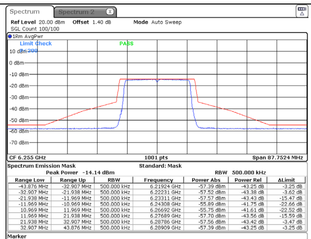
802.11ax (20MHz) 6255MHz Chain D NSS-1
