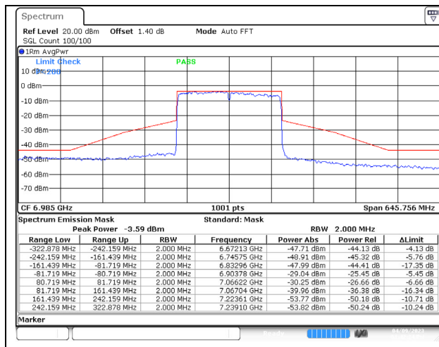
802.11ax (160MHz) 6985MHz Chain A NSS-4
