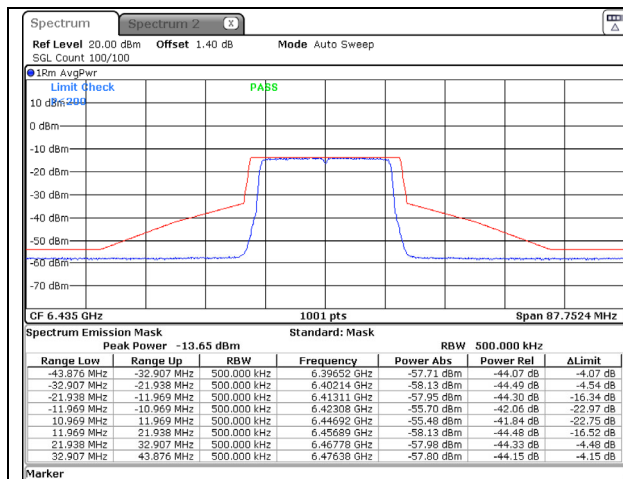
802.11ax (20MHz) 6435MHz Chain A NSS-1
