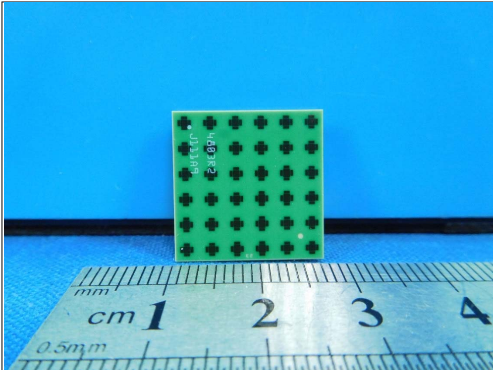
WiGig Antenna
