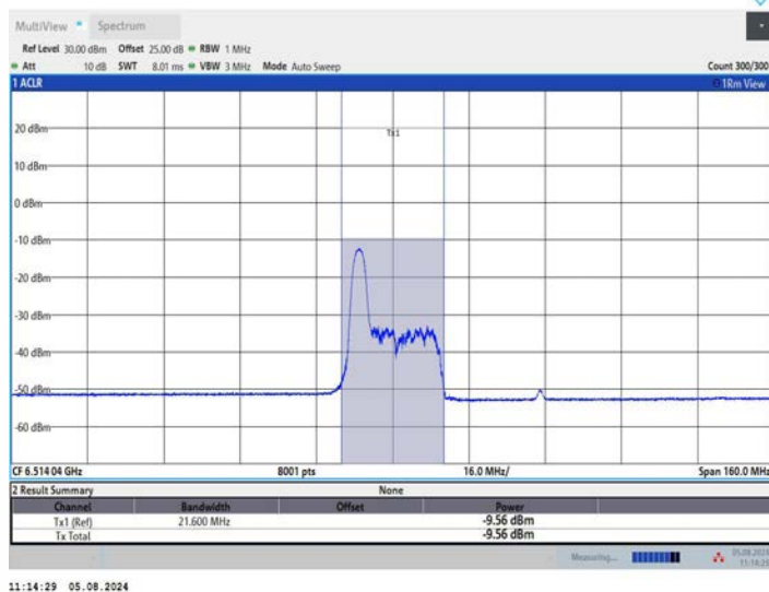
11AX80MIMO_Ant2_6545_52Tone_RU37
