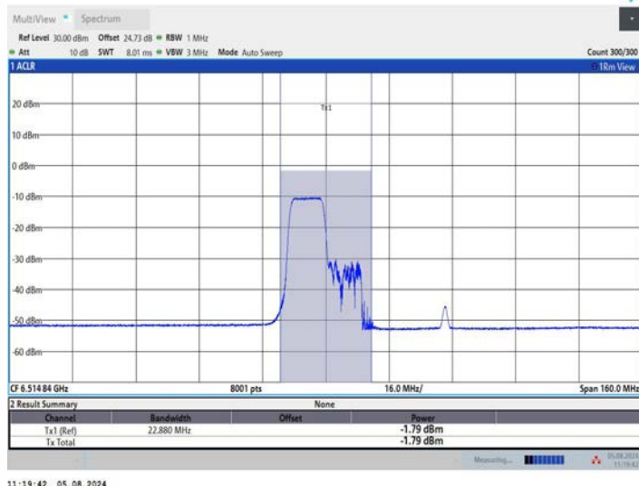
11AX80MIMO_Ant1_6545_242Tone_RU61
