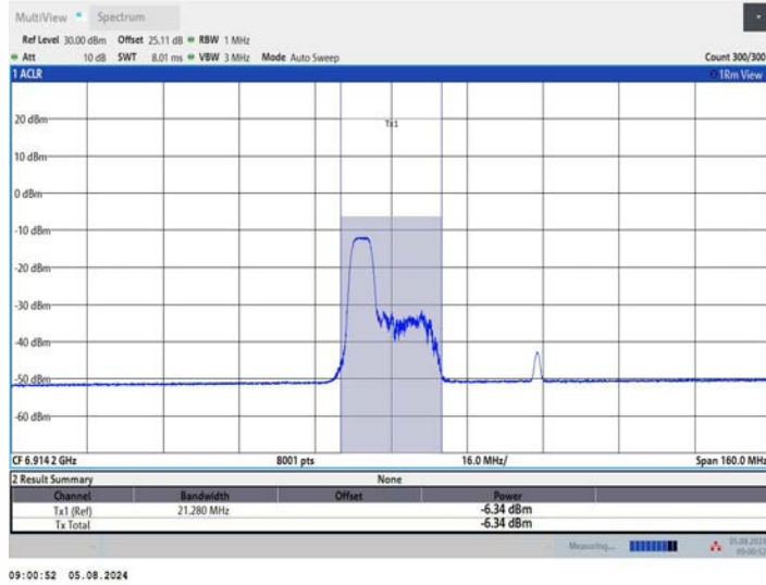
11AX80MIMO_Ant2_6945_106Tone_RU53
