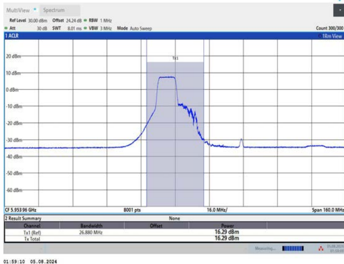
11AX80MIMO_Ant1_5985_242Tone_RU61
