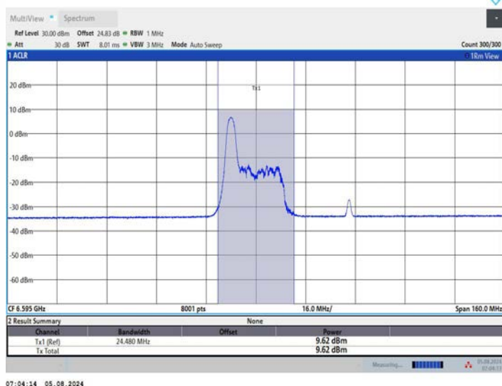
11AX80MIMO_Ant2_6625_52Tone_RU37
