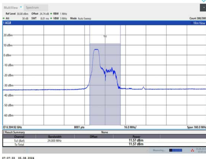
11AX80MIMO_Ant1_6625_106Tone_RU53
