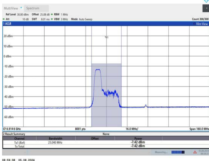
11AX80MIMO_Ant1_6945_106Tone_RU53
