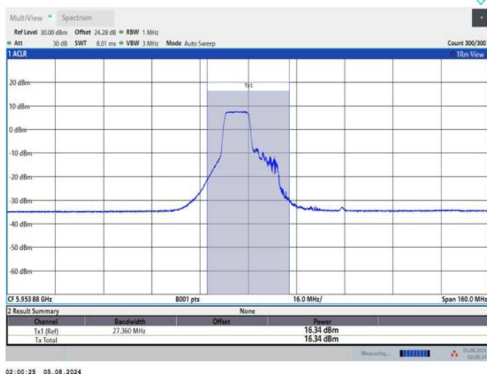
11AX80MIMO_Ant2_5985_242Tone_RU61
