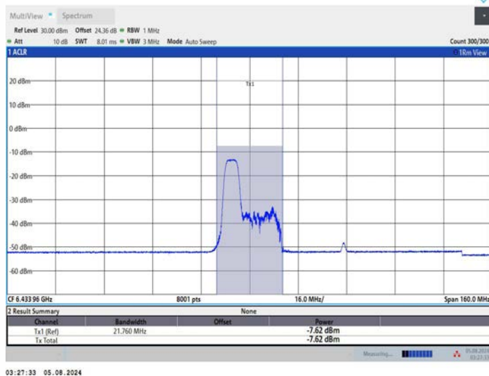
11AX80MIMO_Ant2_6465_106Tone_RU53
