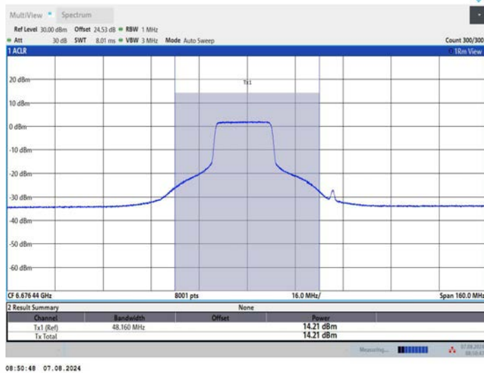
11AX80MIMO_Ant1_6705_484Tone_RU65
