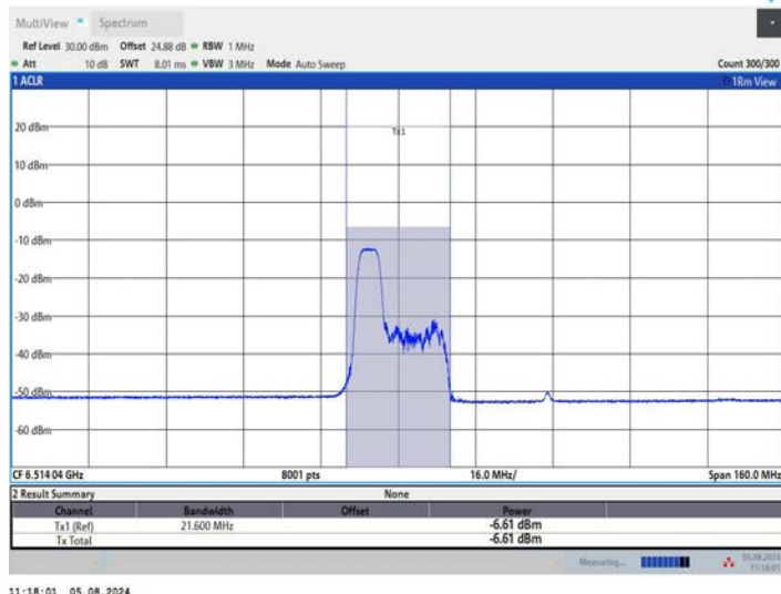
11AX80MIMO_Ant2_6545_106Tone_RU53
