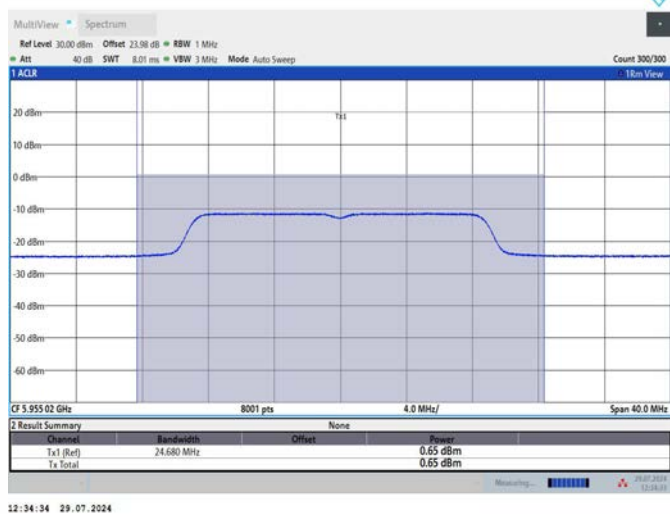
11N20MIMO_Ant2_5955
