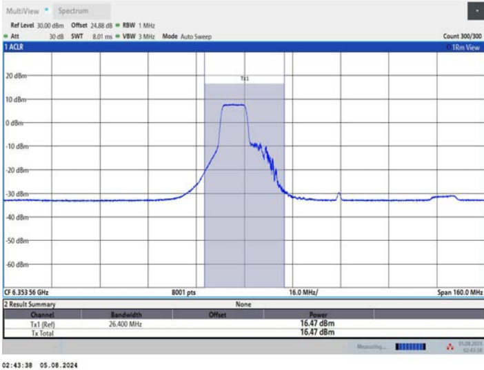
11AX80MIMO_Ant1_6385_242Tone_RU61
