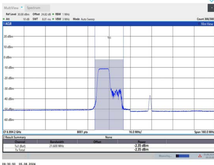
11AX80MIMO_Ant2_7025_242Tone_RU61
