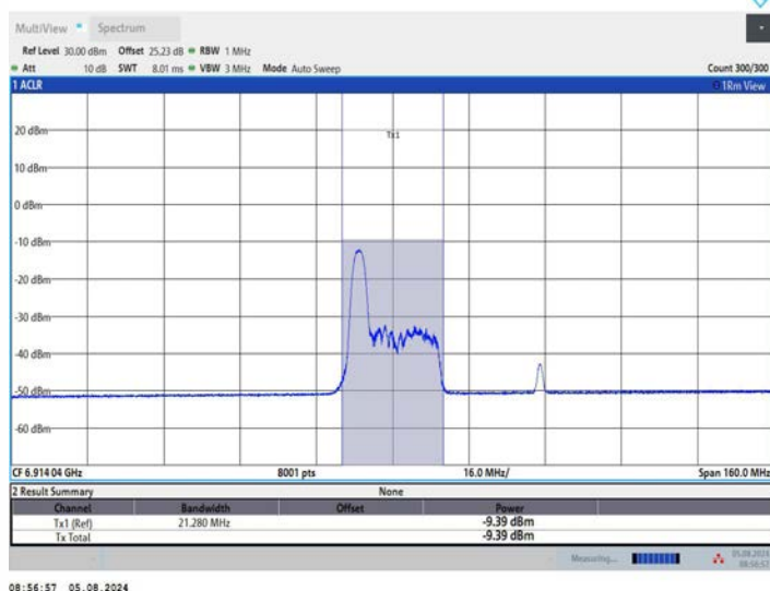
11AX80MIMO_Ant2_6945_52Tone_RU37
