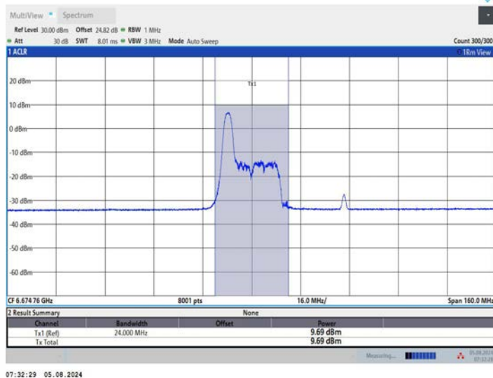
11AX80MIMO_Ant2_6705_52Tone_RU37
