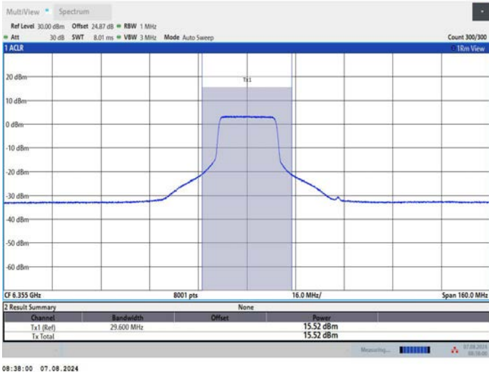
11AX80MIMO_Ant1_6385_484Tone_RU65
