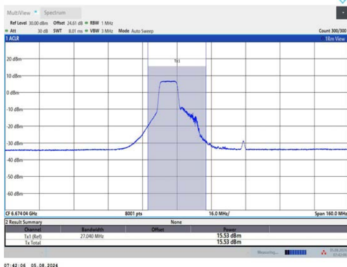
11AX80MIMO_Ant2_6705_242Tone_RU61
