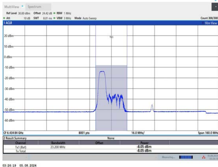
11AX80MIMO_Ant1_6465_106Tone_RU53
