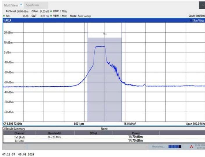
11AX80MIMO_Ant1_6625_242Tone_RU61
