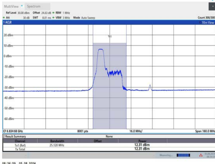
11AX80MIMO_Ant2_6865_106Tone_RU53
