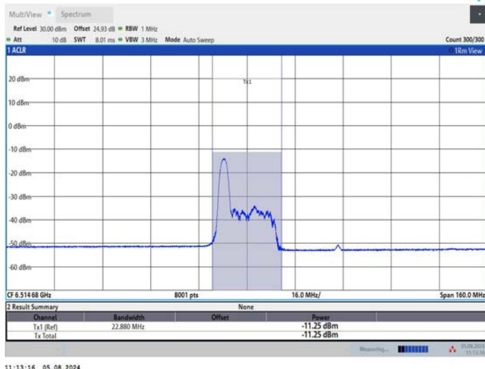
11AX80MIMO_Ant1_6545_52Tone_RU37
