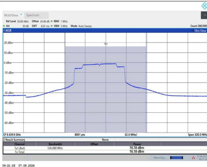
11AX160MIMO_Ant2_6665_996Tone_RU67
