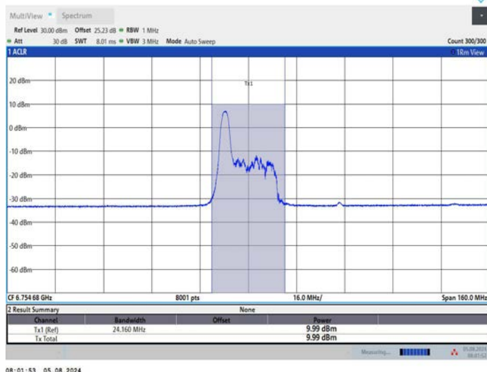
11AX80MIMO_Ant1_6785_52Tone_RU37
