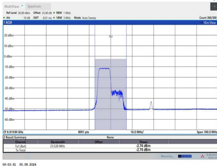
11AX80MIMO_Ant1_6945_242Tone_RU61
