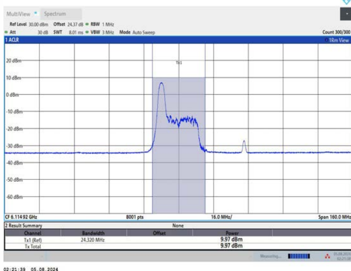
11AX80MIMO_Ant2_6145_52Tone_RU37
