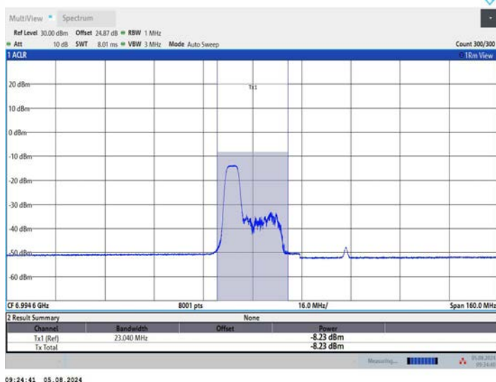
11AX80MIMO_Ant1_7025_106Tone_RU53
