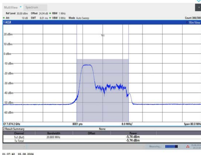
11AX40MIMO_Ant2_7085_106Tone_RU53
