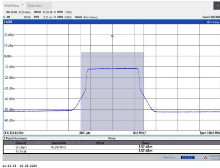
11AX80MIMO_Ant2_6545_26Tone_RU0
