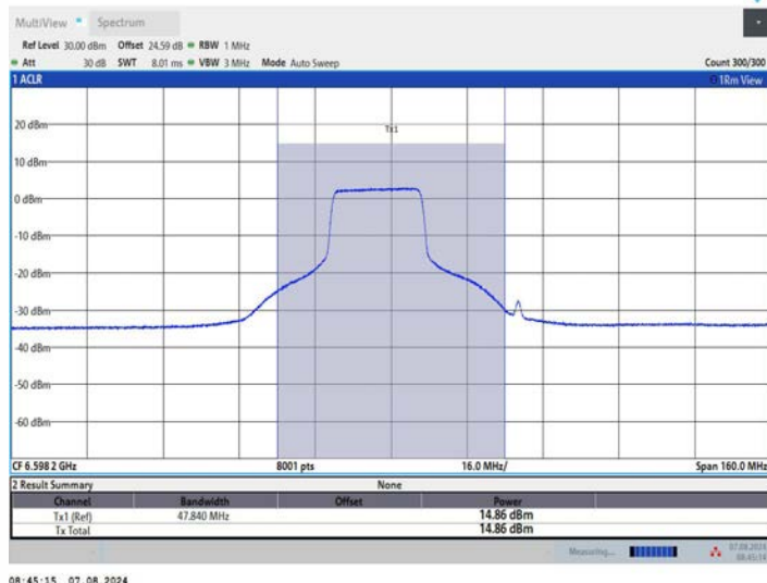
11AX80MIMO_Ant2_6625_484Tone_RU65
