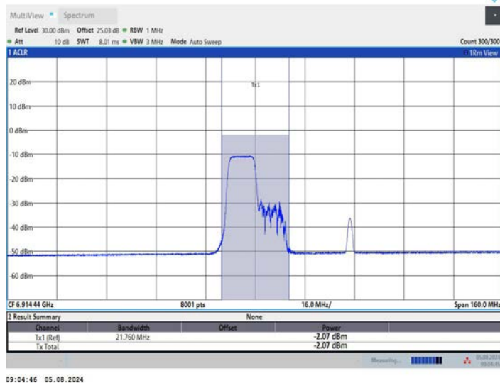
11AX80MIMO_Ant2_6945_242Tone_RU61
