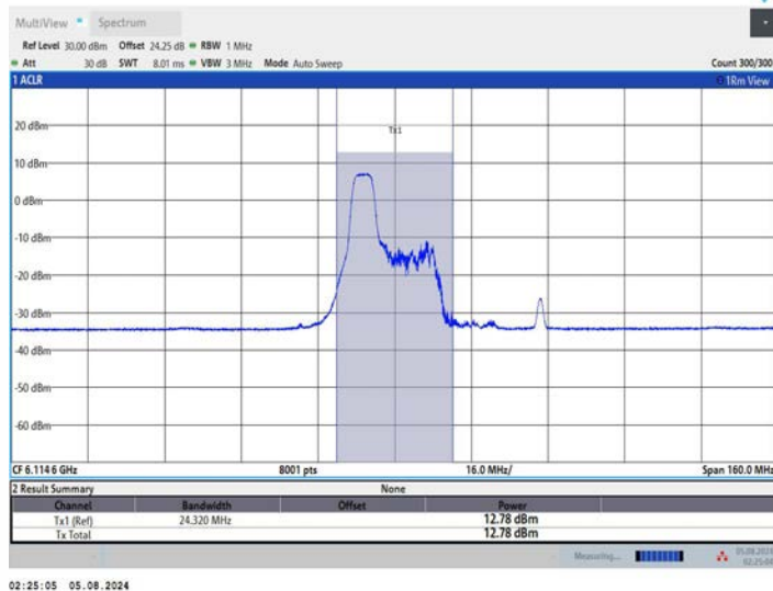
11AX80MIMO_Ant2_6145_106Tone_RU53
