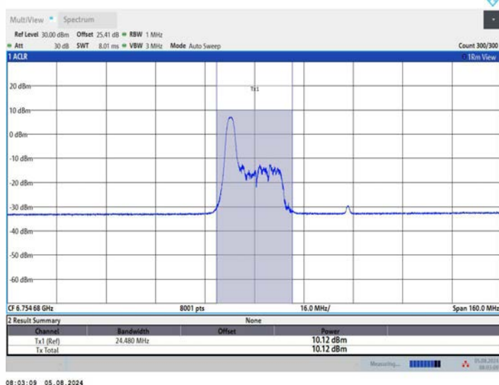
11AX80MIMO_Ant2_6785_52Tone_RU37
