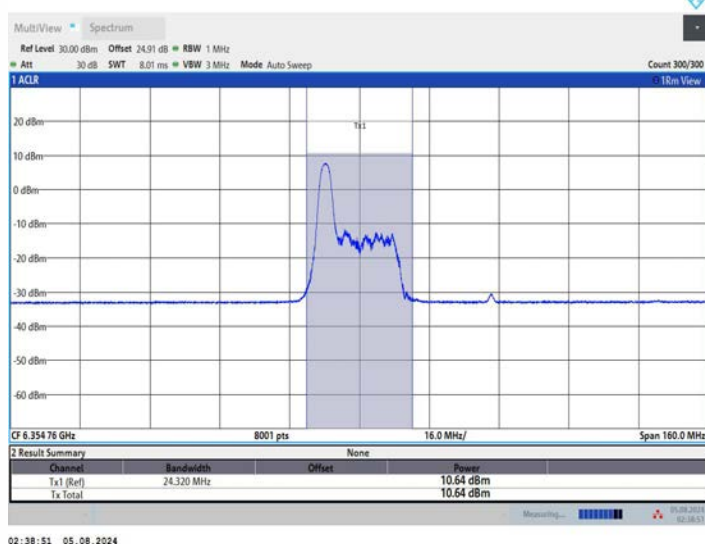
11AX80MIMO_Ant2_6385_52Tone_RU37
