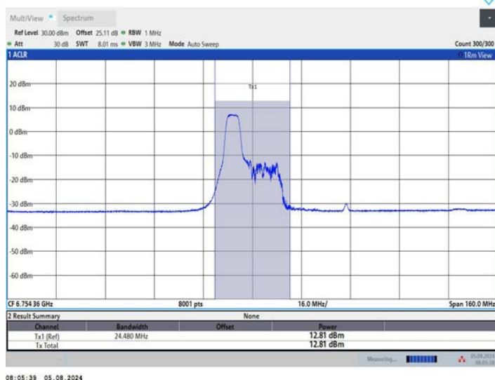
11AX80MIMO_Ant1_6785_106Tone_RU53
