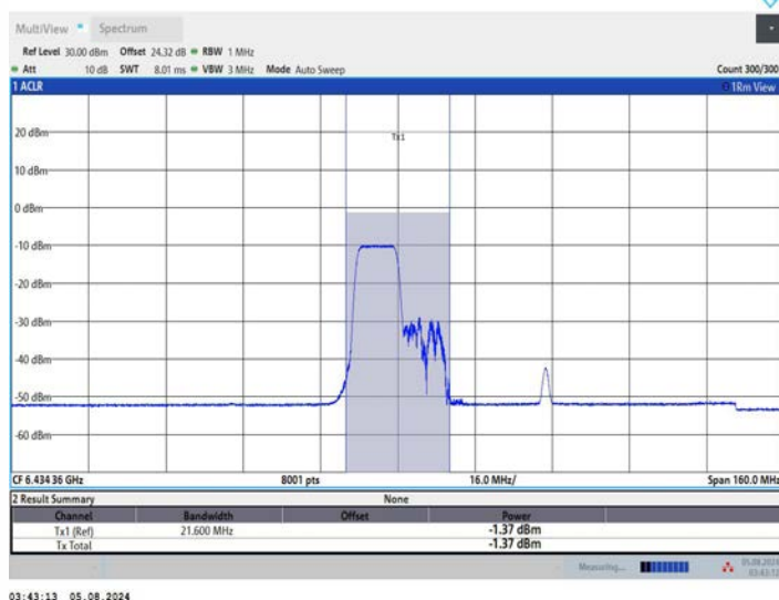
11AX80MIMO_Ant2_6465_242Tone_RU61
