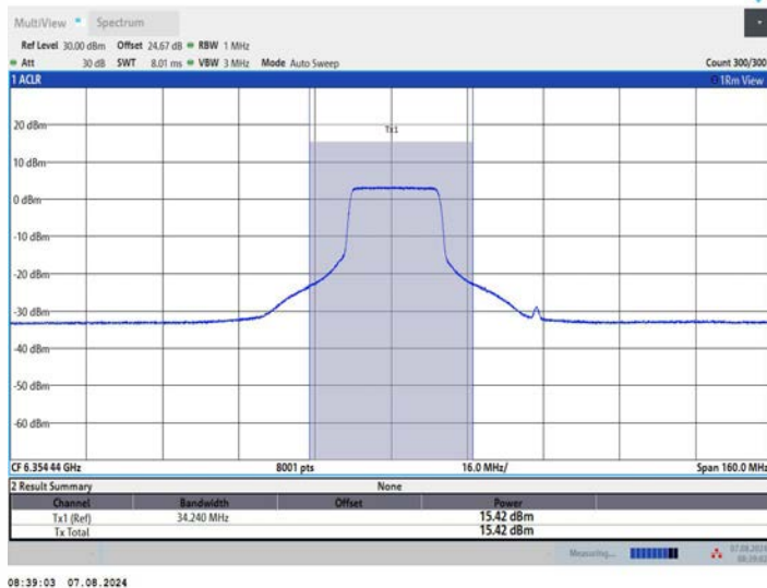
11AX80MIMO_Ant2_6385_484Tone_RU65
