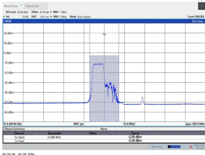
11AX80MIMO_Ant1_7025_242Tone_RU61
