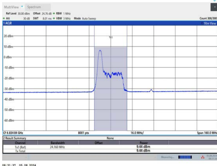
11AX80MIMO_Ant1_6865_52Tone_RU37
