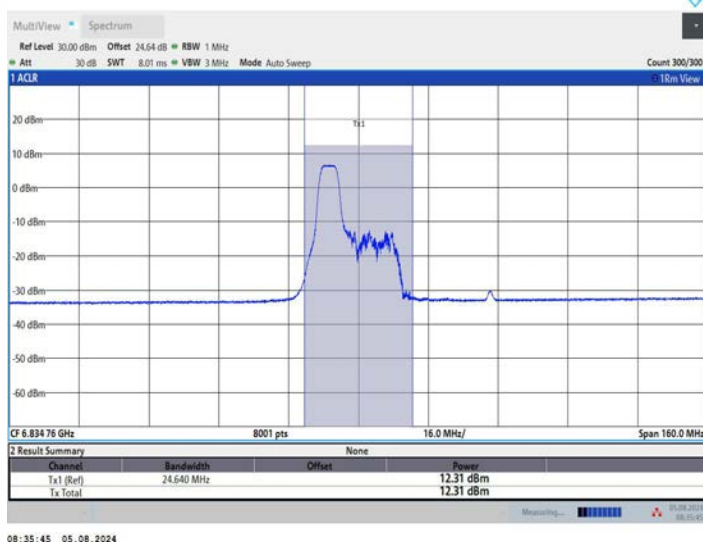
11AX80MIMO_Ant1_6865_106Tone_RU53
