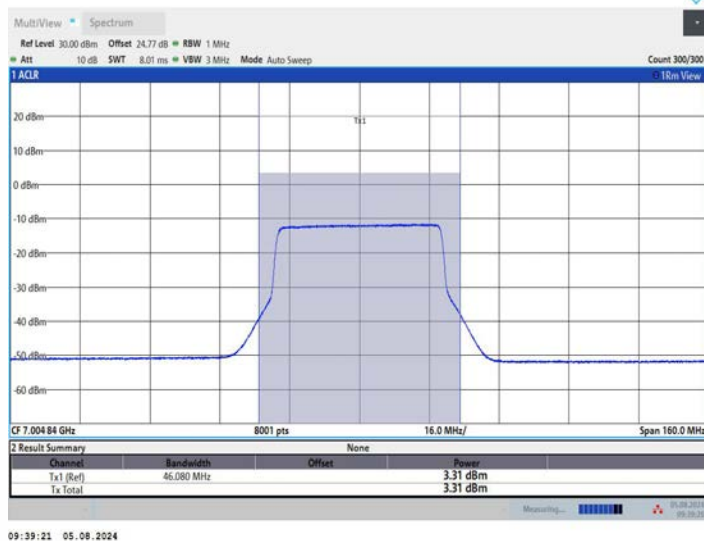
11AX80MIMO_Ant2_7025_26Tone_RU0
