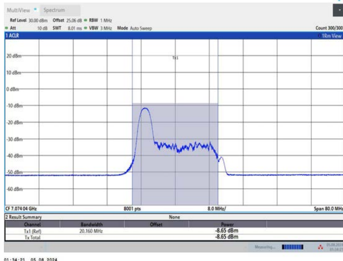
11AX40MIMO_Ant2_7085_52Tone_RU37
