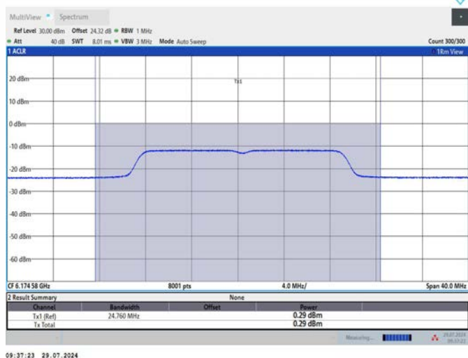
11N20MIMO_Ant1_6175
