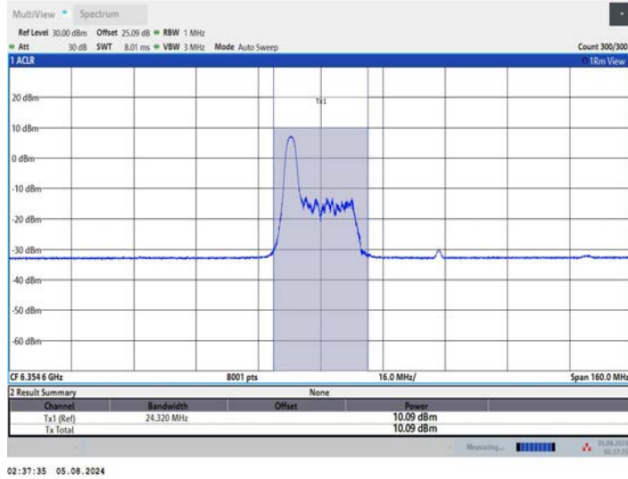
11AX80MIMO_Ant1_6385_52Tone_RU37
