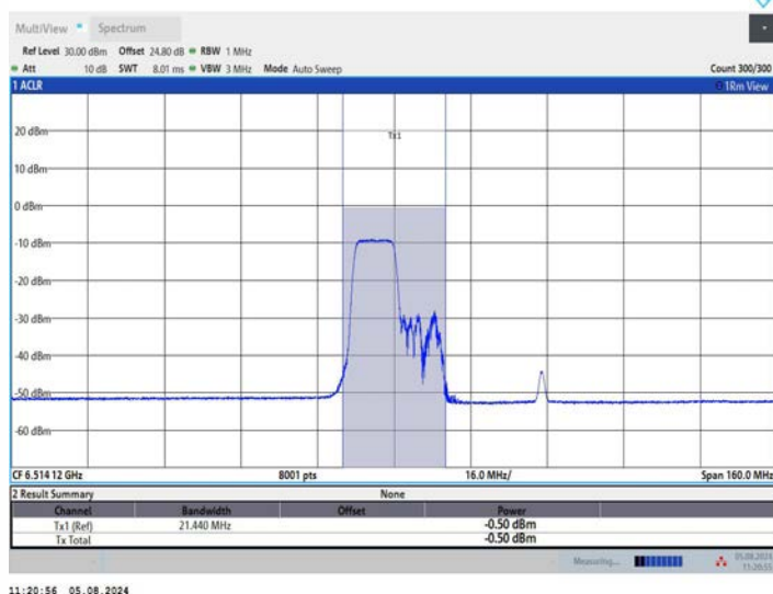
11AX80MIMO_Ant2_6545_242Tone_RU61
