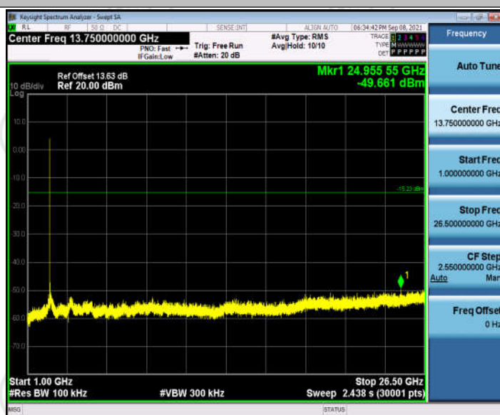
ZIGBEE_Ant1_2440_1000~26500
