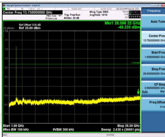
ZIGBEE_Ant1_2405_1000~26500
