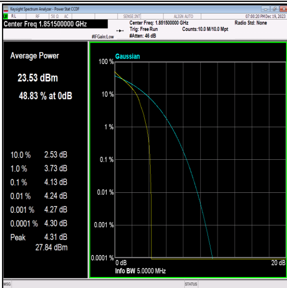
Band2-3MHz-QPSK-18615-1RB#0-PASS
