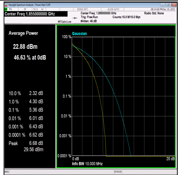
Band2-10MHz-QPSK-18650-50RB#0-PASS
