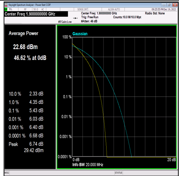
Band2-20MHz-QPSK-19100-100RB#0-PASS
