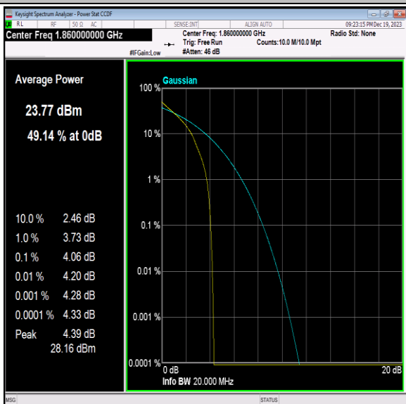
Band2-20MHz-QPSK-18700-1RB#0-PASS
