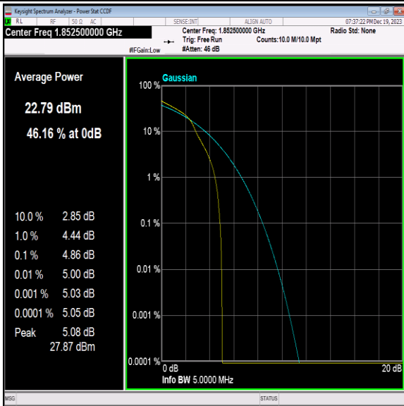
Band2-5MHz-16QAM-18625-1RB#0-PASS
