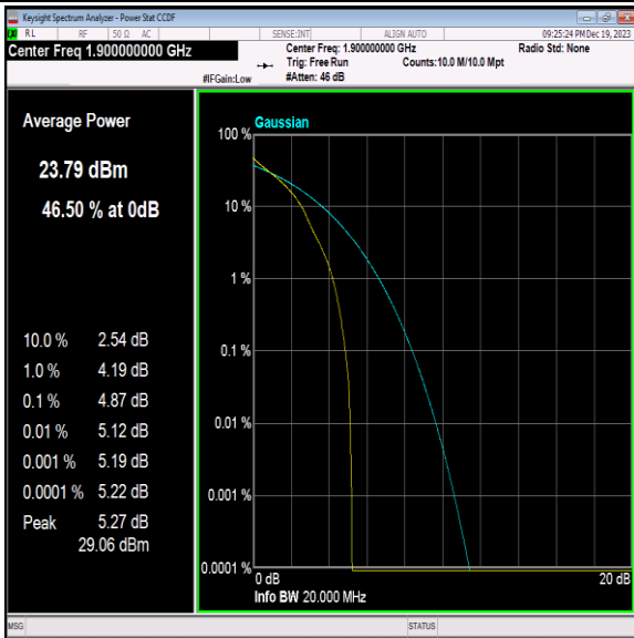
Band2-20MHz-QPSK-19100-1RB#0-PASS
