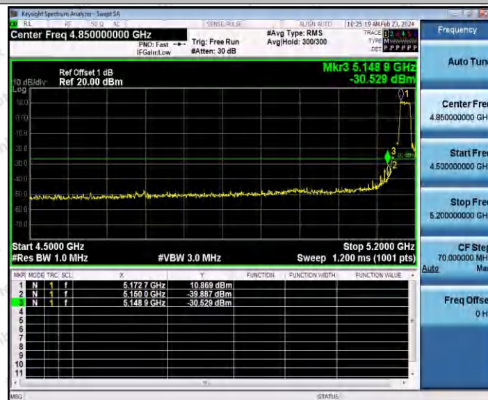
11N20MIMO_Ant1_Low_5180
