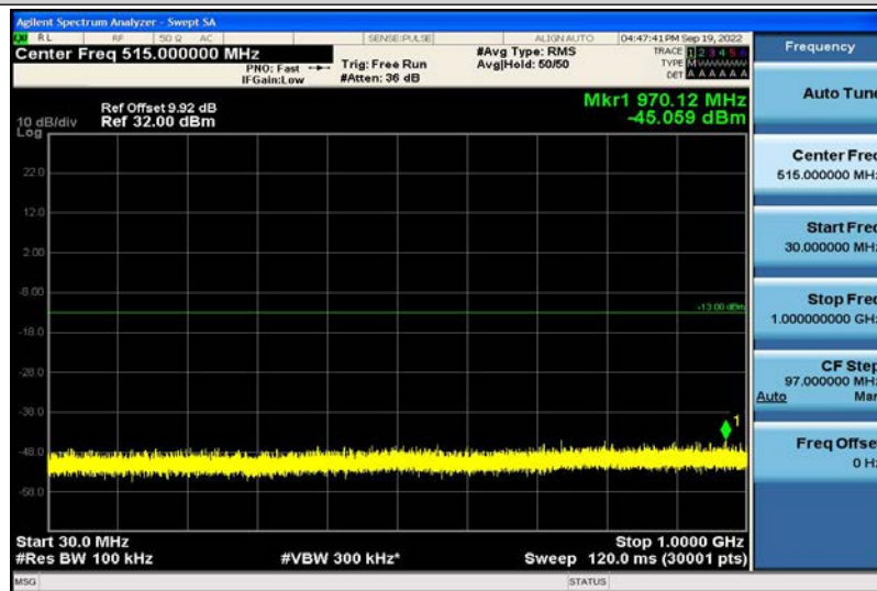
Band2-10MHz-QPSK-19150-1RB#0-30~1000MHz
