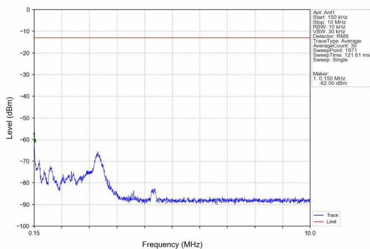
Band12 10MHz QPSK MCH 707.5MHz RB 1 0 NTV
