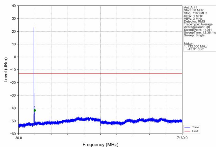
Band12 5MHz QPSK LCH 701.5MHz RB 25 0 NTNV
