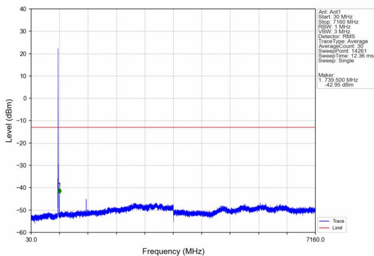
Band12 5MHz QPSK MCH 707.5MHz RB 1 0 NTNV
