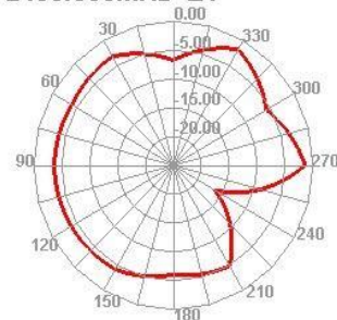
2450.000MHz E1
