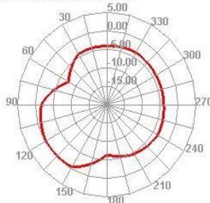
2400.000MHz E2
