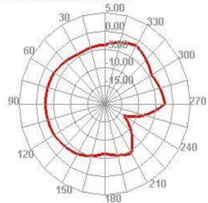
2400.000MHz E1
