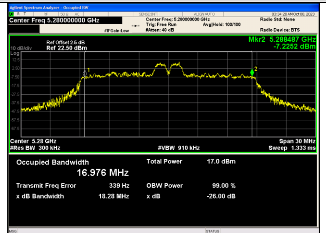
IEEE 802.11ax_Channel 56_20MHz_Antenna 1_RU&Index 26RU4
