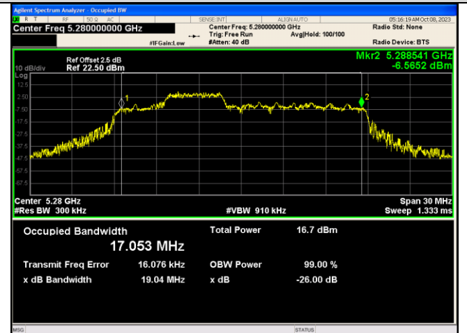
IEEE 802.11ax_Channel 56_20MHz_Antenna 1_RU&Index 52RU38
