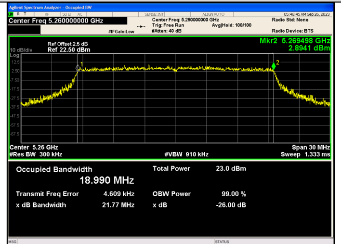
IEEE 802.11ax_Channel 52_20MHz_Antenna 1_RU&Index 242RU61
