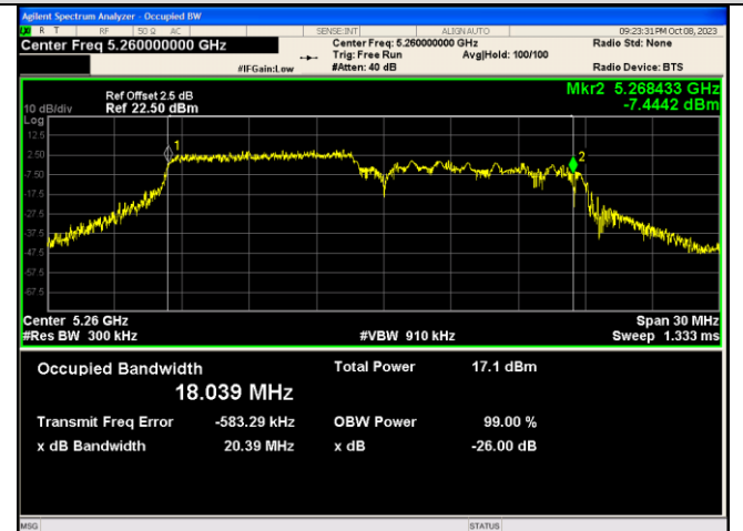
IEEE 802.11ax_Channel 52_20MHz_Antenna 1_RU&Index 106RU53
