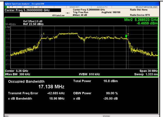
IEEE 802.11ax_Channel 52_20MHz_Antenna 1_RU&Index 52RU38
