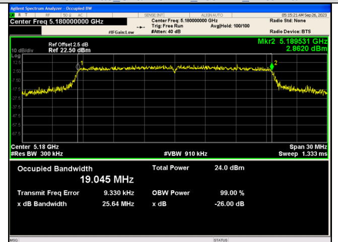
IEEE 802.11ax Channel 36 20MHz Antenna 1_RU&amp;Index 242RU61
