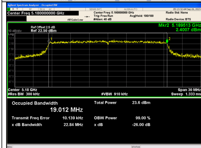
IEEE 802.11ax Channel 36 20MHz Antenna 0_RU&amp;Index 242RU61
