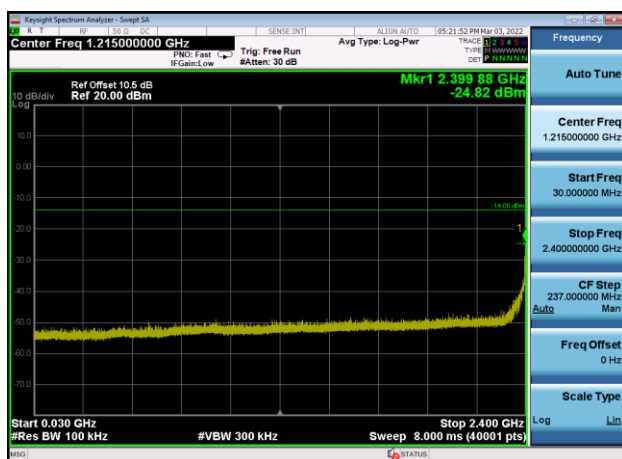
,Plot 3,30MHz~2400MHz-802.11g,2462MHz
