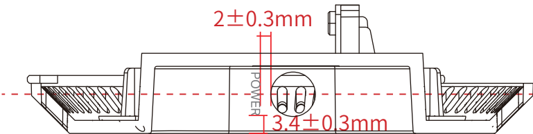
Power接口icon尺寸图
