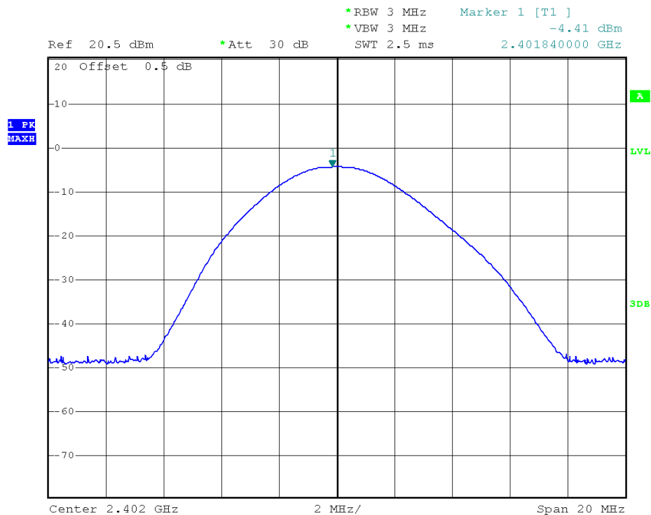
(Plot A: Channel 0: 2402MHz)
