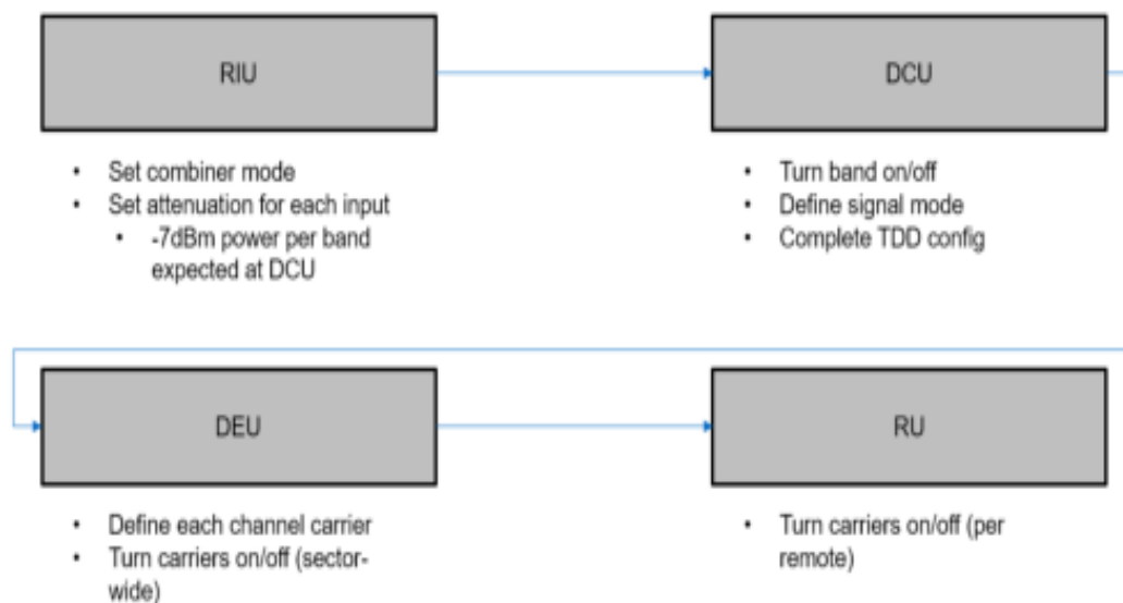
Figure 103. webGUI Workflow
