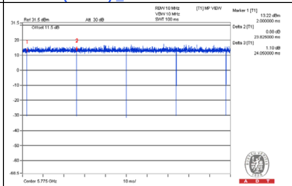
802.11ac (VHT80)_2TX
