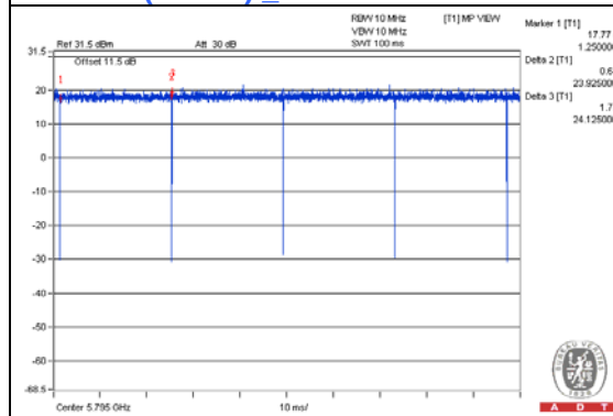
802.11ac (VHT40)_2TX
