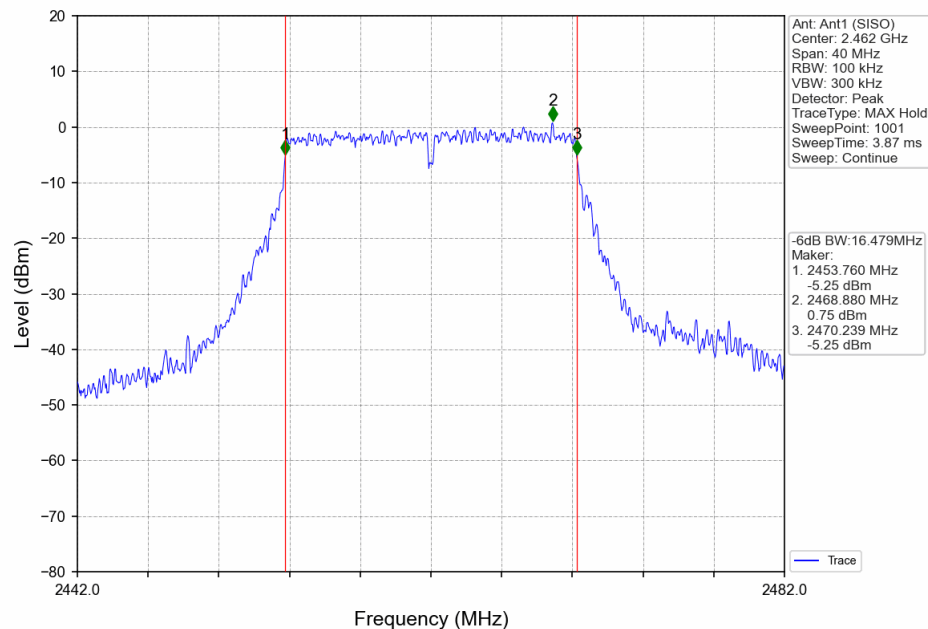
802.11g_HCH_2462MHz_Ant1 (SISO)_NTNV
