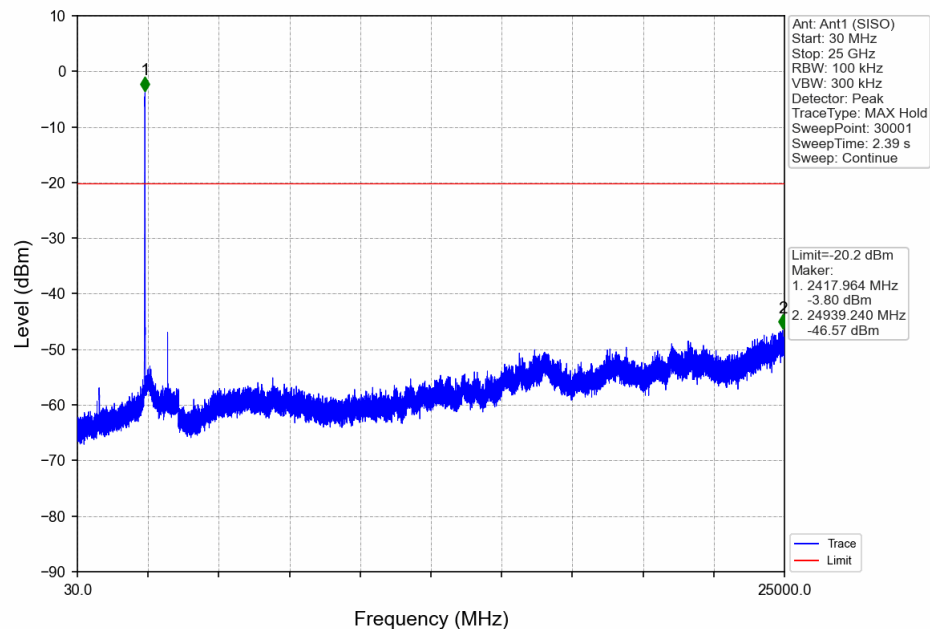
802.11n(HT20)_LCH_2412MHz_Ant1 (SISO)_NTNV
