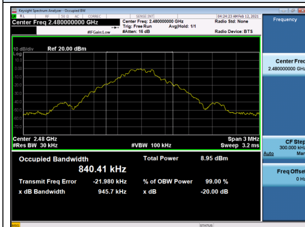
BDR (GFSK) : 20dB BW / OBW (CH78)
