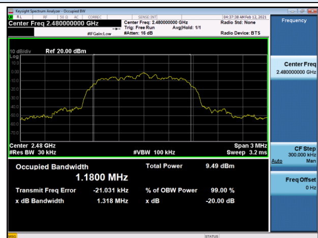
EDR ( \pi/4 -DQPSK) : 20dB BW / OBW (CH78)
