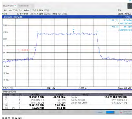
1-N78-3450-3550--30-20-H-9-CP-256QAM-Outer_Fu II-51@0-Ant0-18.223-19.760-≤20-PASS
