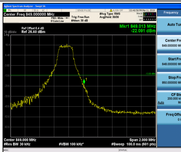
Band5_3MHz_16QAM_20635_1RB#14
