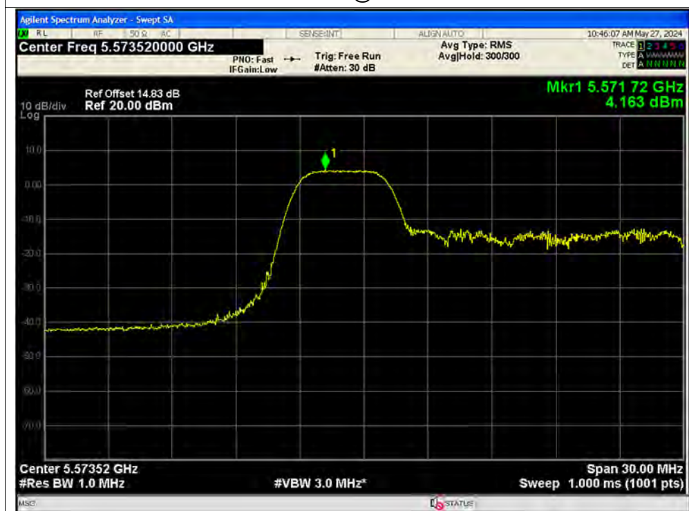
PSD NVNT ax20 52@37 5580MHz Ant1
