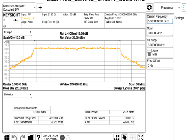
802.11be_20MHz_Chain1_5300MHz
