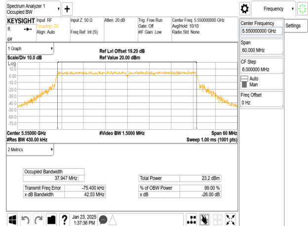
802.11be_40MHz_Chain1_5550MHz
