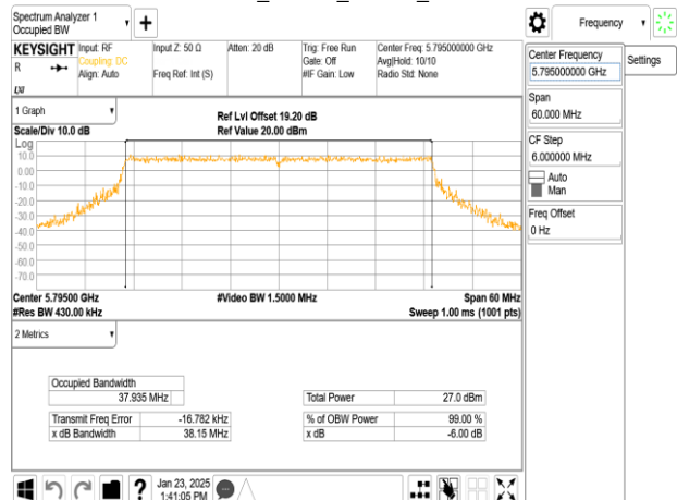
802.11be_40MHz_Chain0_5795MHz
