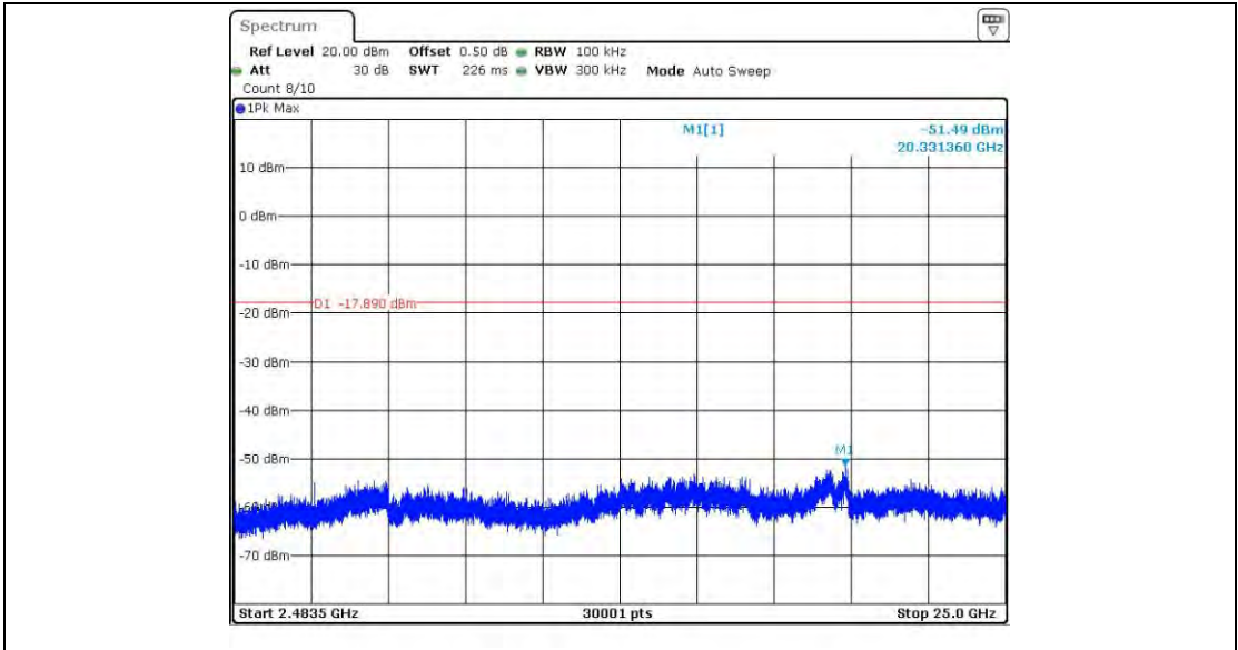
11B_Ant2_2412_2483.5~25000
