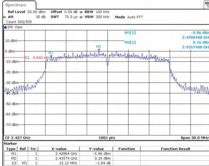
11N20MIMO_Ant2_2437
