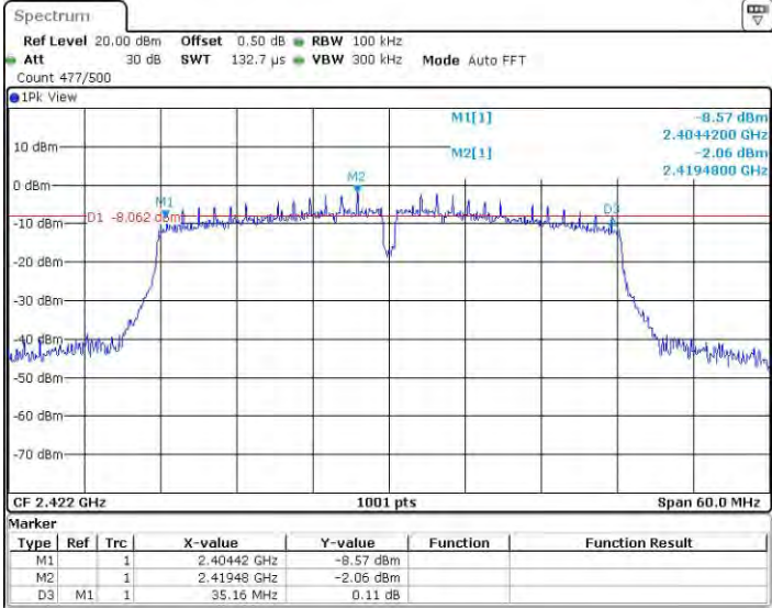
11N40_Ant1_2422
