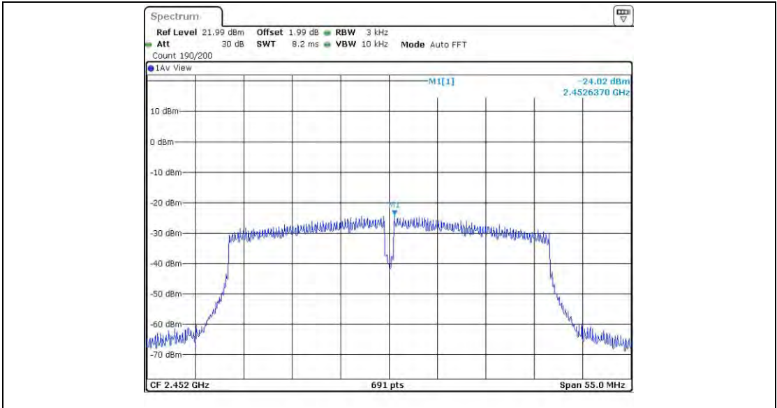
11N40_Ant1_2452
