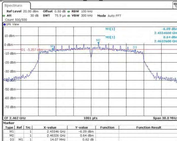
11N20_Ant2_2462
