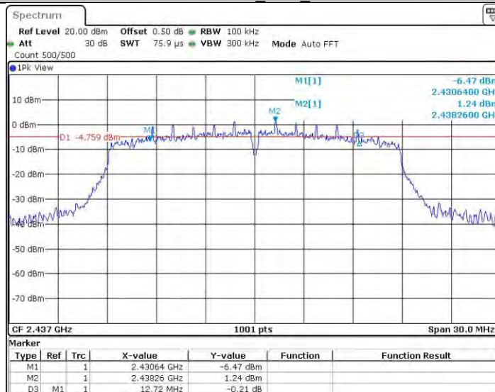
11N20MIMO_Ant1_2437
