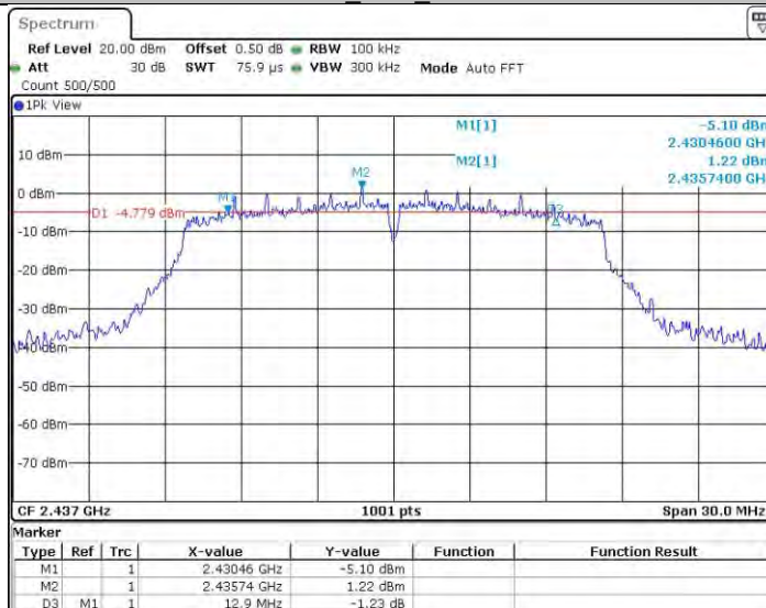
11G_Ant1_2437
