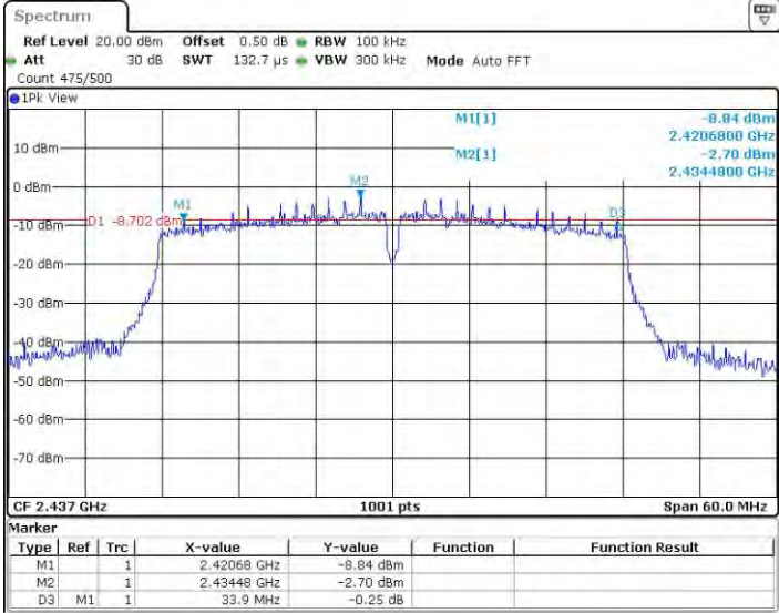
11N40_Ant2_2437
