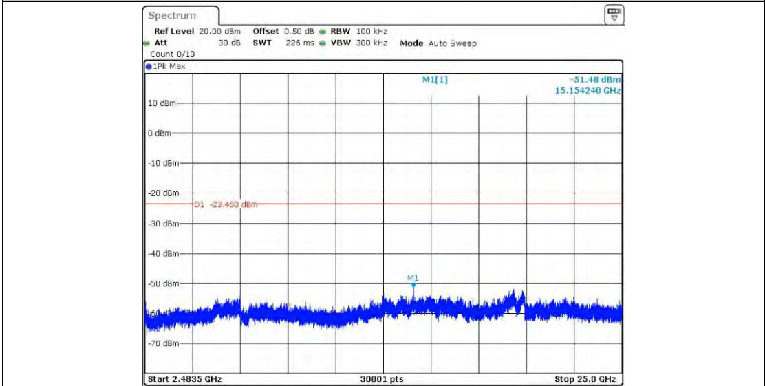
11N40_Ant2_2422_1~2400
