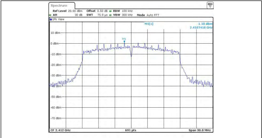
11B_Ant1_2412_0~Reference
