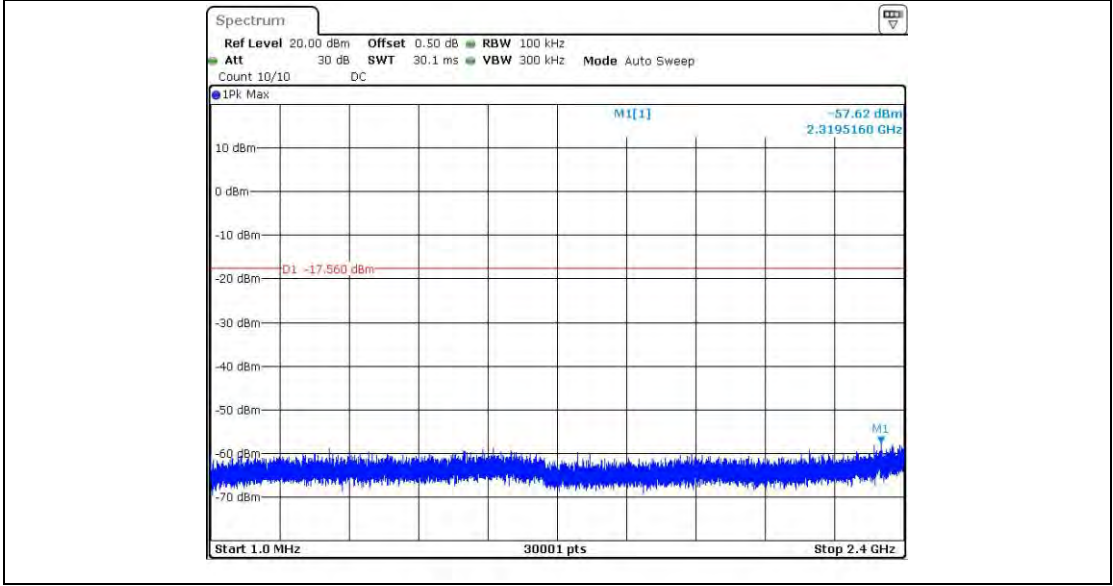
11B_Ant1_2437_0~Reference
