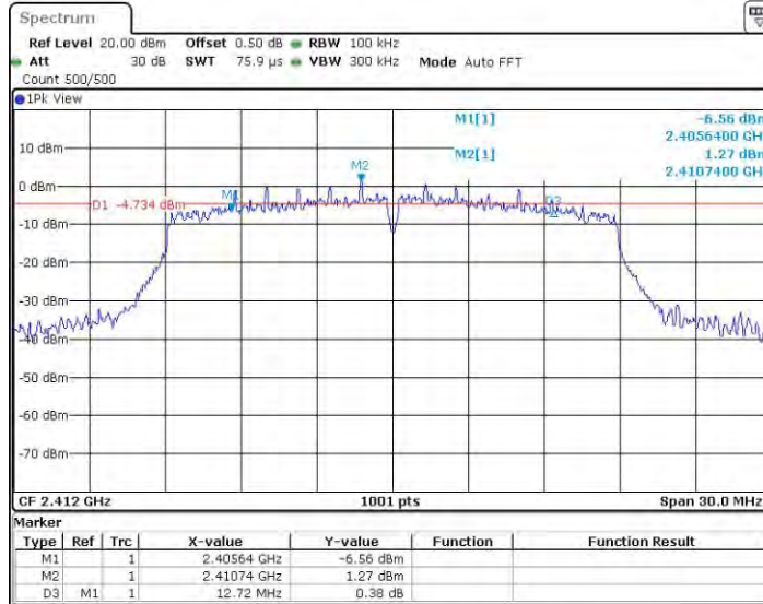
11N20MIMO_Ant1_2412
