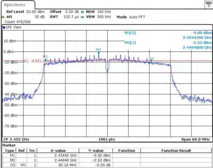
11N40_Ant2_2452
