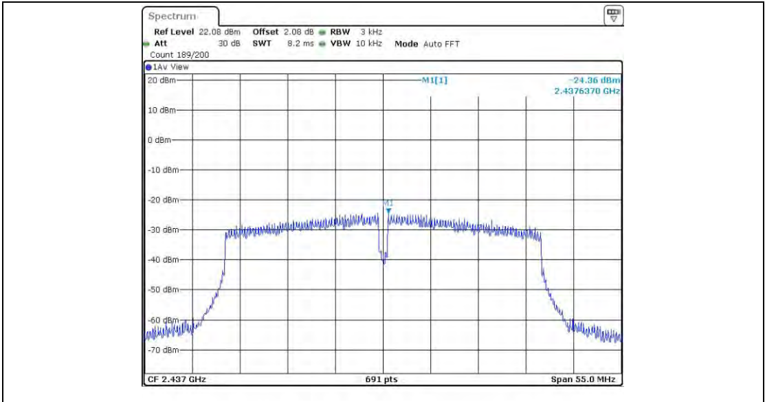
11N4OMIMO_Ant1_2437
