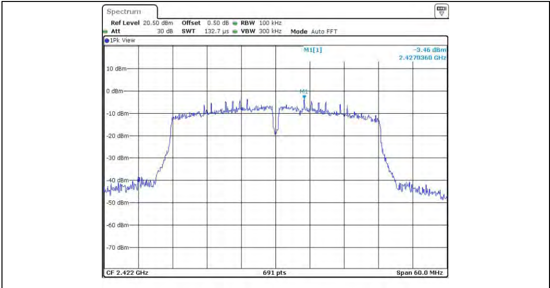
11N40_Ant2_2422_0~Reference
