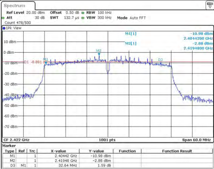
11N40_Ant2_2422
