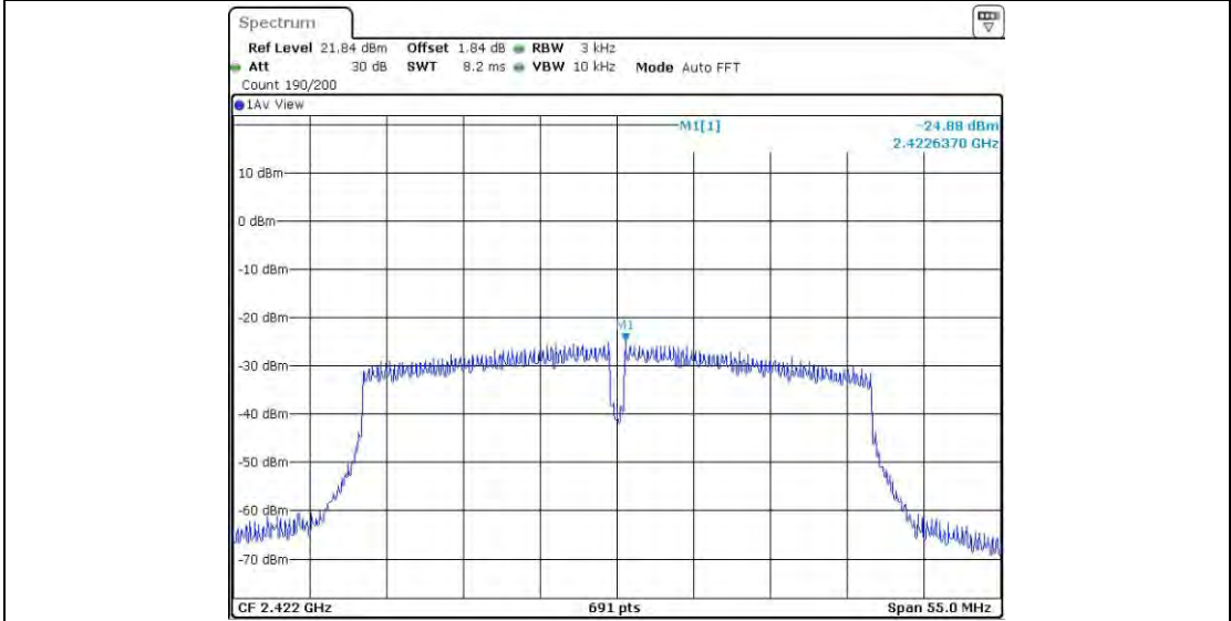
11N40_Ant1_2422
