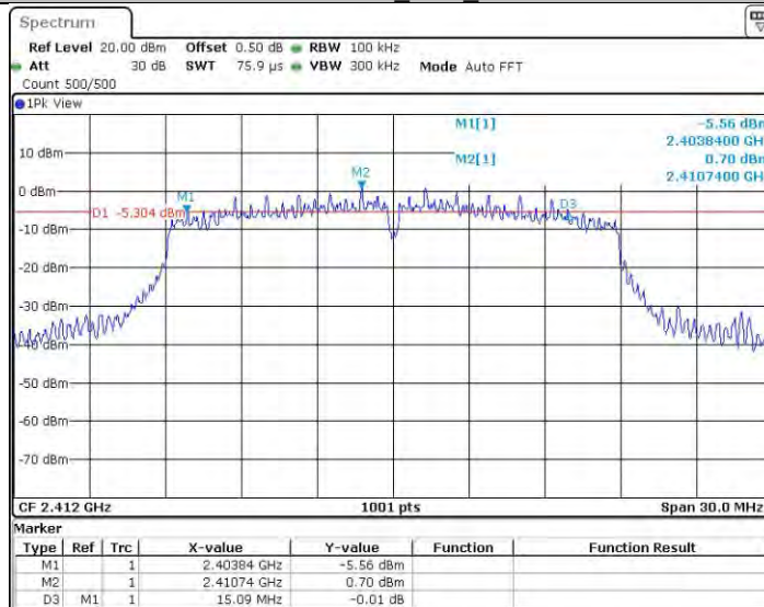
11N20MIMO_Ant2_2412
