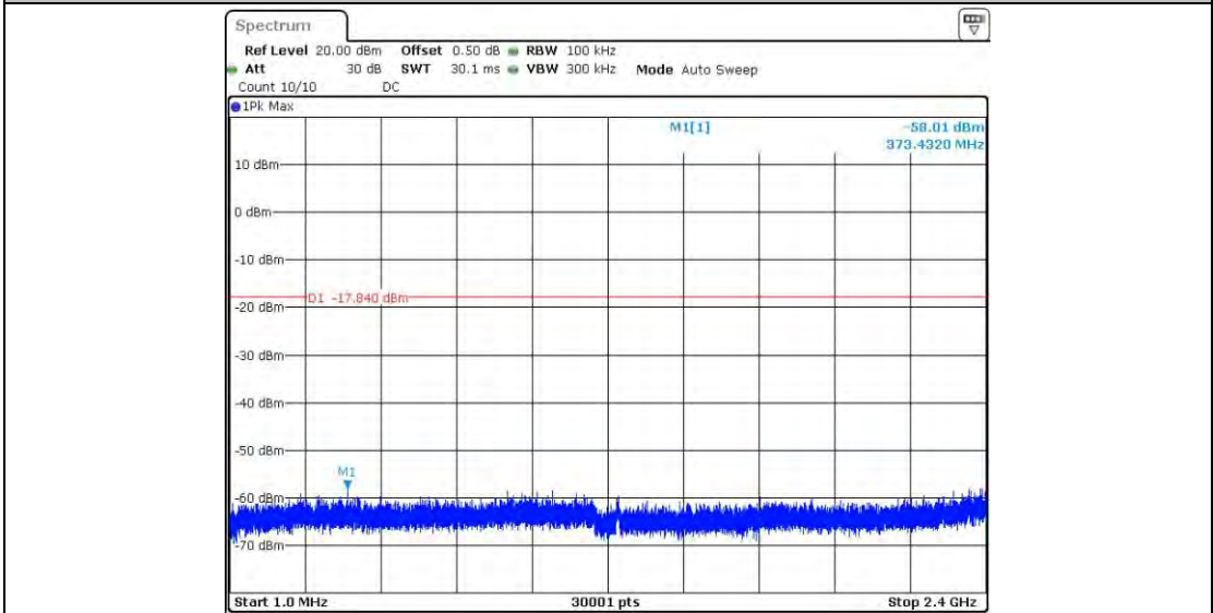
11B_Ant2_2462_0~Reference
