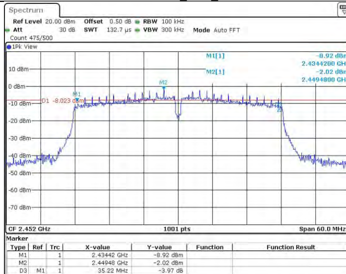
11N4OMIMO_Ant1_2452
