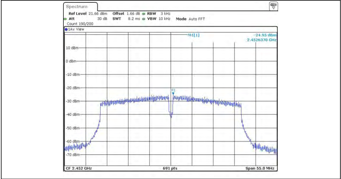
11N40_Ant2_2452
