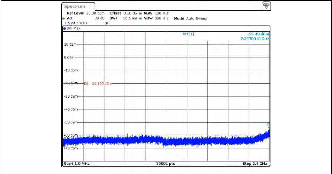
11N20MIMO_Ant1_2462_1~2400
