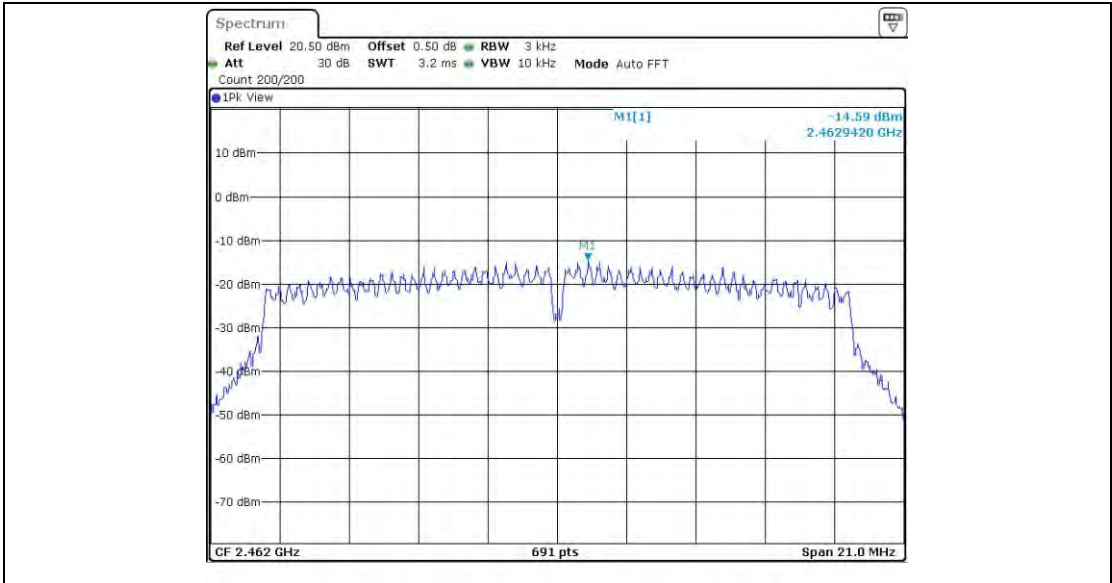
11N20_Ant2_2462
