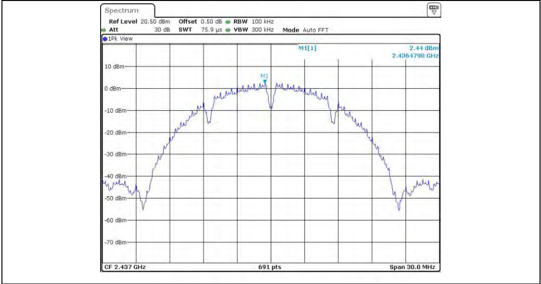
11B_Ant1_2437_0~Reference
