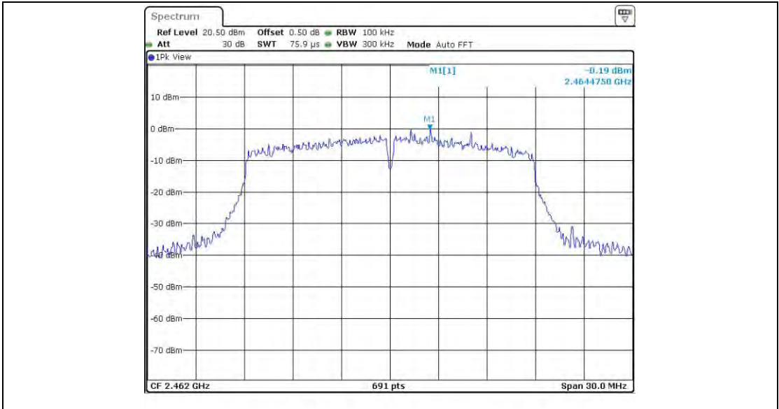
11N20MIMO_Ant1_2462_0~Reference
