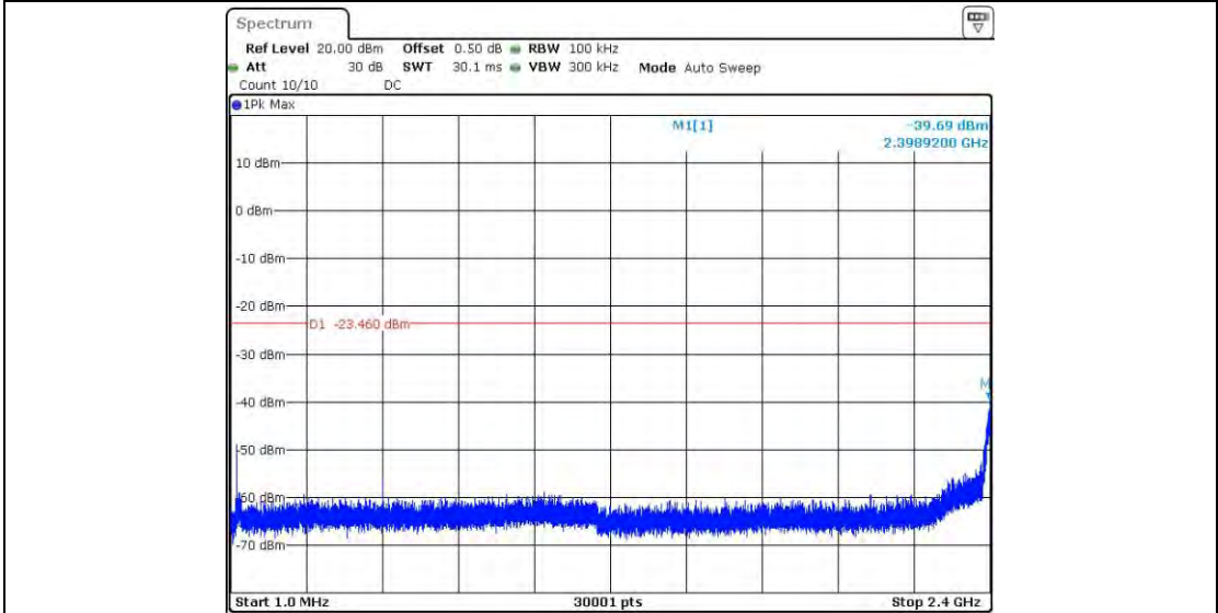
11N40_Ant2_2422_0~Reference
