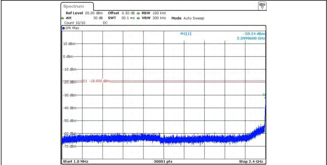
11B_Ant1_2412_1~2400
