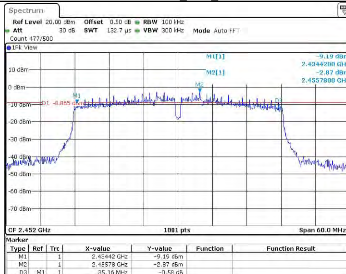
11N4OMIMO_Ant2_2452
