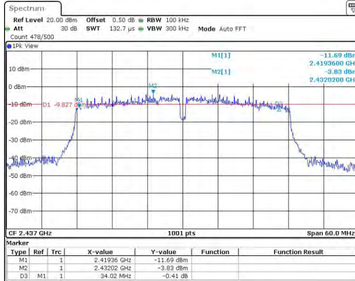
11N4OMIMO_Ant2_2437
