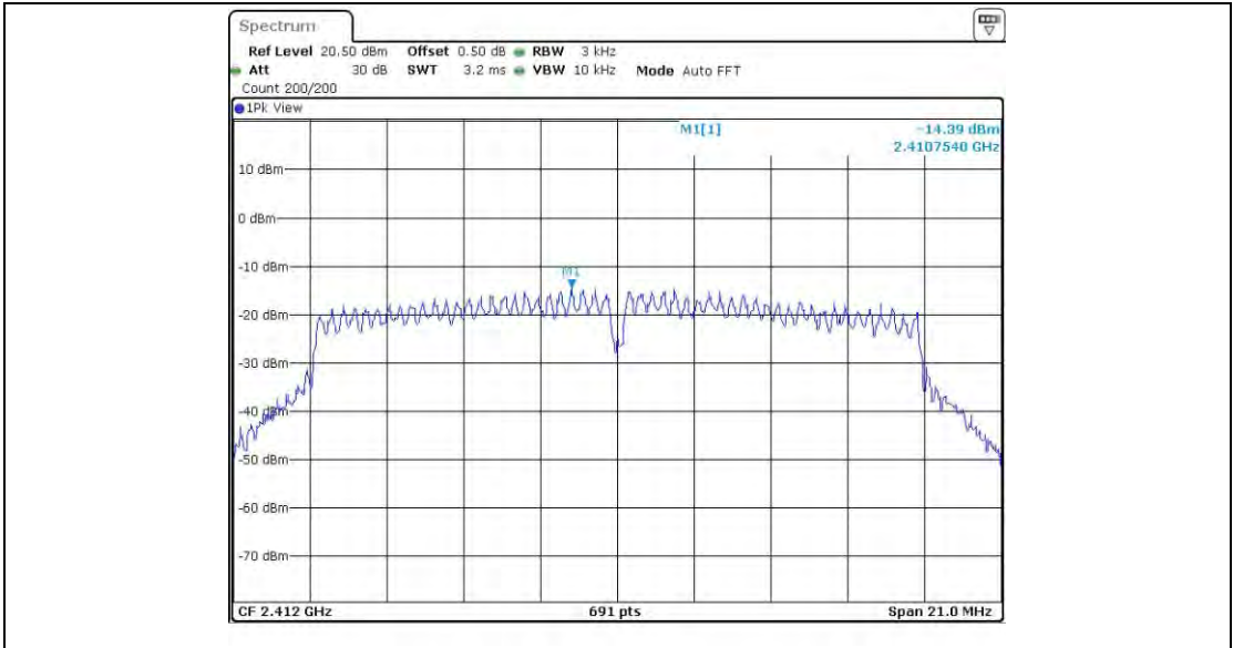
11G_Ant2_2412
