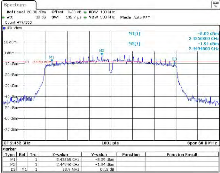
11N40_Ant1_2452
