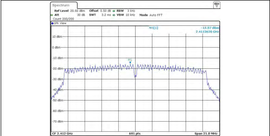
11N20_Ant1_2412
