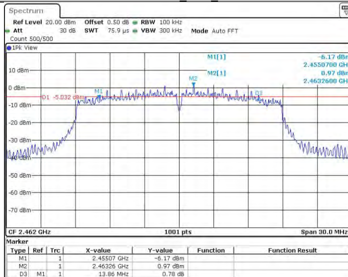
11N20MIMO_Ant2_2462
