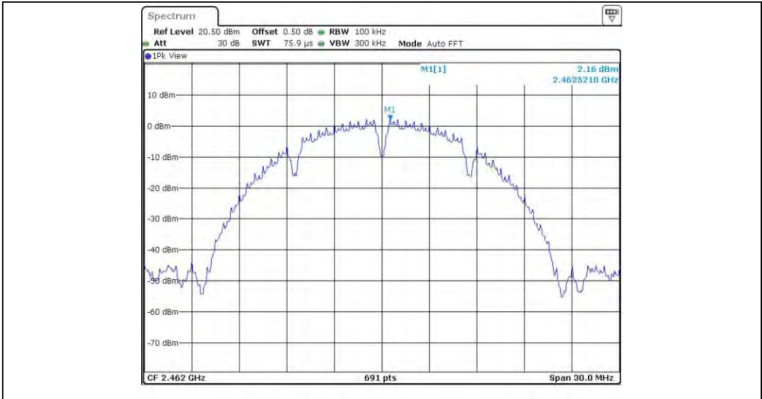
11B_Ant2_2462_0~Reference
