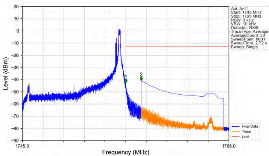
Band4 10MHz QPSK HCH 1750MHz RB 1 49 NTN
