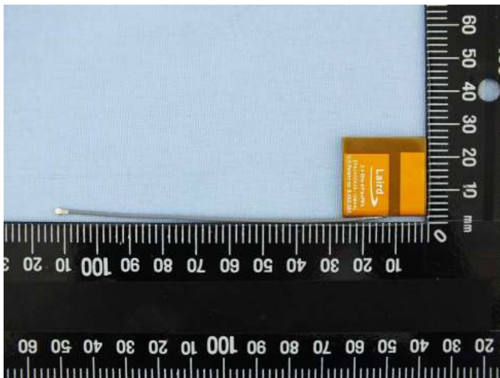
Antenna: mFlexPIFA
