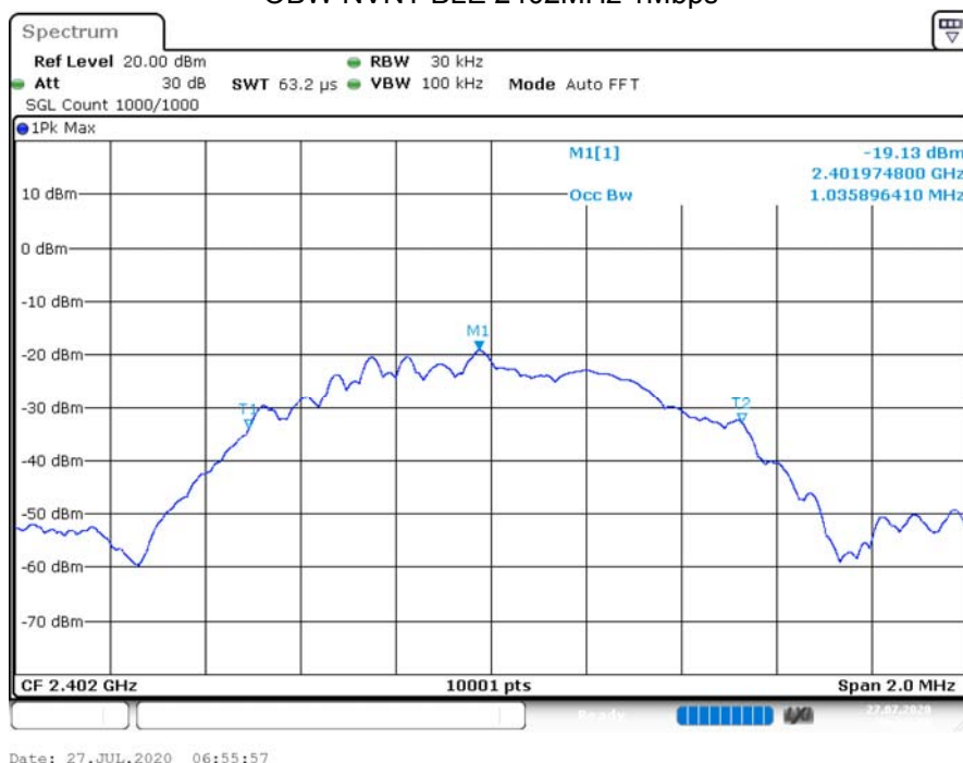
OBW NVNT BLE 2402MHz 1Mbps
