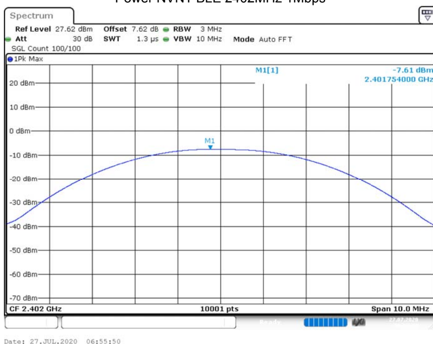
Power NVNT BLE 2402MHz 1Mbps
