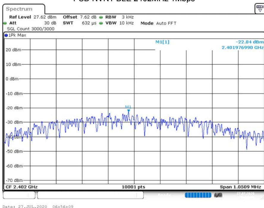
PSD NVNT BLE 2402MHz 1Mbps
