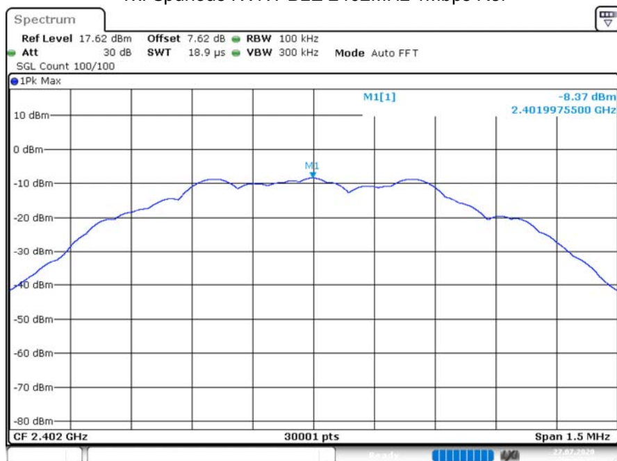
Tx. Spurious NVNT BLE 2402MHz 1Mbps Ref
