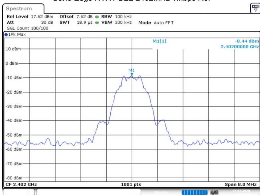
Band Edge NVNT BLE 2402MHz 1Mbps Ref
