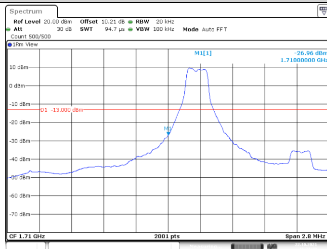
Band66-1.4MHz-QPSK-131979-1-0-Low--26.96-PASS
