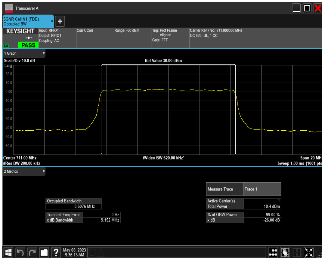
n12 SCS=30kHz CP_QPSK BW=10MHz Channel=142200 RB=24@0
