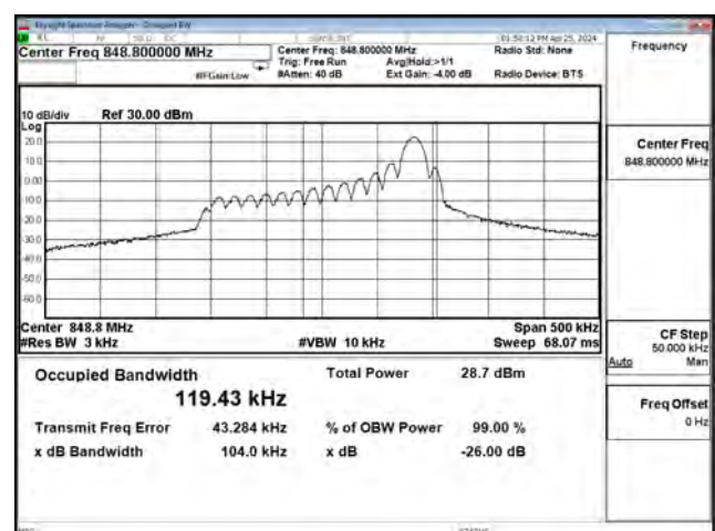
QPSK_CH27038_15k_1RB11
