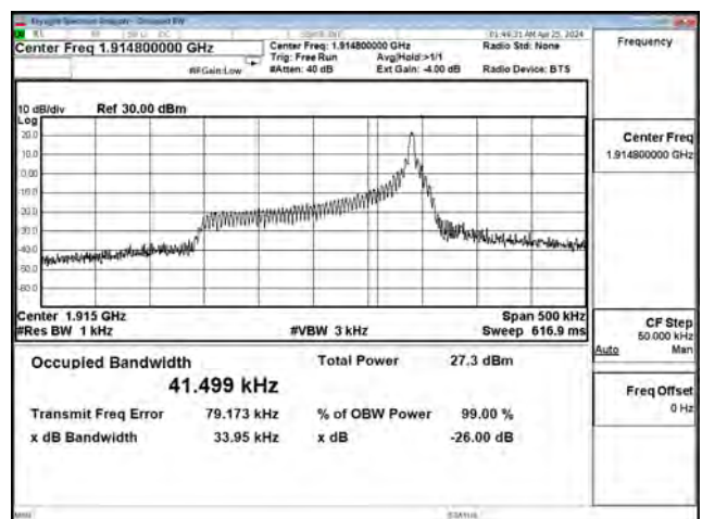
QPSK_CH26688_3.75k_1RB47
