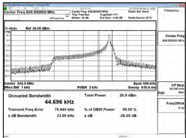
QPSK_CH27038_3.75k_1RB47
