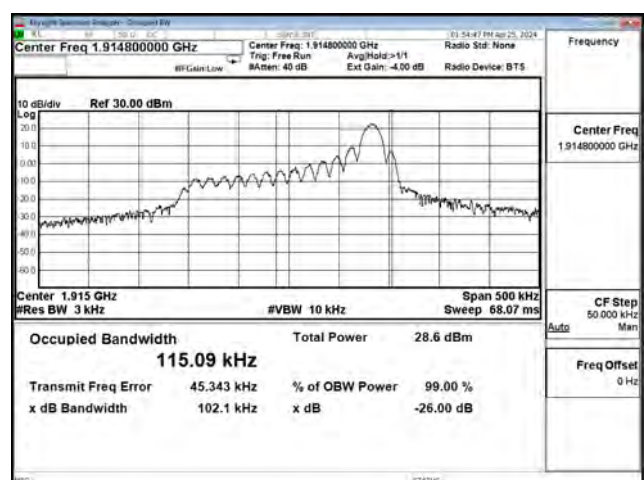
QPSK_CH26688_15k_1RB11
