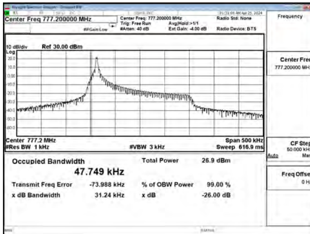
BPSK_CH23278_3.75k_1RB47
