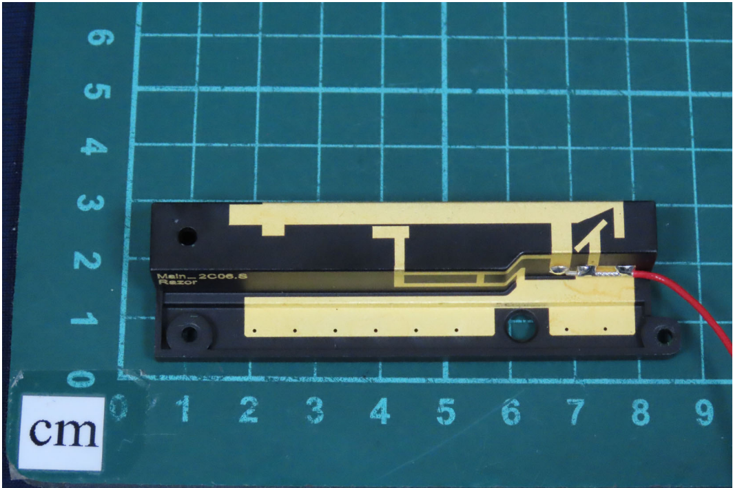
(37) EUT Photo_LTE Antenna
