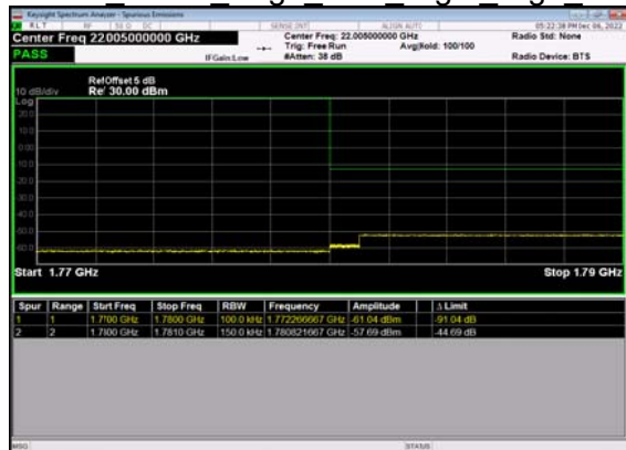
N66(15M)_DFT-s- OFDM BPSK Edge 1RB Right High CH
