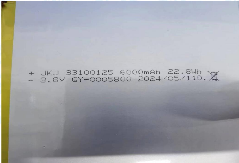
Photo 11 Battery parameter
