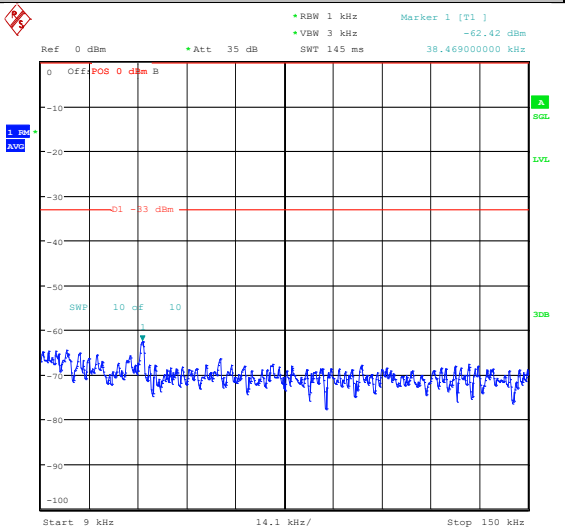
Band26(824-849)-3MHz-QPSK-26805-1RB#0-100 0~3000-PASS
